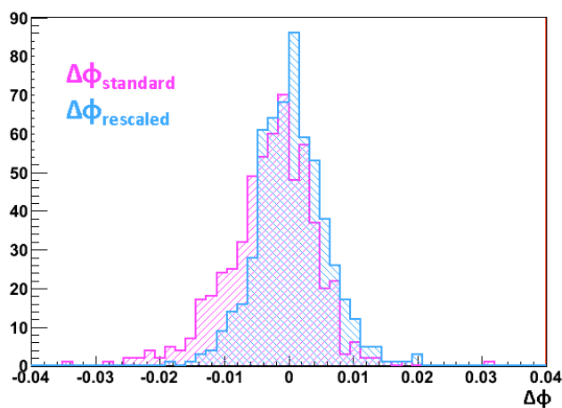
Figure 5.21 – Distribution \Delta\varphi_{rescaled} et \Delta\varphi_{standard} pour les électrons medium identifiés comme issus de la désintégration de Z dans les données à 7 TeV
