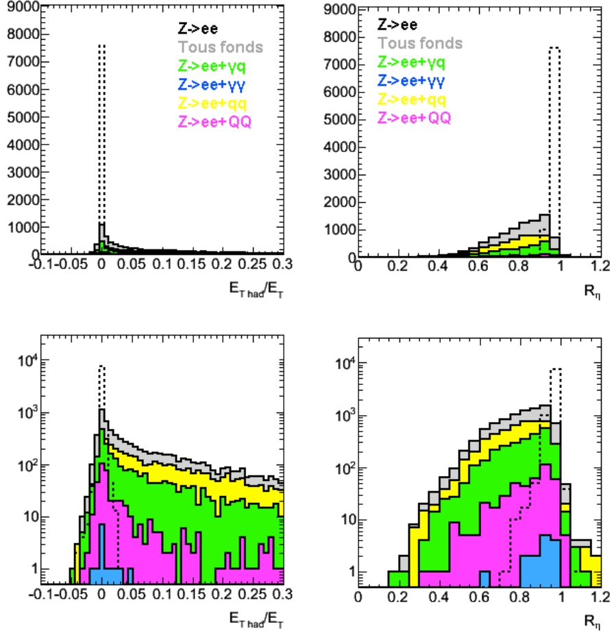
Figure 6.24 – Distribution de R_{had} et R_{\eta} pour les différents types d'électrons sélectionnés par la reconstruction des évènements Z \rightarrow ee + xx , avec x = \gamma, q et Q . En haut les distributions sont données en échelle linéaire et en bas en échelle logarithmique.
