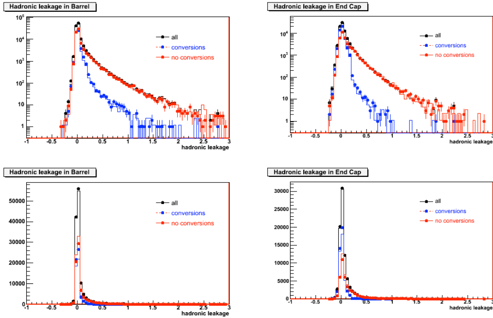
Figure 5.3 – Distributions de leakage hadronique pour les premières données à 7 TeV (points) et le Monte Carlo de biais minimum à 7 TeV (lignes continues). A gauche dans le tonneau et droite dans les bouchons, logarithmique en haut, linéaire en bas
