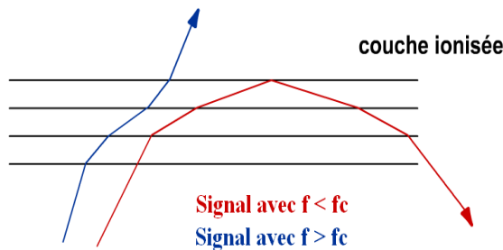
Figure I.3 Fréquence critique des couches ionosphériques
