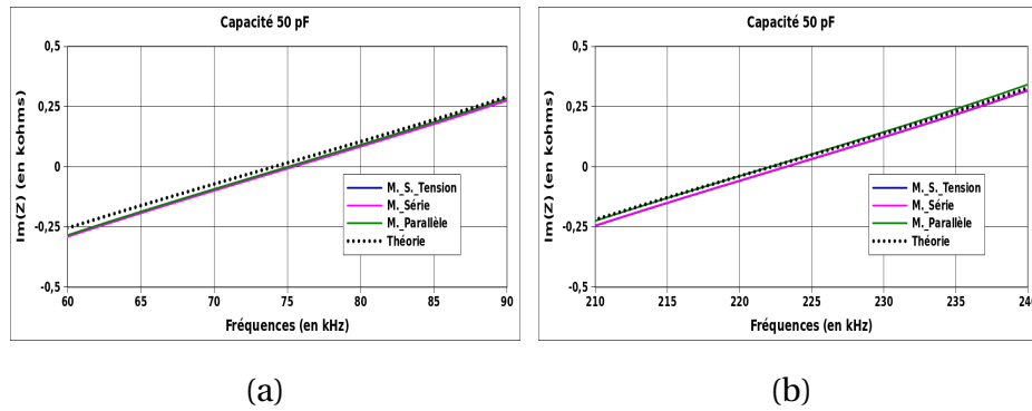
Figure III.19 : Partie imaginaire de l'impédance ramenée au niveau du générateur : au voisinage des fréquences f = 75 \text{ kHz} (a) et f = 225 \text{ kHz} (b)
