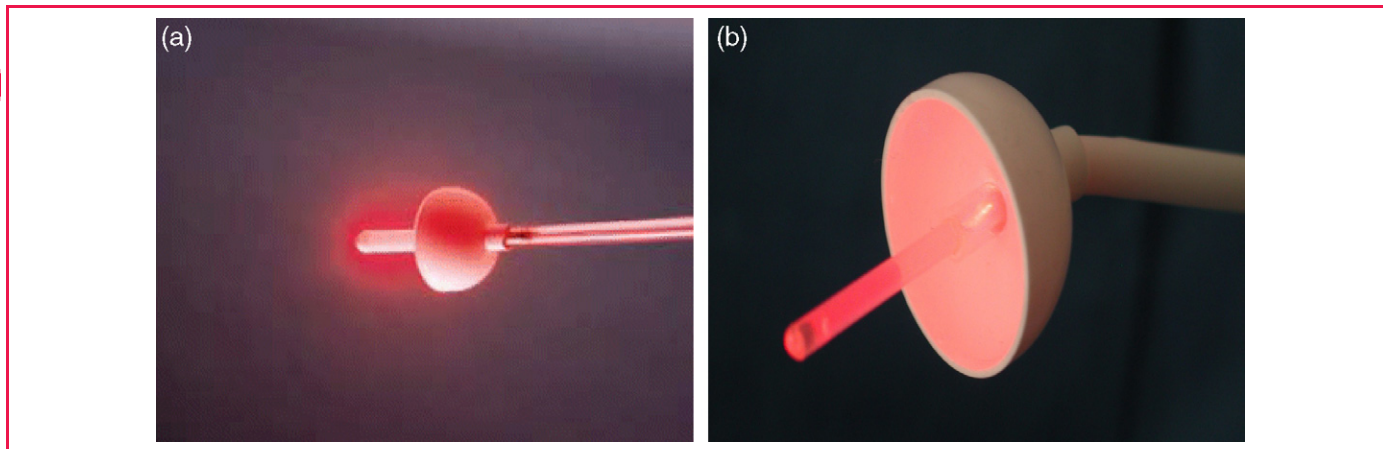
Fig. 7. (a) et (b) Appliqueur de lumière exo- et endocervicale permettant la PDT des dysplasies cervicales ( http://www.biolitec.com ).
