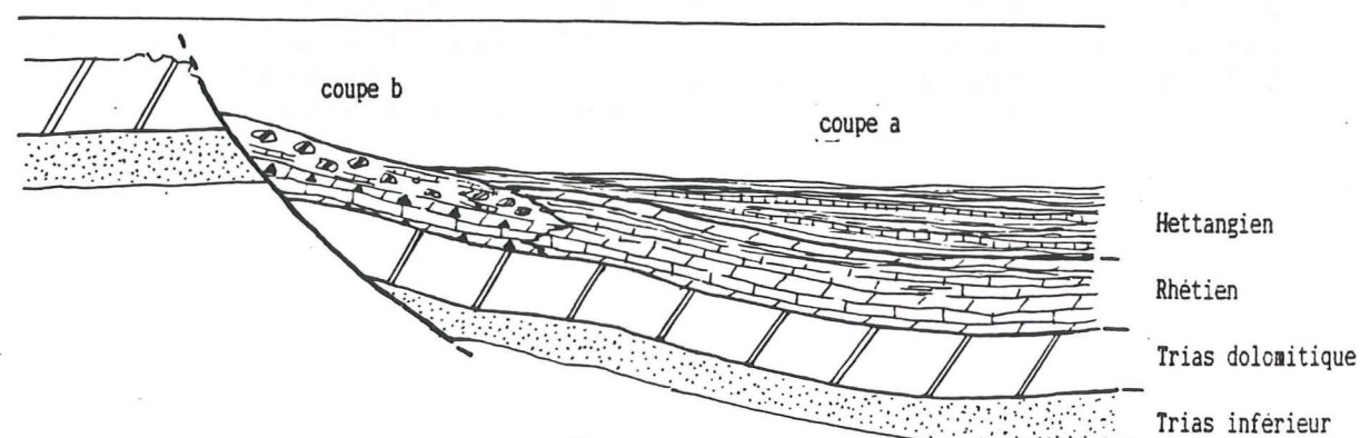
Fig 51: schéma hypothétique de la structuration anté-tectonique du secteur du Coëtet
