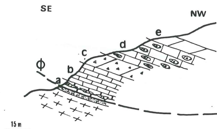
Fig 23: complexe de Chasseforêt, coupe 1
