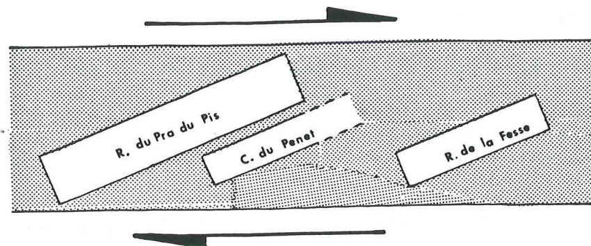
Obliquité des mégaboudins triasiques par rapport à la direction d'alignement = déformation non coaxiale.
