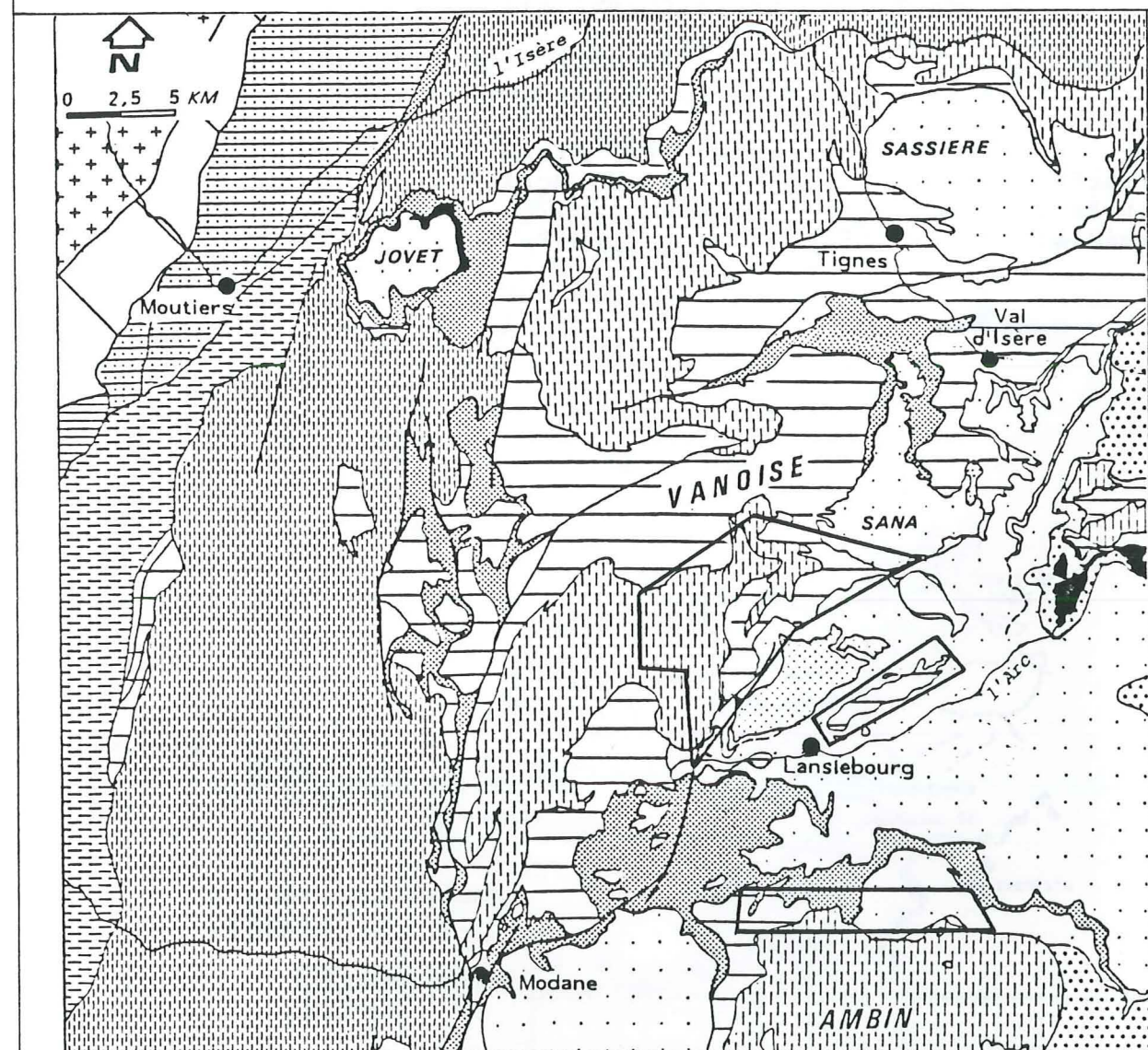
Fig 2 : schéma structural des Alpes occidentales
