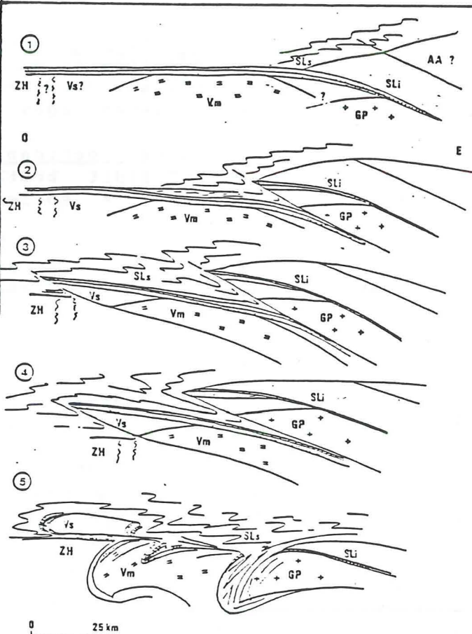
Fig 11 : modèle d'évolution structurale de la chaîne alpine sur la transversale de Vanoise (d'après GOFFE, 1982)
