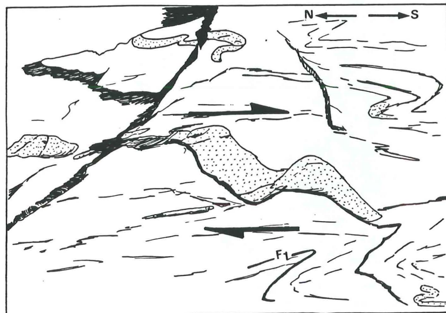
Rotation dextre des boudins de quartz, cisaillement contemporain de D3b.
