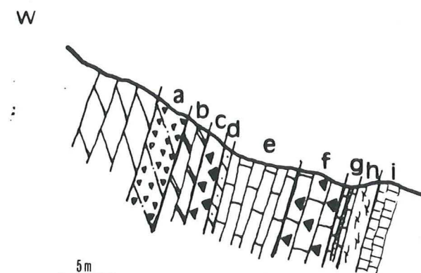
Fig 14: coupe de Bellecombe-Est.
