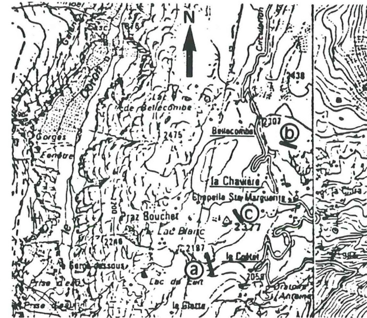
Fig 45 : localisation des coupes du Coëtet et de Chavière (carte topo. au 1/50 000, feuille Modane)
