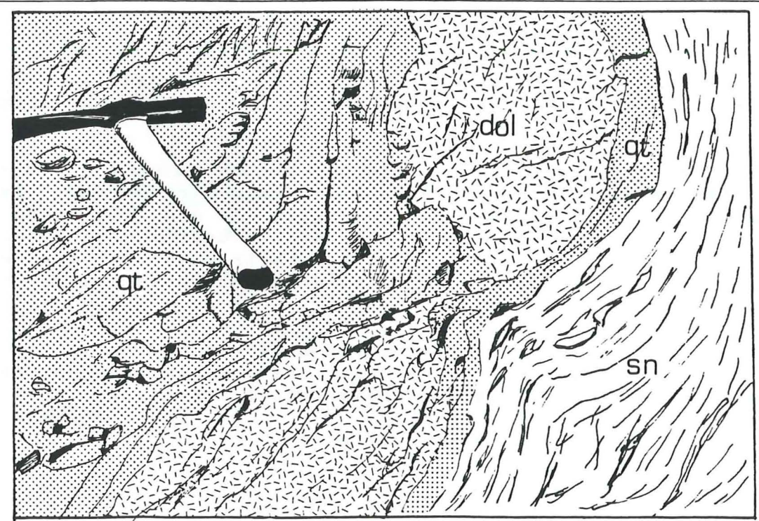
Fig 25: quartzites reconstitués à la base de la série bréchiq. de Chasseforêt. Noter l'intercalation de dolomie bréchiq. boudinée. qt : quartzites à faciès scythien ; dol : dolomie bréchiq. ; sn : schistes noirs (Dogger?)
