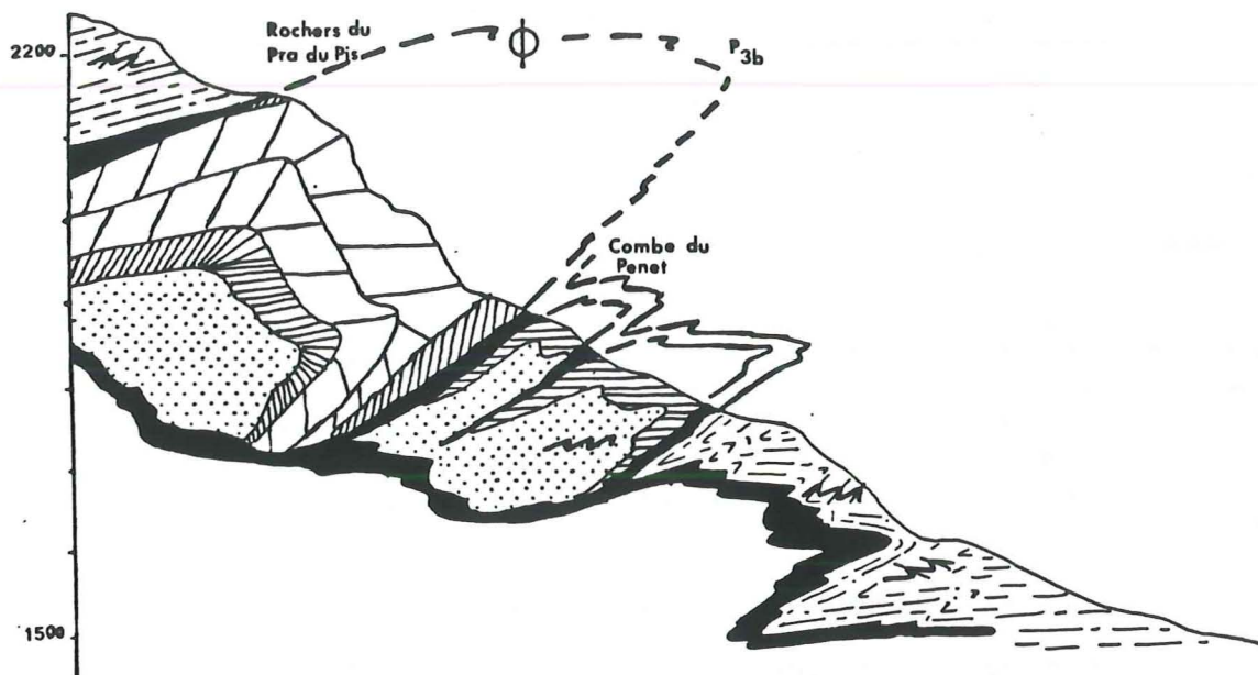
Fig100: coupe géologique simplifiée de la fenêtre de Lanslevillard.
