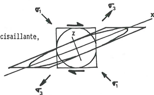
Fig 99: la fenêtre de Lanslevillard, témoin d'un mégaboudinage SW-NE dû au rétrocharriage D3b.
