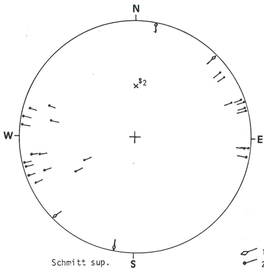
Fig101: orientation des mésostructures de la fenêtre de Lanslevillard
