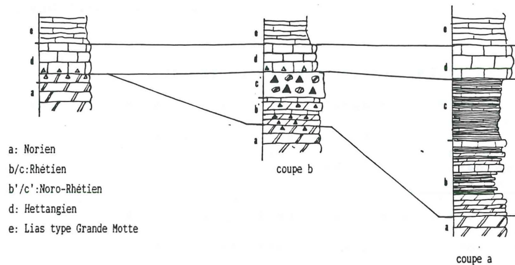
Fig 50: corrélation des coupes a et b après remise de la série à l'endroit
