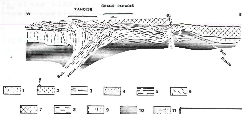
Fig 10: les Alpes occidentales au Crétacé supérieur (d'après CABY et al., 1978).
