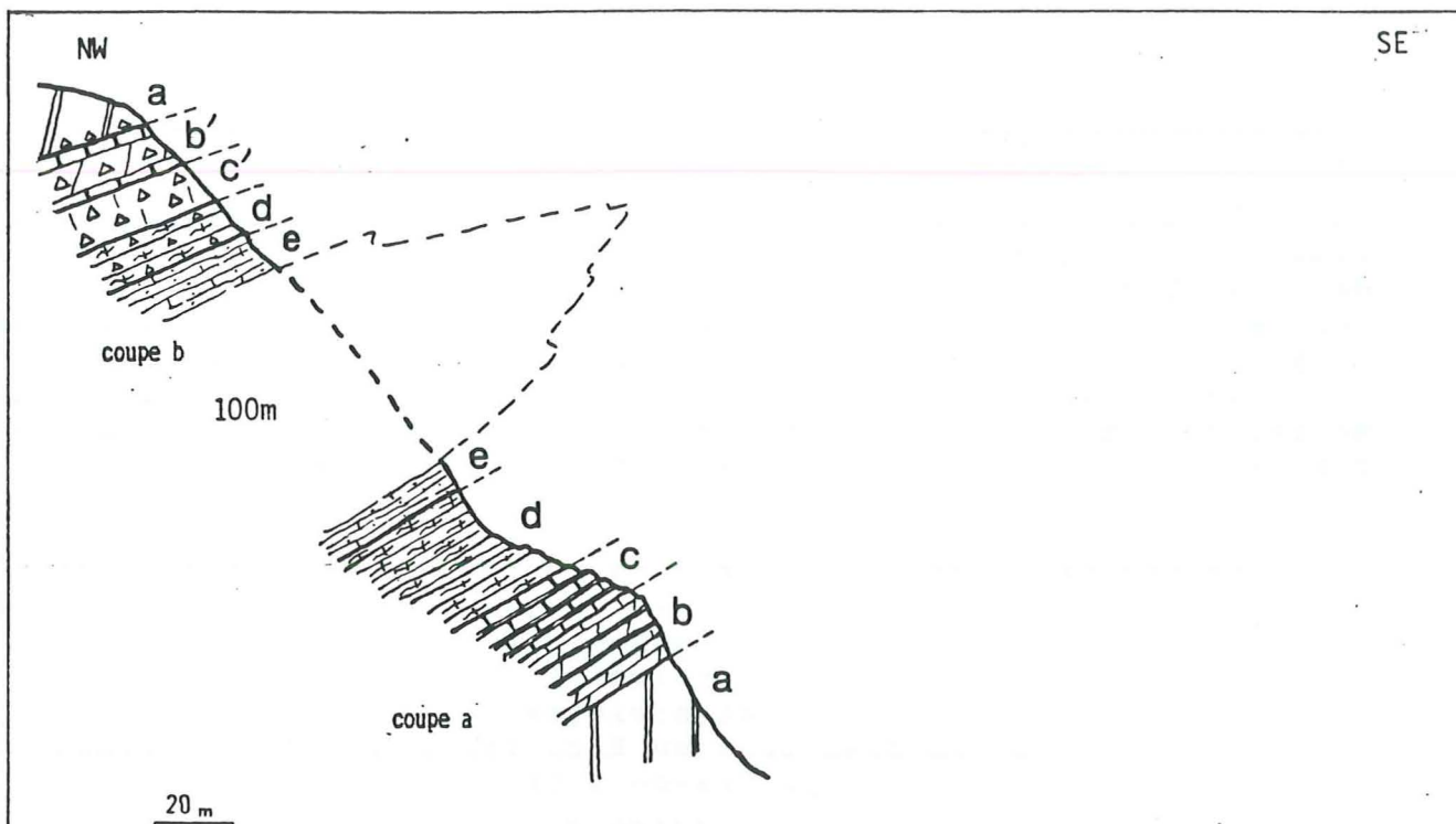
Fig 49: coupe du secteur du Coëtet
