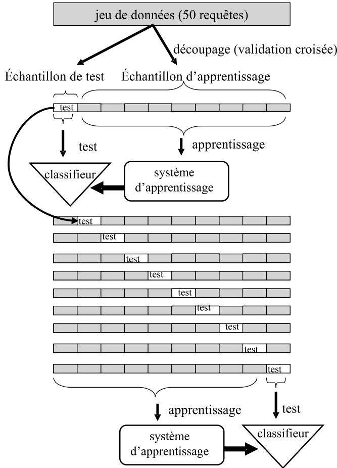
FIG. 4.4 – Illustration de la méthode de la validation croisée pour le découpage des données utilisées pour l'apprentissage et le test du classifieur
