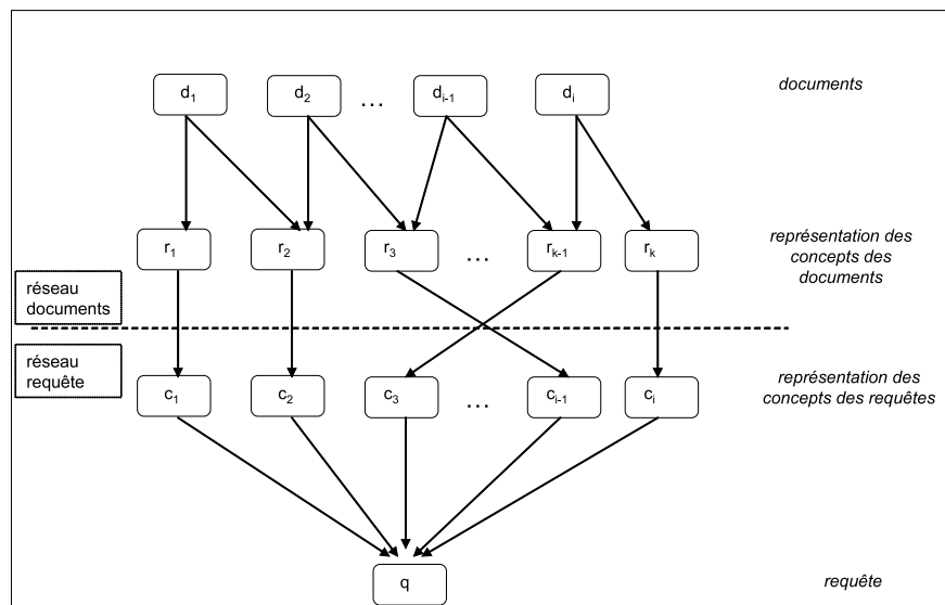
FIG. 1.5 – Exemple de réseau d'inférence pour la RI (Turtle et Croft, 1991)
