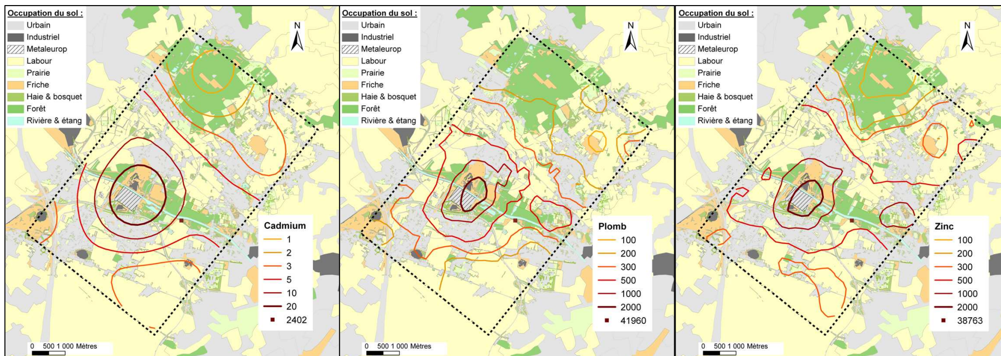
Figure II.6.2. Courbes d'iso-concentration des concentrations totales en Cd, Pb et Zn dans les sols ligneux (mg.kg -1 masse sèche). Le point représenté par un rectangle visualise la localisation et la contamination du point particulier des dépôts de boues de curage. La zone d'étude étendue (8 x 5 km) est figurée par des tirets.
