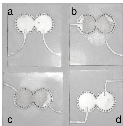
Figure II-12 : photographie des filtres SICC d'ordre 2 avec différents angles d'alimentation
