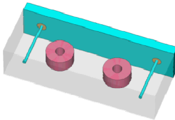
Figure I-17 : dessin d'un filtre d'ordre 2 à résonateurs diélectriques cylindriques
