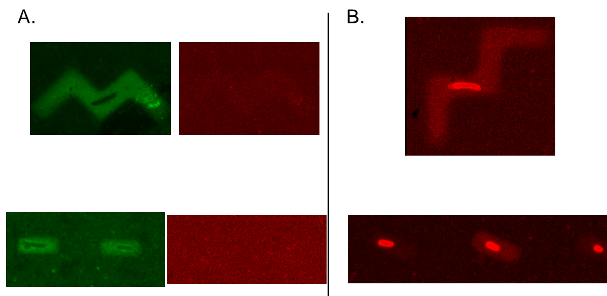
Figure 7. Détection de la viabilité des cellules par coloration. A. Image en fluorescence d' E. coli marquées à l'IP et déposées sur une surface microstructurée d'OTS avec motifs époxyde-streptavidine. B. Image en fluorescence de ce même substrat exposé à l'air et placé sur une plaque chauffante à 180°C.
