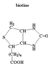
Figure 3. Structure chimique d'une molécule de biotine.
