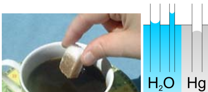
Figure 13. Capillarité. Montée capillaire dans un sucre qui trempe dans une tasse de café (à gauche). L'eau monte le long du tube par capillarité, et à l'inverse, l'air descend dans le tube en repoussant le mercure par capillarité. Plus le tube est fin et plus la montée capillaire est importante (à droite).
