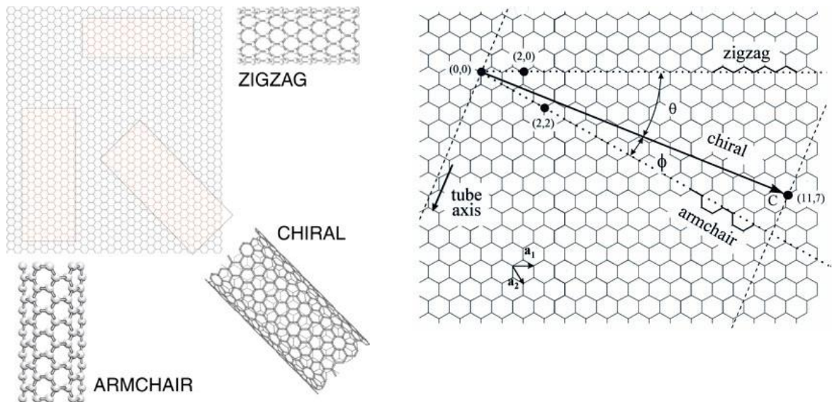
Figure 1 : schéma montrant les différentes structures d'un nanotube monoparoï, et définition des vecteurs a_1 et a_2 .
