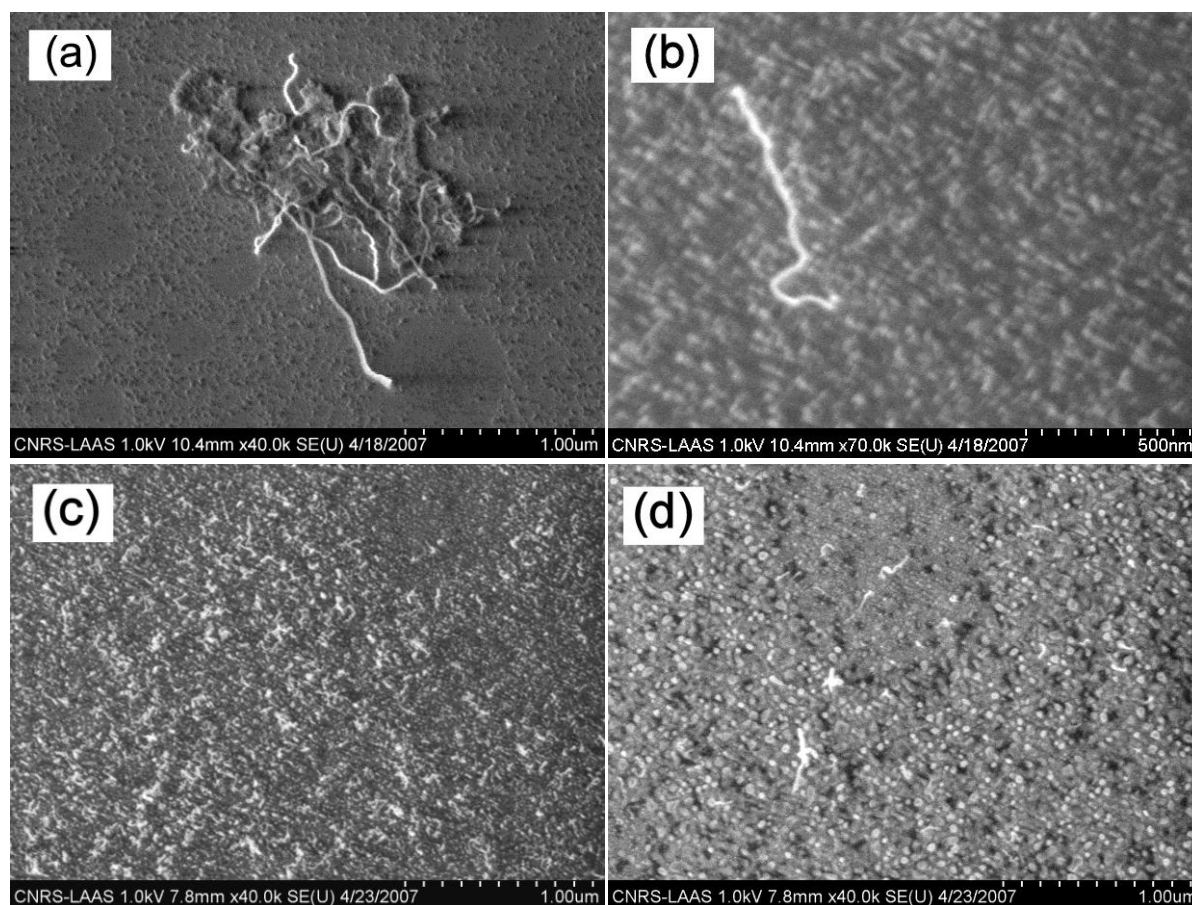
Figure II.9 : Images MEB des échantillons C (a,c) (850°C, 15 min) et D (b,d) (850°C, 45 min).
