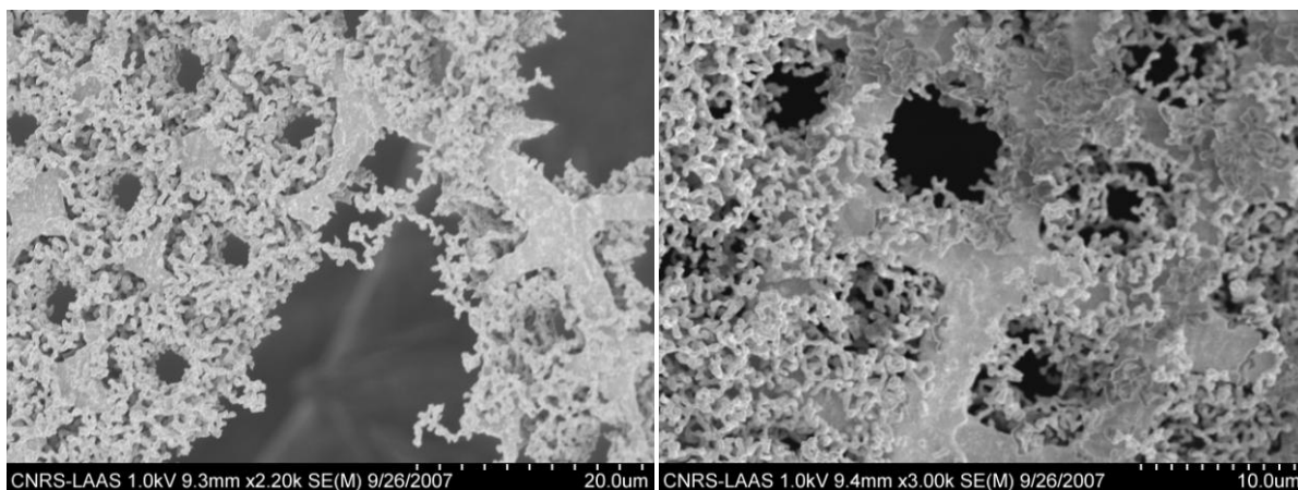
Figure II.13 : Images de MEB de l'échantillon L (850°C, 15min).
