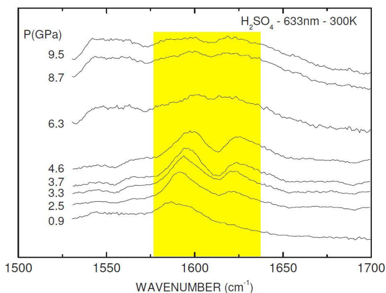
Figure IV.2 : Bande G d'un échantillon de DWNT soumis à différentes pressions jusqu'à 9,5GPa. (milieu transmetteur de pression H_2SO_4 ) [114].
