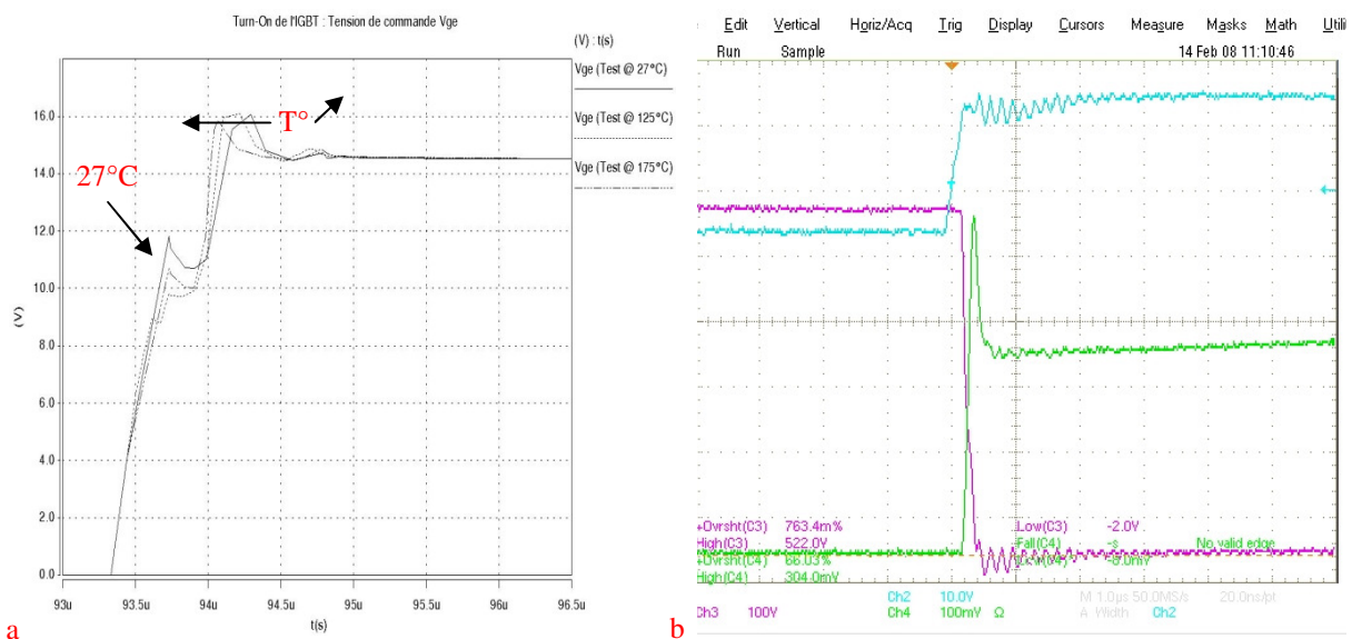
Figure 3.38 : Visualisation des tensions de grille à la mise On de l'IGBT+VT @ (V ge =15V) : a) Simulations ; b) Mesure pour le test à 27°C.
