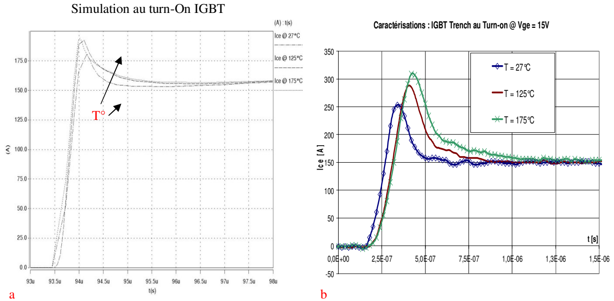
Figure 3.37 : I c au Turn-On de l'IGBT+VT @ (T=27°C, 125°C, 175°C ; V ge =15V) :a) Simulation ; b) Mesures.
