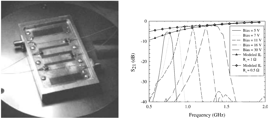
Figure I.29 : Exemple d'utilisation des varactors dans un filtre accordable [44]
