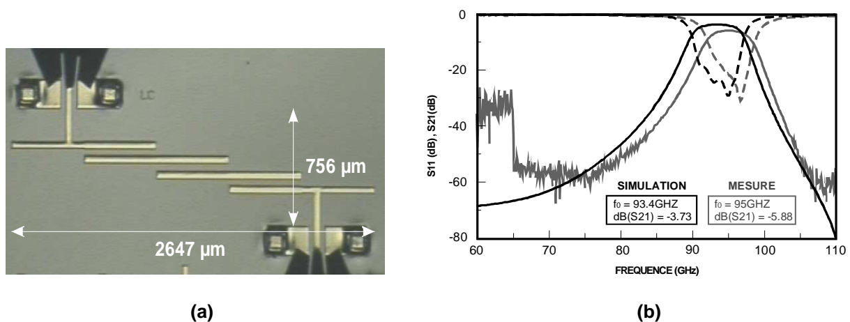
Figure II.50. Filtre à lignes couplées (a) photographie, (b) résultats de simulation HFSS et de mesures
