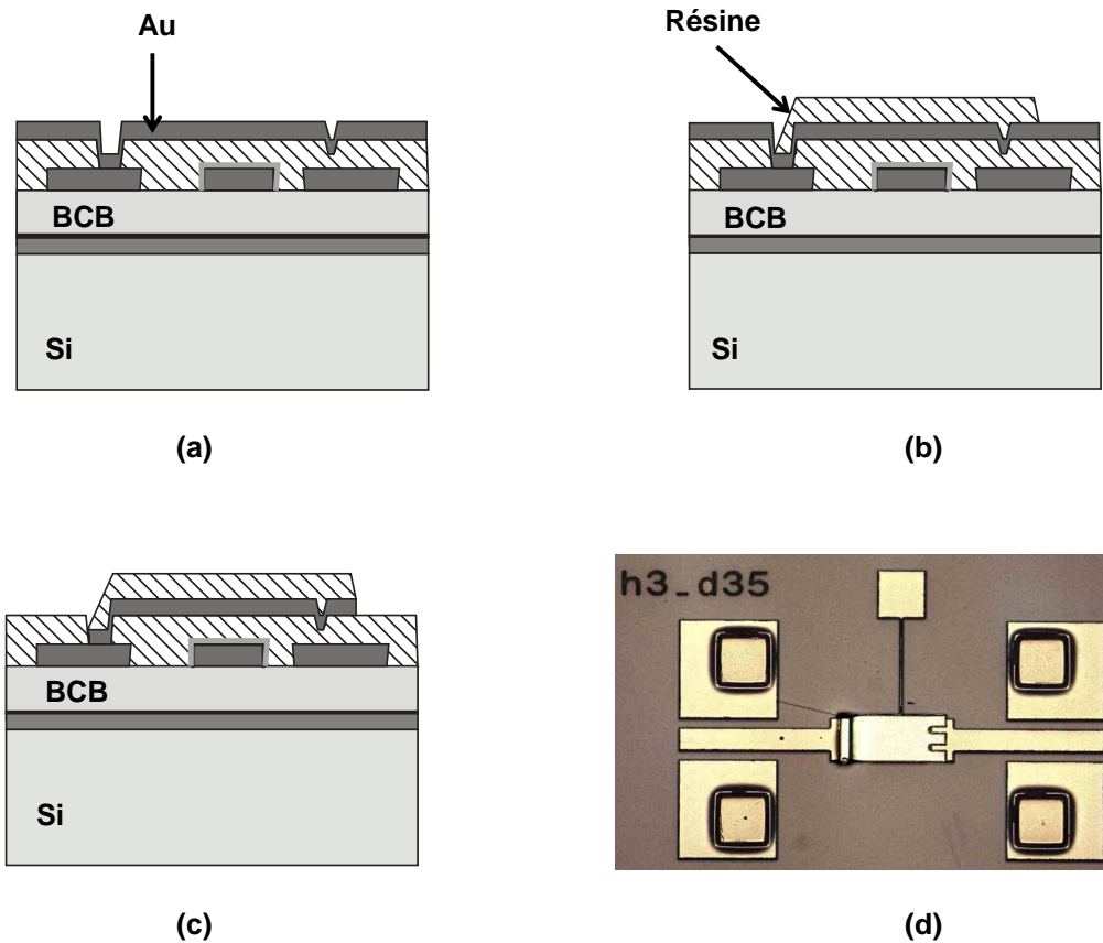
Figure IV.26. Métrallisation de la partie mobile du cantilever
