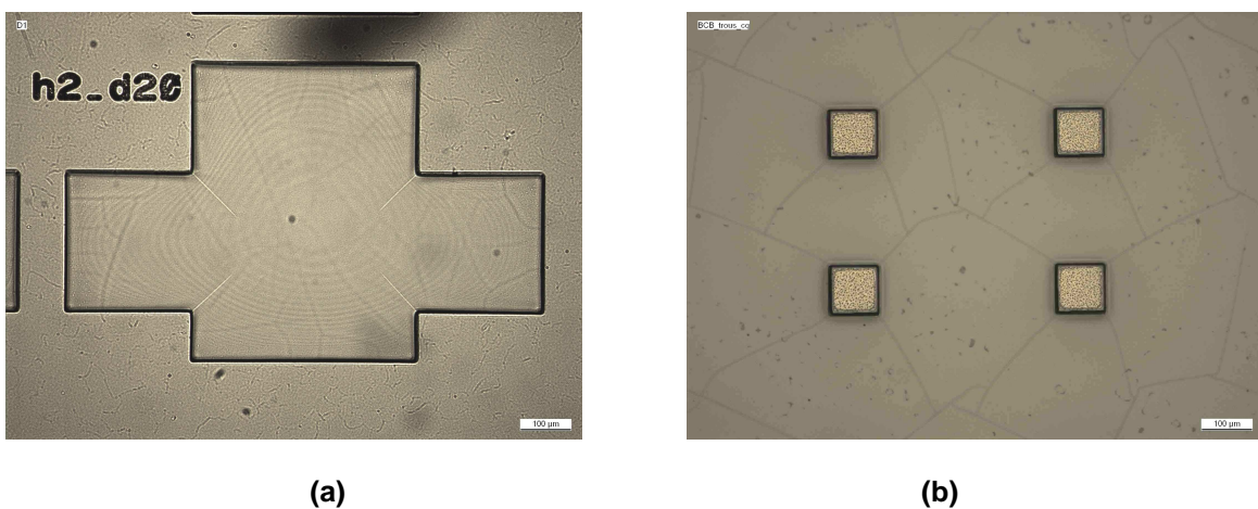
Figure II.36. Photographe des dépôts de 20µm-BCB obtenus
