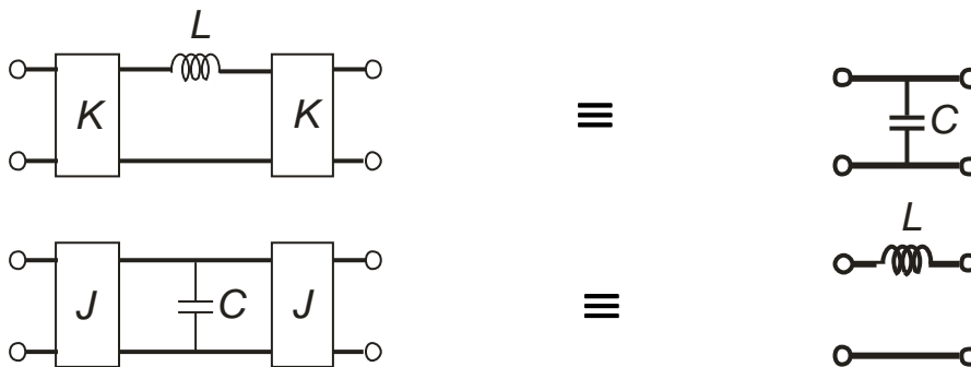
Figure I.8 : Deux des propriétés des inverseurs
