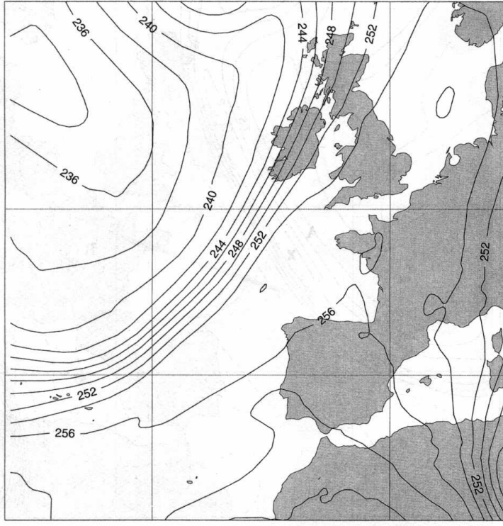
FIG. 1 – Pr vision ARPEGE 6h du champ de temp rature   500 hPa pour le 9 janvier 1988   12H. L' cart entre les isolignes est de 2K.
