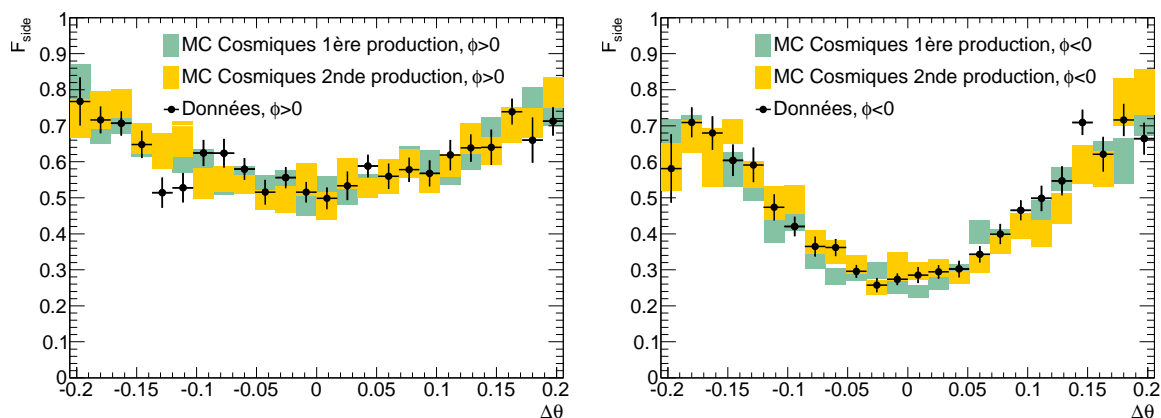
FIG. 4.29 : Profil moyen de la variable F_{side} en fonction de \Delta\theta pour les objets électromagnétiques de la partie haute ( \phi > 0 ) et de la partie basse ( \phi < 0 ) dans les événements cosmiques.
