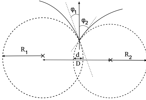
FIG. 3.9 : La proximité des traces issues d'un même vertex est estimée par la distance d d'approche minimale. Sortant d'un vertex de conversion, leur colinéarité est vérifiée : par la différence d'angles \eta et \phi et par la comparaison de la distance D à la somme R_1 + R_2 .
