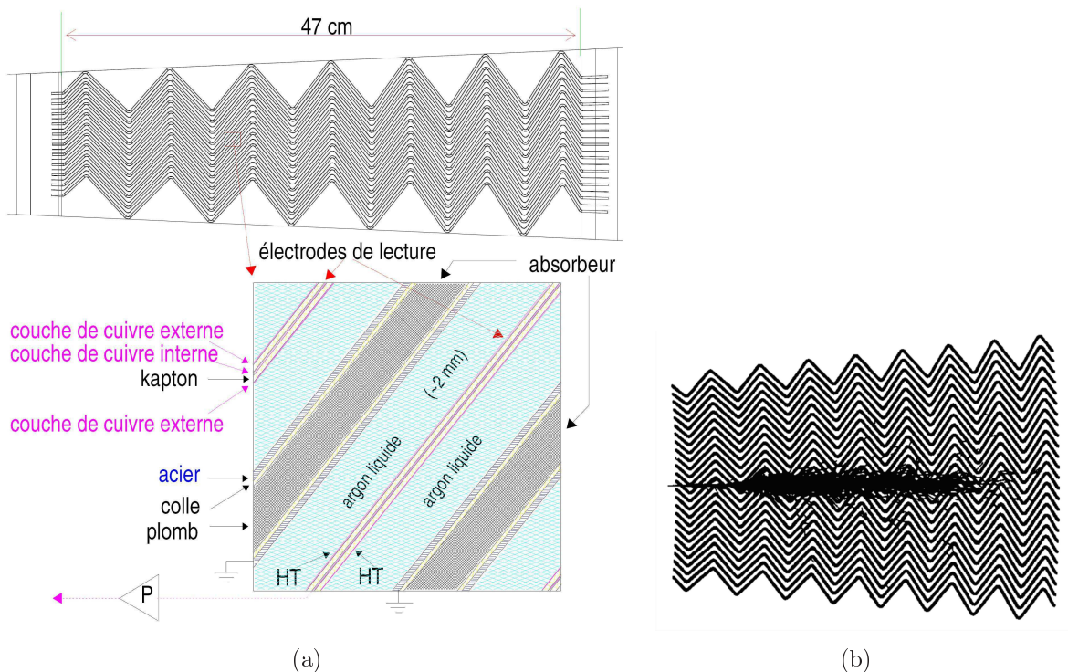
FIG. 2.7 : (a) Structure en accordéon du calorimètre électromagnétique avec l'argon liquide pris en sandwich entre des tranches d'absorbeur. (b) Simulation GEANT4 d'une gerbe électromagnétique se développant dans une partie du calorimètre électromagnétique.
