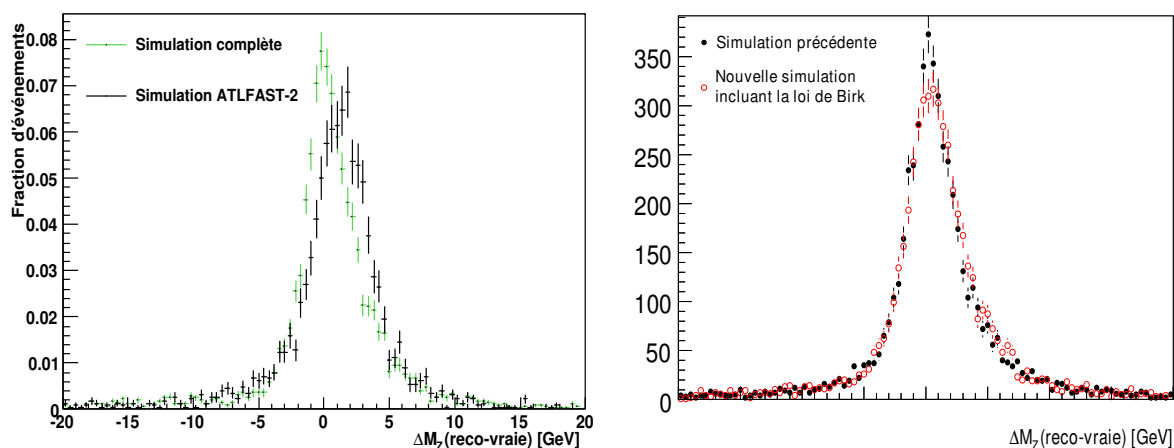
FIG. 2.15 : A gauche : Effets sur la masse reconstruite du boson Z de l'utilisation d'une simulation rapide non satisfaisante. A droite : Après l'ajout de l'utilisation de la loi de Birk dans la simulation du signal dans le pré-échantillonneur, l'échelle d'énergie des électrons n'est plus correctement étalonnée et la masse reconstruite du Z est déplacée de \sim 0.2\% .
