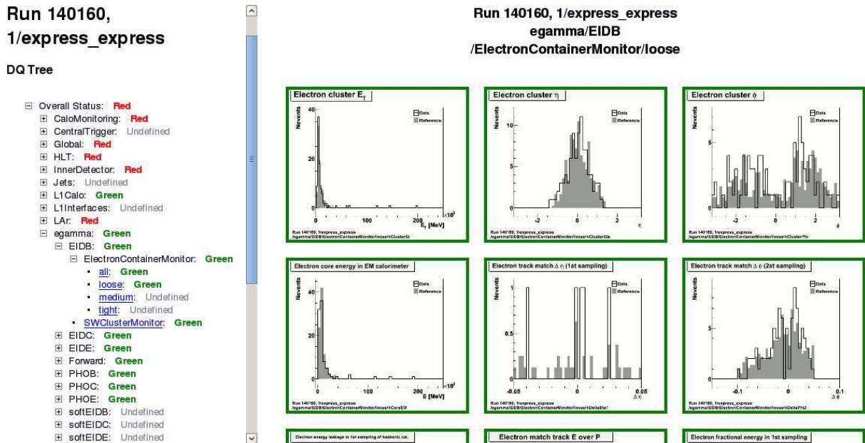
FIG. 3.17 : Interface web d’affichage des histogrammes de contrôle de qualité, ici pour une prise de données de collisions à 900 GeV dans le centre de masse au cours de laquelle le détecteur à pixels était éteint.
