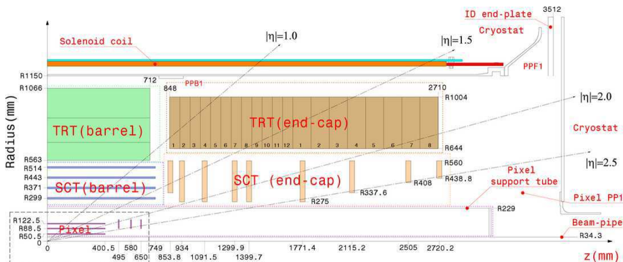
FIG. 2.5 : Schéma du quart ( z > 0, \eta > 0 ) du détecteur interne montrant les différentes couches de sous-détecteurs et leurs dimensions.
