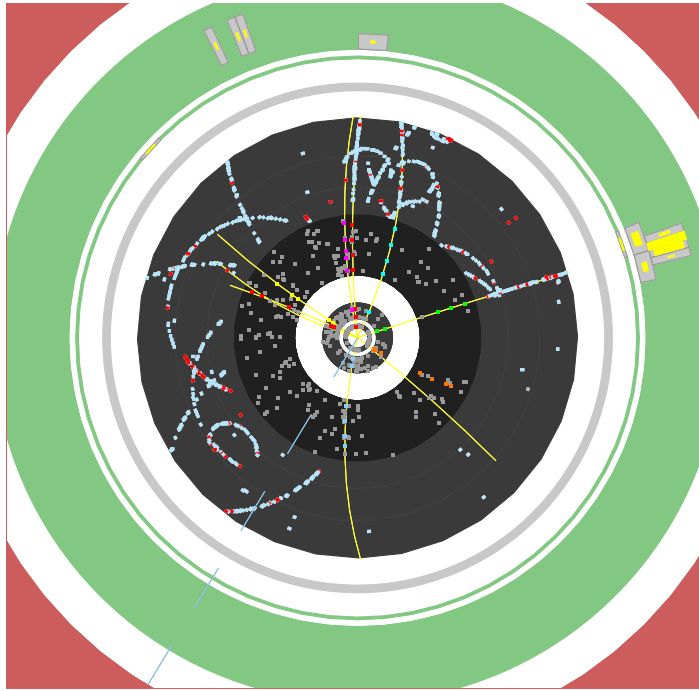
FIG. 3.2 : Vue du détecteur de traces dans le plan XY pour un candidat 1 W \rightarrow e^+\nu_e . Sont visibles du centre vers l'extérieur : les couches de pixels (en gris) contenant un grand nombre de points d'impact, le SCT (en noir), le TRT (en gris clair) ainsi que le calorimètre électromagnétique (en vert). Les points d'impact de chaque trace reconstruite sont groupés par couleur et les points d'impact TRT "haut-seuil" apparaissent en rouge. On peut aussi voir le dépôt d'énergie dans les cellules (en jaune) du calorimètre ( E_T = 34.5 GeV).
