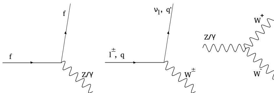
FIG. 1.1 : Vertex d'interaction introduits par le Lagrangien électrofaible. On retrouve à gauche le diagramme QED couplant photons et fermions.
