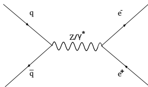
FIG. 1.8 : Diagramme de Feynman pour le processus Drell-Yan à l'ordre dominant.
