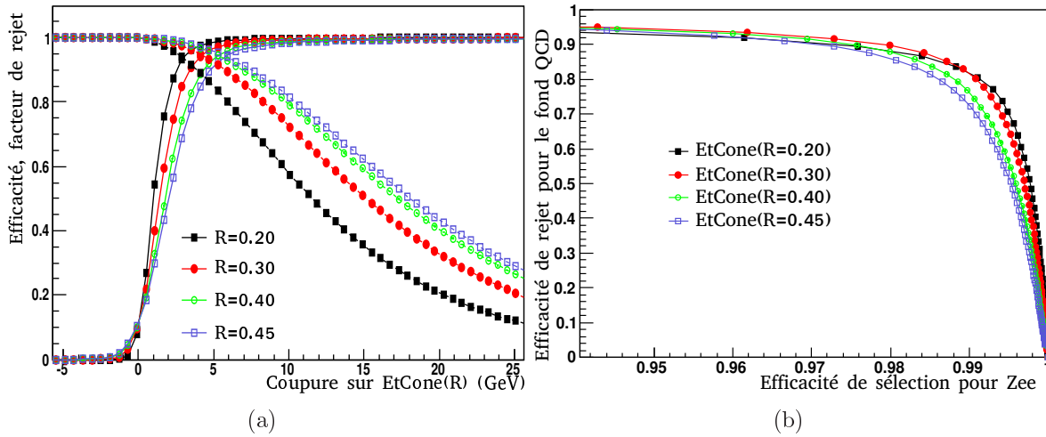
FIG. A.2 : (a) Efficacité de sélection pour les candidats électrons issus du boson Z (traits pleins) et facteur de rejet des hadrons mimiquant les électrons (pointillés) en fonction de la coupure supérieure sur les variables EtCone(R) . (b) Efficacité de rejet sur le fond QCD vs efficacité de sélection pour les électrons issus du Z .
