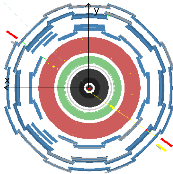
FIG. 4.3 : Événement enregistré lors de la prise de données de cosmiques en 2008 au cours duquel un muon émet un photon de bremsstrahlung visible (en jaune) dans le calorimètre sur une vue en coupe XY d'ATLAS.
