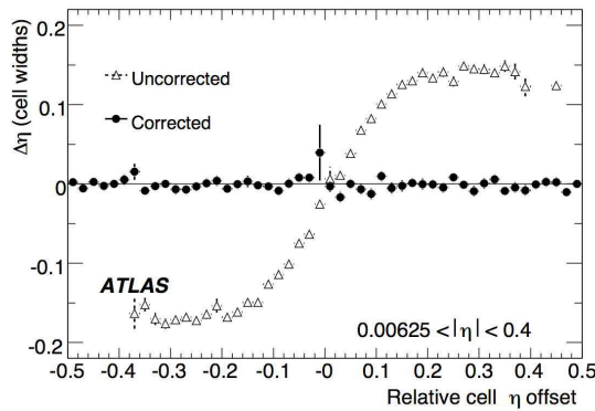
FIG. 3.11 : \Delta\eta vs \nu , la position relative de l'amas à l'intérieur de la cellule, avant et après correction pour des électrons de 100 GeV dans le compartiment avant du calorimètre.
