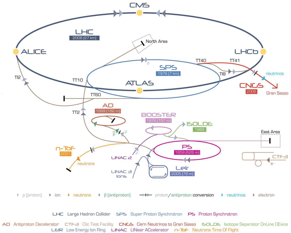
FIG. 1.6 : Complexe des accélérateurs du CERN. Le LHC est le dernier des anneaux (en gris foncé) de la chaîne d'accélérateurs de particules. Les machines plus petites sont utilisées en chaîne afin d'accélérer les particules jusqu'à leur énergie d'injection dans le LHC mais aussi pour fournir à un ensemble de petites expériences les faisceaux qui leur sont nécessaires.
