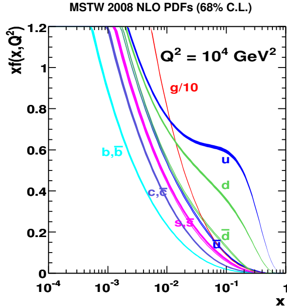
FIG. 1.9 : Fonctions de structure de partons en fonction de la variable de Bjorken x représentant la fraction d'énergie emportée par le parton telles que prédites par le groupe MSTW[41].
