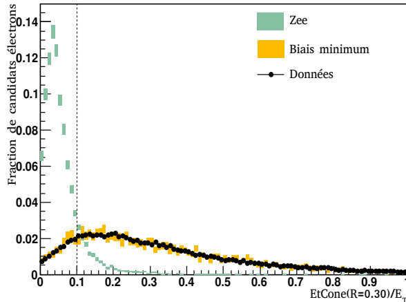
FIG. 5.33 : Distributions normalisées au nombre de candidats électrons de la variable d'isolation \frac{Et_{\text{Cone}}(R=0.30)}{E_T} pour les lots de simulation d'événements de biais minimum et Z \rightarrow e^+e^- et pour les données.
