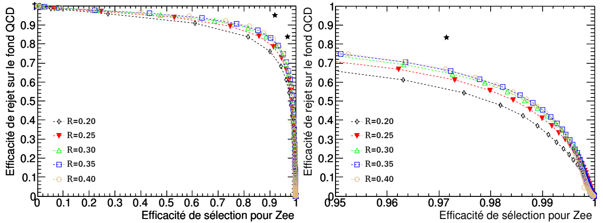
FIG. 5.6 : Efficacité de rejet des jets mimiquant les électrons en fonction de l'efficacité de sélection des électrons issus du Z pour la variable \frac{Et_{\text{cone}}(R)}{E_T} utilisant des tailles de cônes allant de R = 0.20 à R = 0.40 . A droite est figure un agrandissement de la région à grande efficacité de sélection des électrons issus du Z.
