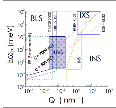
Figure 1: Gammes d'énergie h et de vecteur de diffusion Q sondés par différentes techniques de diffusion inélastique de rayonnement. Les principales utilisées dans ce travail sont la diffusion Brillouin de la lumière visible (BLS), la diffusion inélastique du rayonnement ultraviolet (IUVS) réalisée sur le nouvel instrument du synchrotron Elettra, ainsi que la diffusion inélastique des rayons X (IXS) réalisée à l'ESRF.
