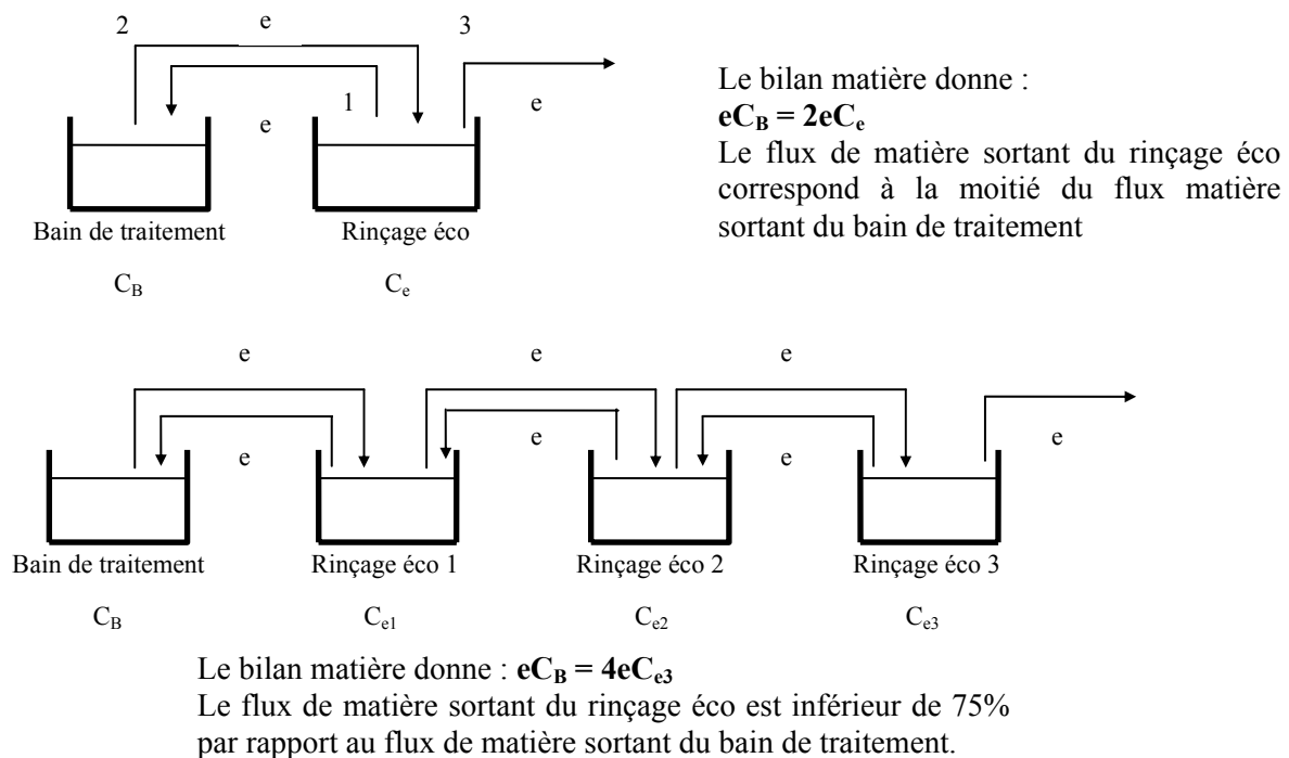
Figure 18 : Comparaison des flux sortant entre l'intégration d'un rinçage éco et de quatre rinçages éco
