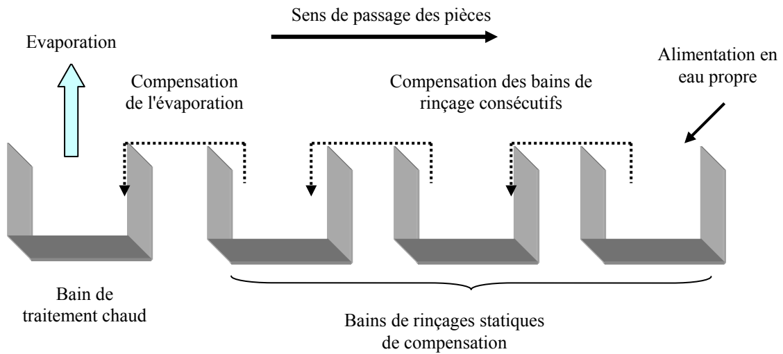
Figure 20 : Schématisation d'une chaîne comptant trois rinçages statiques de compensation
