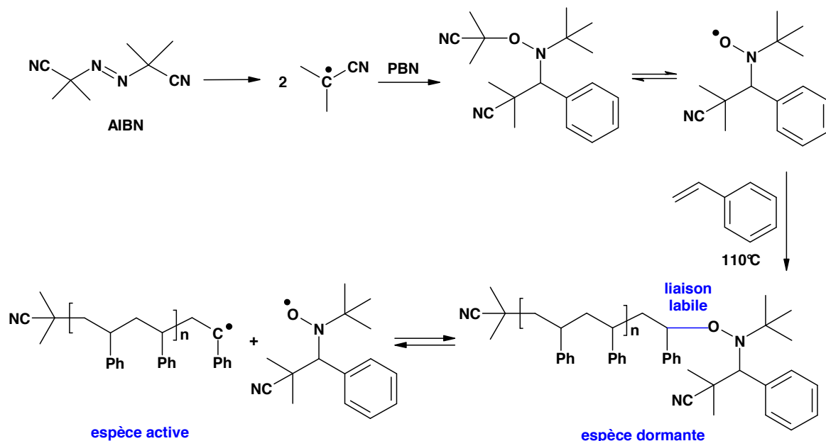
Schéma 171 : Première utilisation des nitrones en CRP
