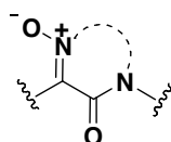
Figure 12 : \alpha_C -dialkylaminocarbonyl-nitron
