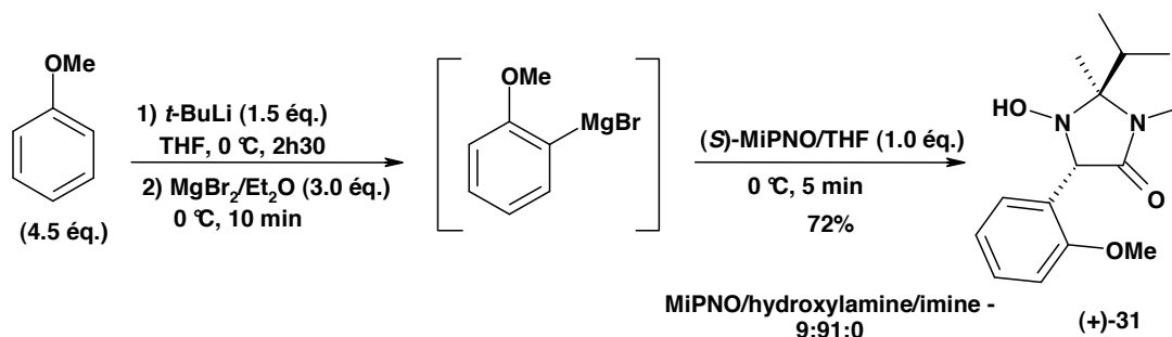
Schéma 108 : Obtention de l'hydroxylamine (+)-31
