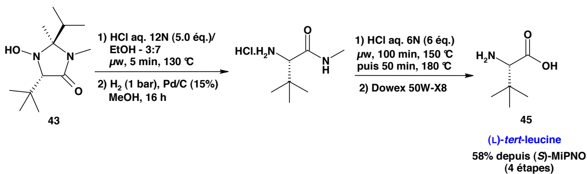
Schéma 123 : Synthèse de la (L)- tert -leucine 45
