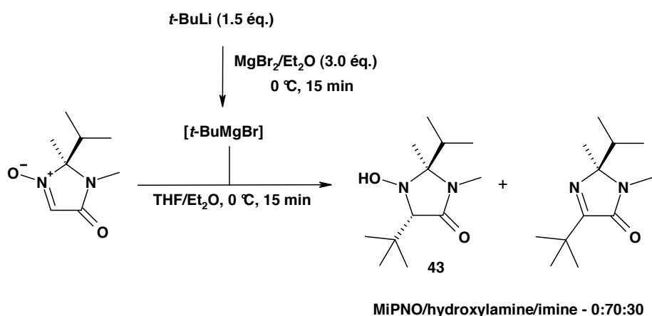
Schéma 121 : Obtention de 43
