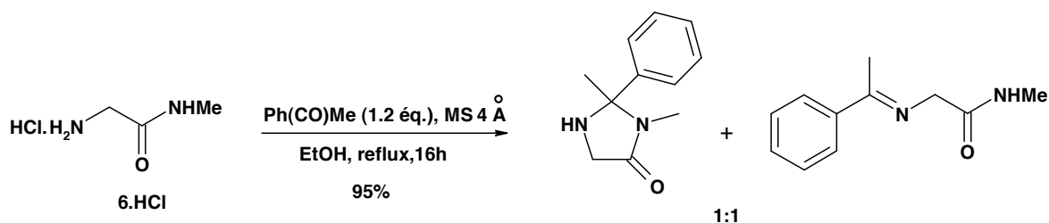
Schéma 59 : Cyclisation de 6·HCl avec l'acétophénone
