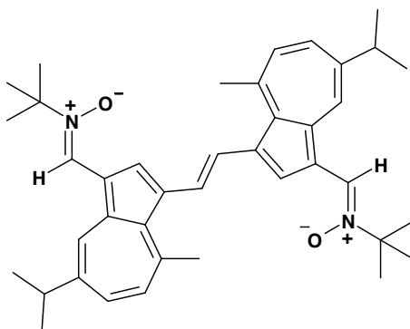
Figure 60 : STAZN
