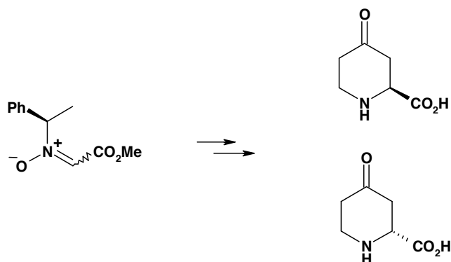
Schéma 28 : Synthèse simultanée des acides (2 S )- et (2 R )-4-oxopipécoliques selon A. Brandi
