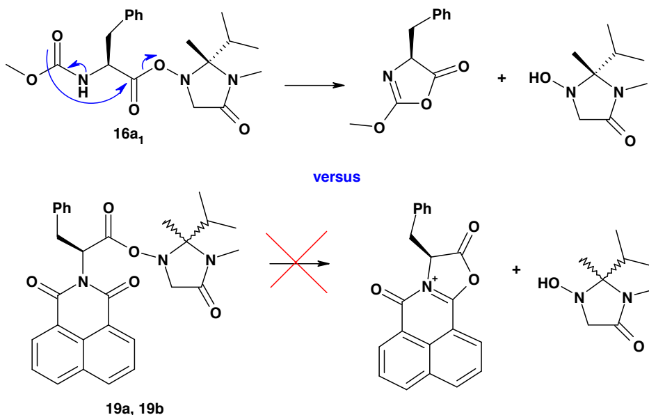
Schéma 77 : Hypothèse de la libération de l'hydroxylamine favorisée par la formation d'une oxazolone
