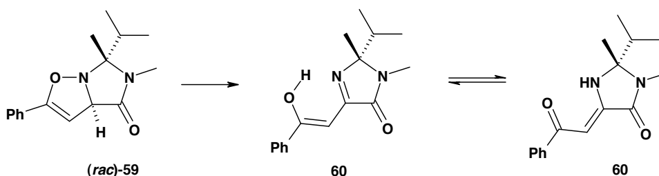
Schéma 155 : Structures tautomères du sous-produit 60
