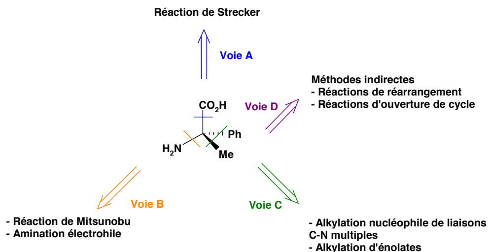
Figure 40 : Voies de synthèse des \alpha -aryl, \alpha -méthylglycines
