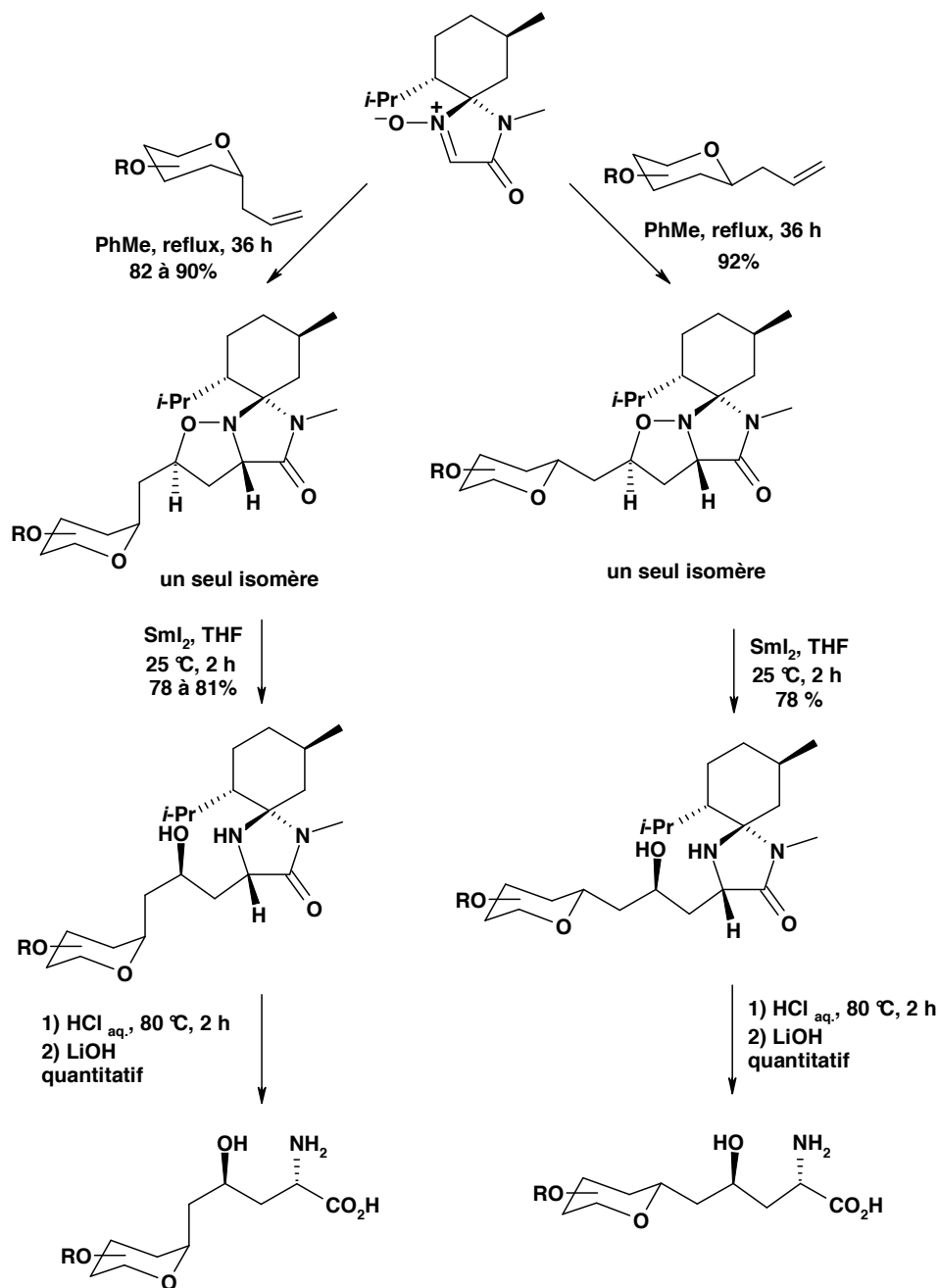
Schéma 37 : Synthèse de \gamma -hydroxy- \alpha -amino-acides C-glycosylés par cycloaddition selon H.-A. Altenbach
