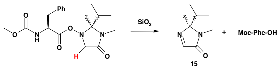
Schéma 72 : Dégradation de l'hydroxylamine O -acylée sur gel de silice
