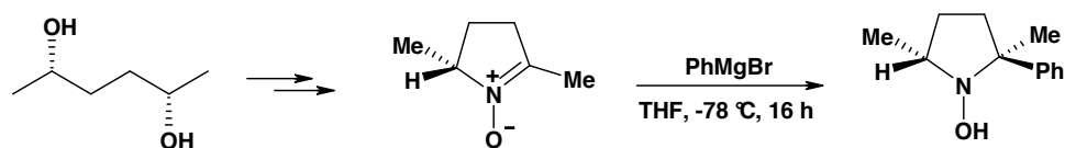
Schéma 19 : Addition nucléophile sur une cétonitronne
