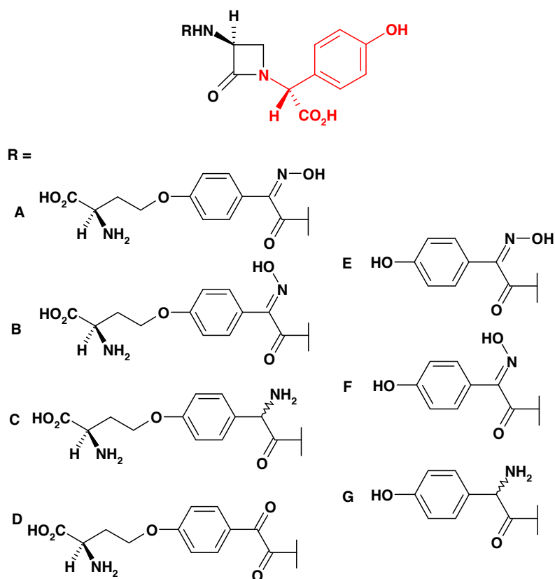
Figure 28 : Nocardicines A-G
