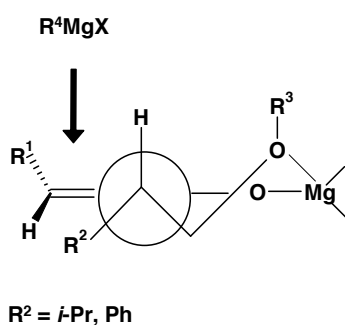
Figure 9 : Etat de transition de la réaction présentée sur le Schéma 17
