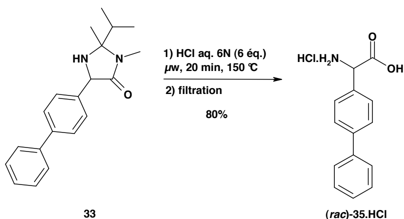
Schéma 112 : Obtention de l'arylglycine ( rac )- 35 ·HCl
