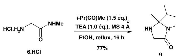
Schéma 58 : Obtention de l'imidazolidinone 9
