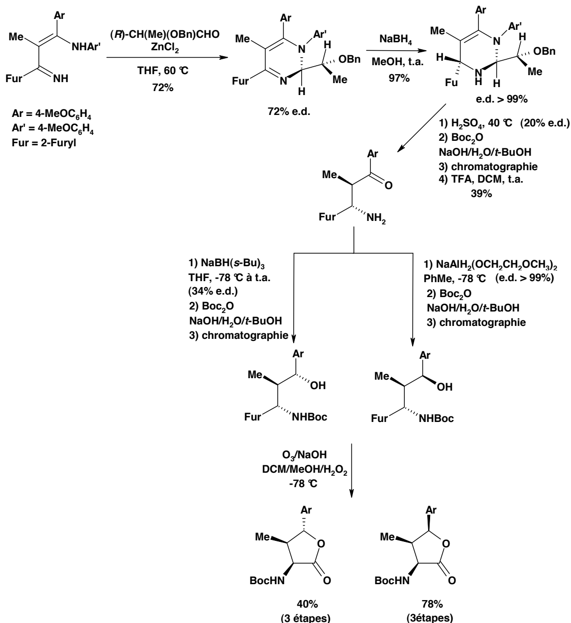
Schéma 151 : Préparation d' \alpha -amino- \gamma -lactones à partir d'un intermédiaire tétrahydropyrimidine
