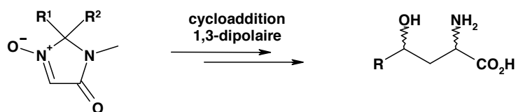
Schéma 46 : Accès à des γ-hydroxy-α-amino-acides
