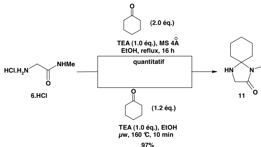
Schéma 61 : Procédures possibles pour la préparation de 11
