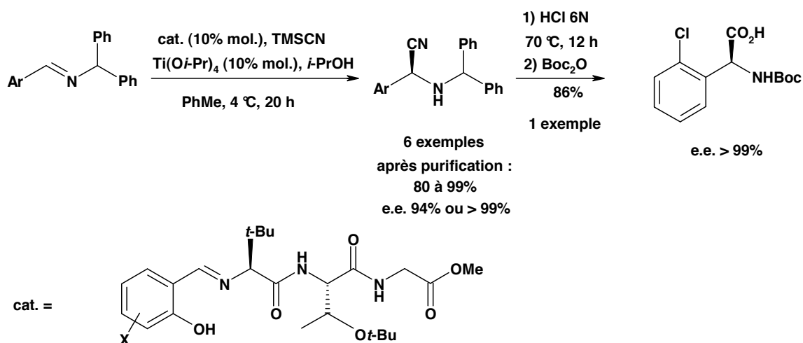
Schéma 100 : Hydrocyanation d'aryladimines par A. H. Hoveyda
