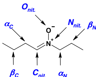
Figure 2 : Nomenclature utilisée dans la suite du manuscrit
