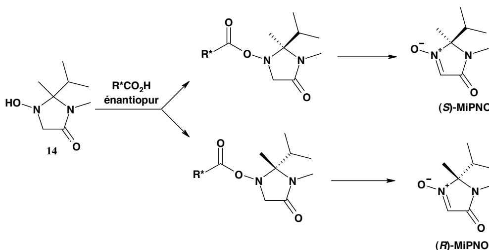
Schéma 66 : Principe de l'obtention de MiPNO énantiopure
