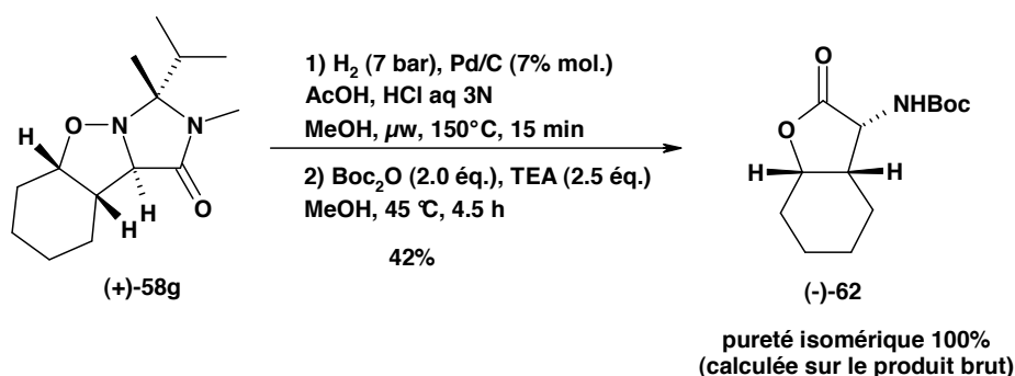
Schéma 160 : Obtention de la N -Boc- \alpha -amino- \gamma -lactone (-)-62
