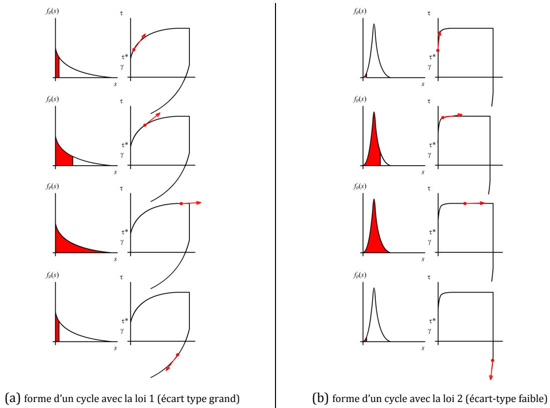
fig. 9 Lien entre le module d'écrouissage et la fonction de distribution f_\rho(s) .
