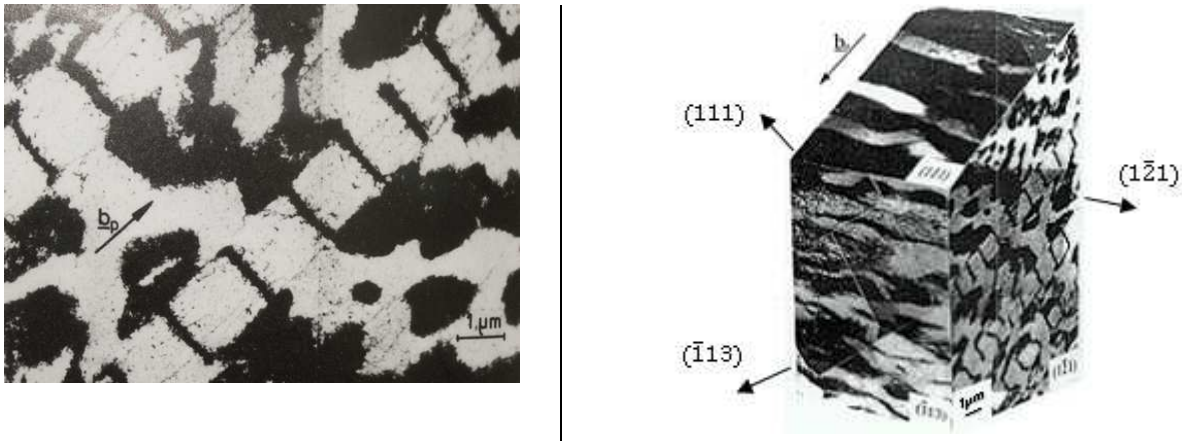
fig. 2 Microstructure de dislocations hétérogène obtenue en fatigue – cristal de Cu [Mughrabi et al. 79].
