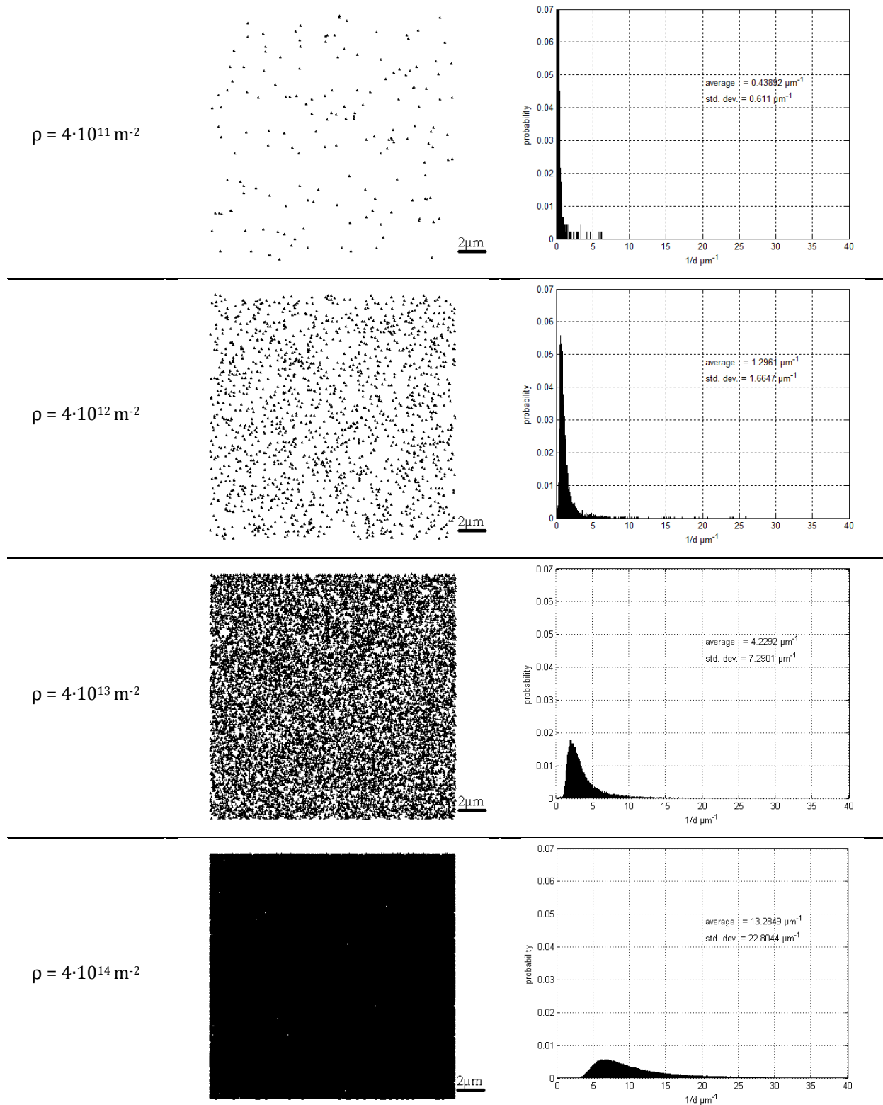
fig. 5 Spectre de répartition de l'inverse de la distance au plus proche voisin pour différentes densités
