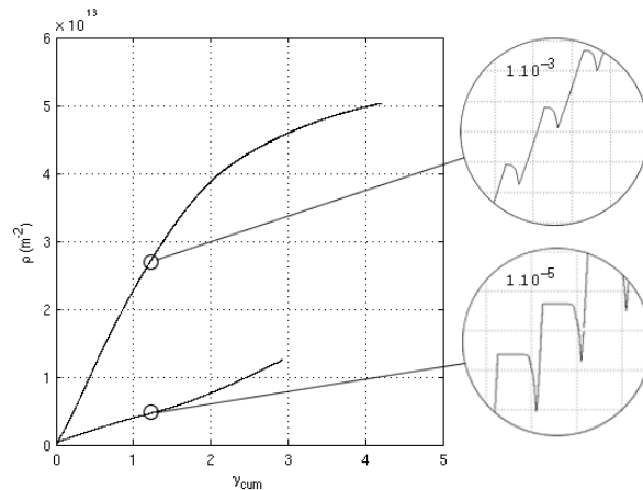
fig. 3 Simulation de l'influence de l'amplitude de la déformation plastique sur la production de dislocations sur le système primaire.
