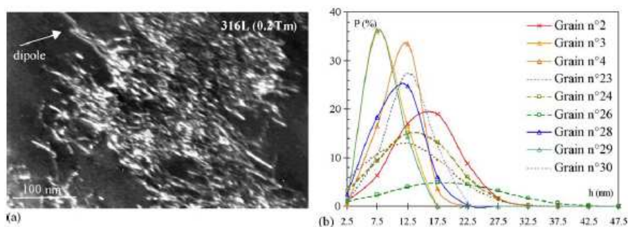
fig. 24 (a) Microstructure dipolaire dans un monocristal AISI 316L (b) Distributions des hauteurs des dipôles, pour différents grains ( \epsilon_p = 10^{-3} , T = 823 K) [Catalao et al. 05].
