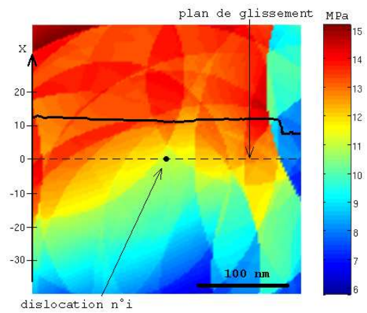
(c) champ de contraintes à longue distance autour du segment n^o i ; c'est le champ créé par les dislocations éloignées du segment. On prendra garde à l'échelle de couleur qui a tendance à trop souligner les variations qui demeurent faibles. La courbe superposée représente cette contrainte le long du plan de glissement : on remarque qu'elle présente une grande longueur d'onde.
