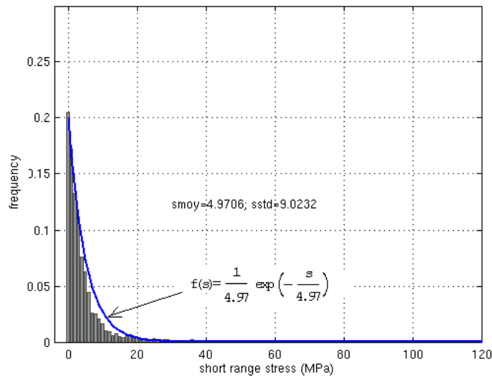
fig. 29 Adaptation de la distribution exponentielle au spectre trouvé en DDD.
