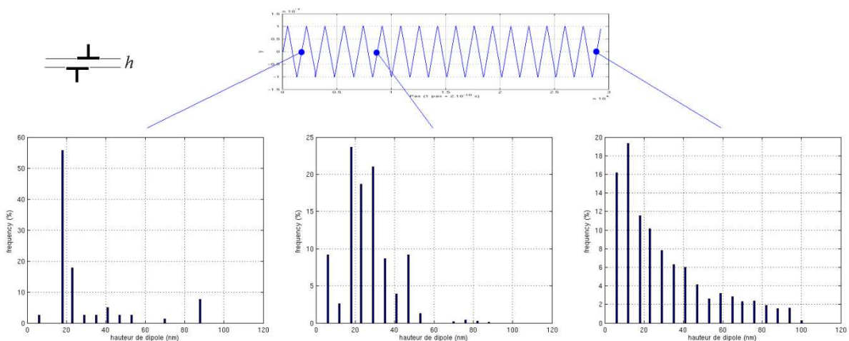
fig. 21 Répartition selon leur taille des dipôles (à caractère coin) dans la microstructure, à différents instants.
