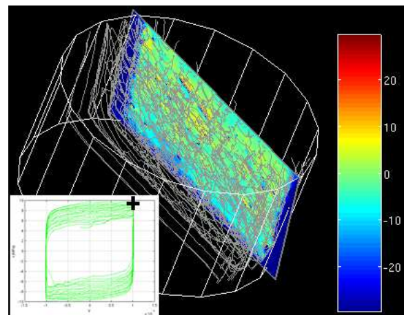
(c) champ de contrainte à longue distance induit par la microstructure, hors effet produit par les dislocations empilées contre le joint de grain. C'est le champ de contrainte à longue distance du monocristal.
