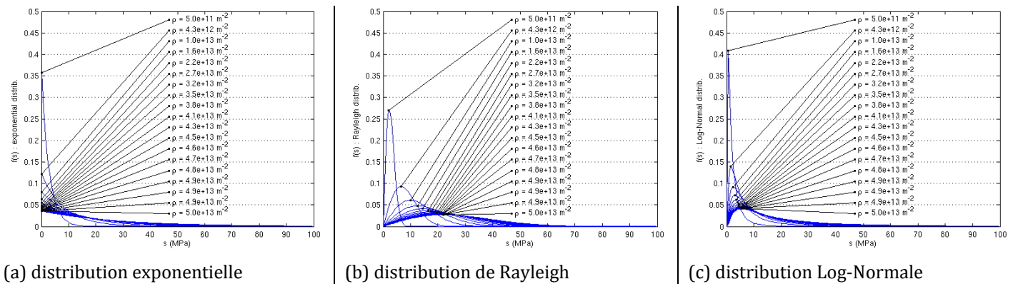
fig. 10 Différentes évolutions possibles de la densité de probabilité f_\rho .
