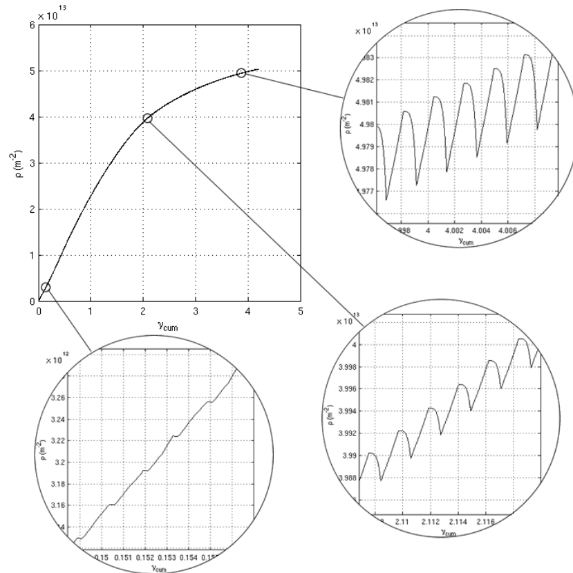
fig. 9 Evolution de la densité de dislocations \rho en fonction de la déformation plastique cumulée \gamma_{cum} .
