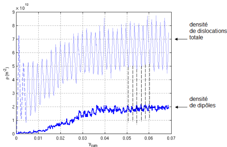
fig. 17 Evolution de la densité de dislocations impliquées dans la formation de dipôles dans la microstructure.
