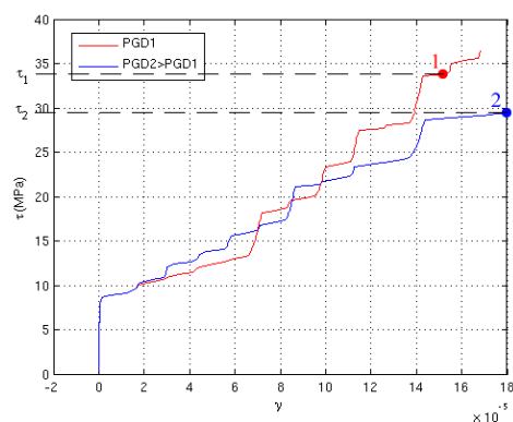
(c) Evolution de la cission pour deux probabilités de glissement dévié
