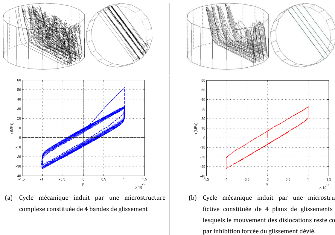
fig. 13 Mise en évidence de l'effet macroscopique des dislocations empilées contre le joint de grain.
