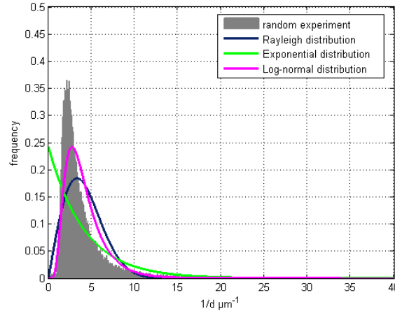
fig. 6 Essai d'adaptation de densités de probabilités analytiques connues sur le spectre obtenu par tirages aléatoires (ici pour \rho = 10^{13} \text{ m}^{-2} ).
