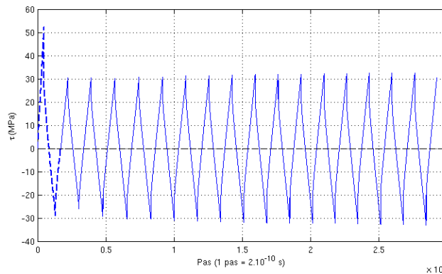
fig. 10 Evolution de la cission appliquée sur le système \frac{a}{2} [1\ 1\ 0] (1\ \bar{1}\ \bar{1}) .
