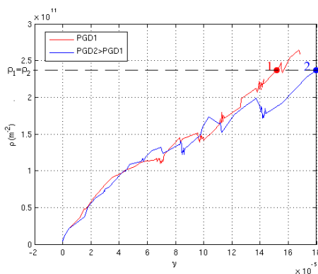
(b) Evolution de la densité de dislocations pour deux probabilités de glissement dévié
