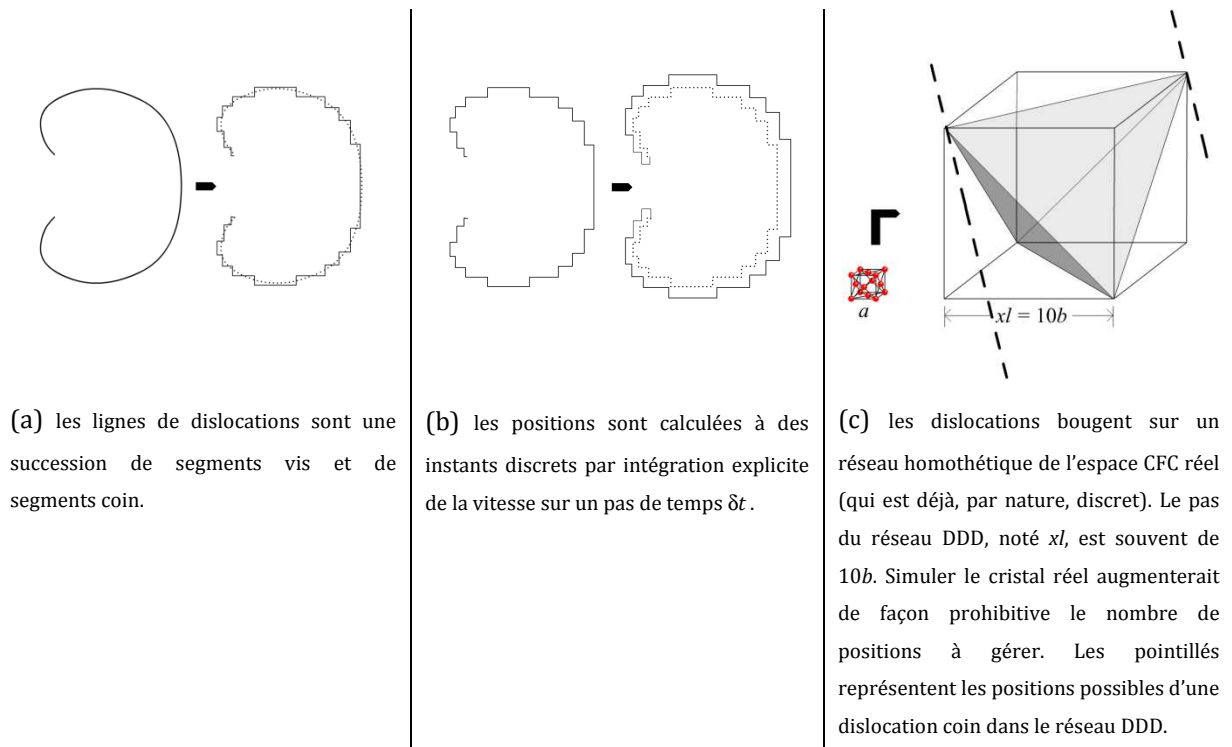
fig. 4 Principe de la triple discrétisation sur laquelle repose le code DDD.
