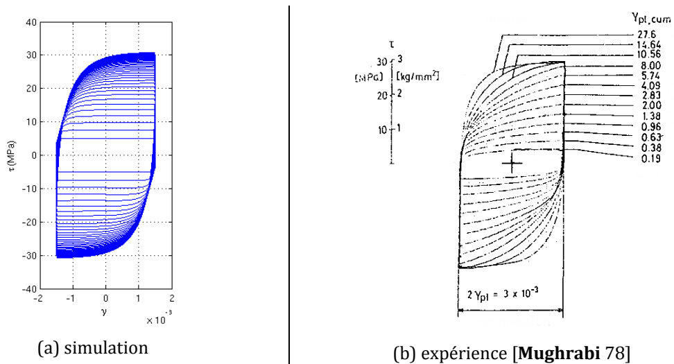
fig. 1 Comparaison modèle – expérience du comportement mécanique sous une sollicitation cyclique d'amplitude \Delta\gamma/2 = \pm 1,5 \cdot 10^{-3} .
