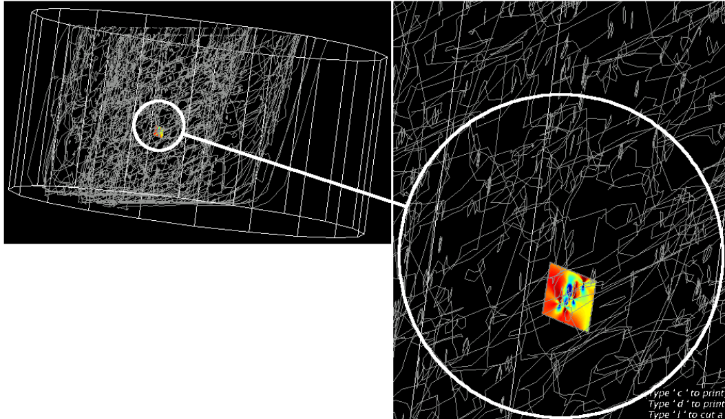
(a) situation dans la microstructure du segment n^o i sur lequel on calcule les contraintes à courte et à longue distance
