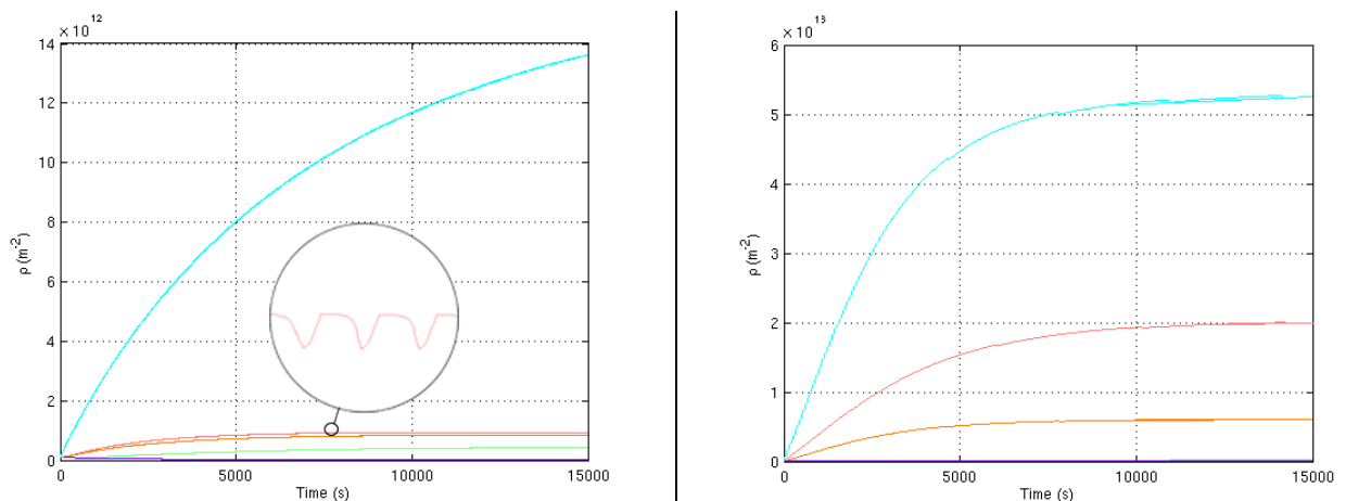
(a) \Delta\gamma = \pm 1 \cdot 10^{-3} : on note que la densité sur les systèmes secondaires sature très vite, par effet de réversibilité
