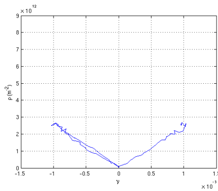
(a) fluctuation de la densité de dislocations induite par une microstructure fictive constituée de 4 plans de glissements dans lesquels le mouvement des dislocations reste confiné, par inhibition forcée du glissement dévié. On montre facilement [Déprés 06]
