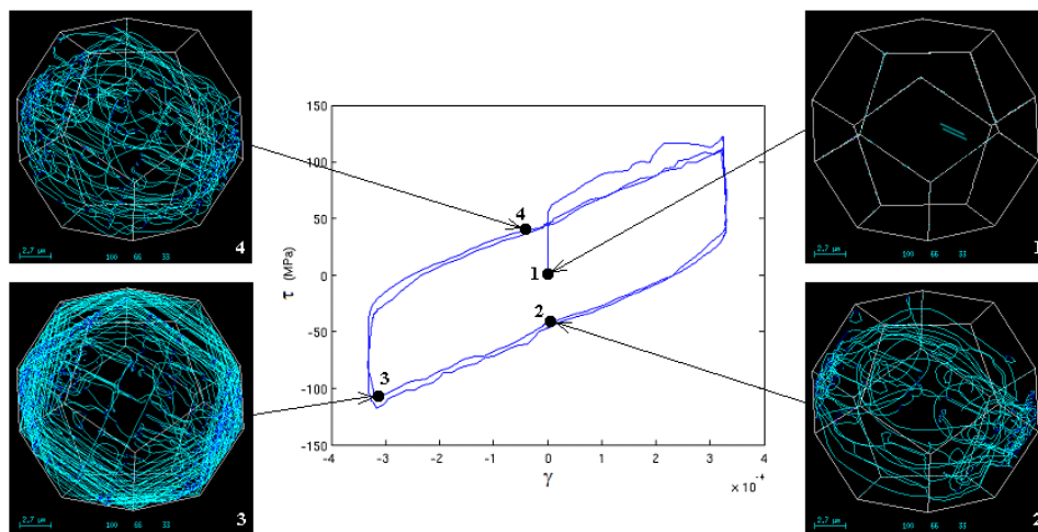
fig. 3 Microstructure de dislocations générée par sollicitation cyclique d'un grain CFC orienté en glissement simple et cycle associé {Cission résolue sur le système B4 – Déformation plastique}.
