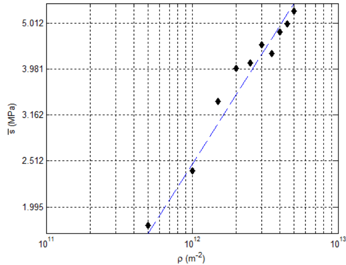
fig. 30 Lien ( log-log ) entre la moyenne de la distribution \bar{s} et la densité de dislocations \rho . Les points noirs sont issus de l'étude DDD, la droite en pointillé est la meilleure approximation linéaire du nuage de point.
