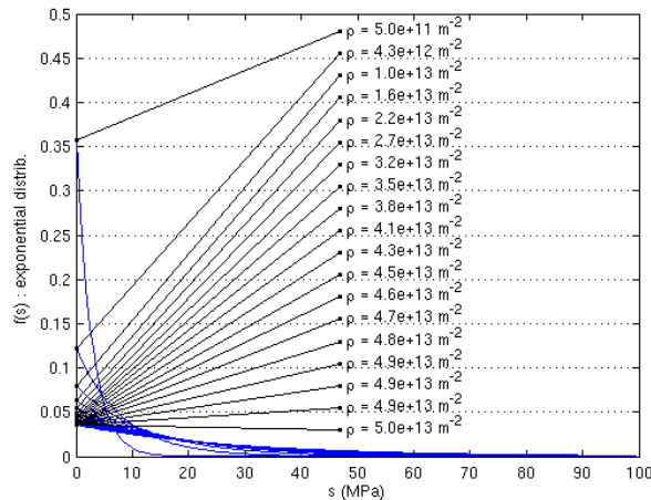
fig. 10 Evolution de la densité de probabilité f_{\rho}(s) en fonction de la densité de dislocations \rho .
