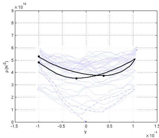
fig. 19 Schématisation sur un cycle de l'évolution de la densité de dislocations dans un monocristal.
