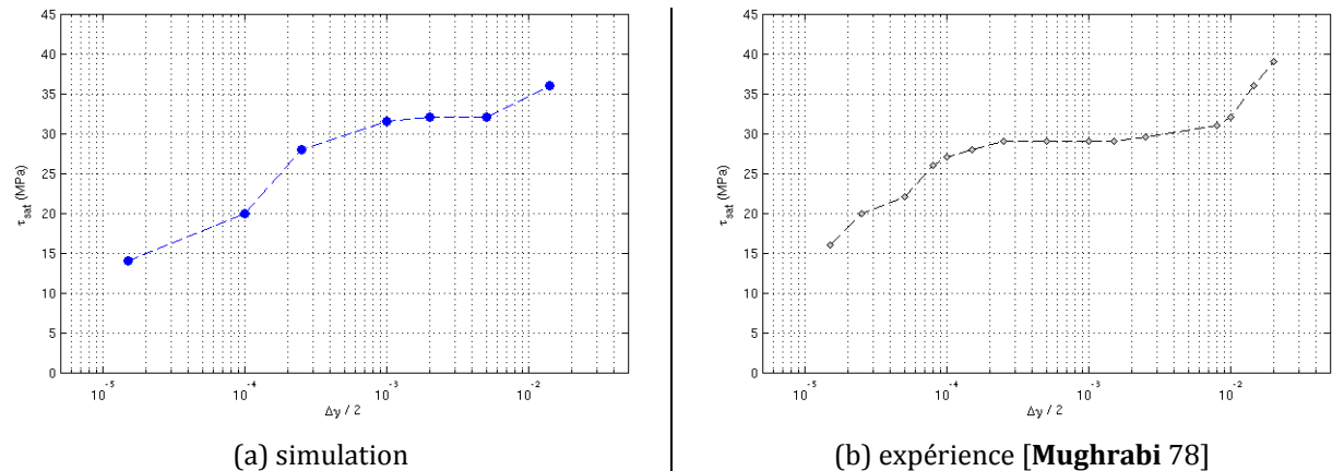
fig. 4 Courbe contrainte-déformation cyclique \tau_{\text{sat}} = f(\Delta\gamma) .
