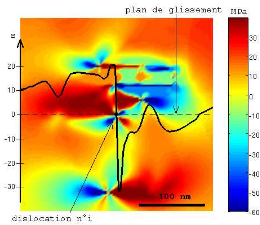
(b) champ de contraintes à courte distance autour du segment n^o i ; c'est le champ créé par les dislocations présentes dans un rayon de coupure r_c autour de la dislocation. La courbe superposée représente cette contrainte le long du plan de glissement : on remarque qu'elle présente un longueur d'onde faible.
