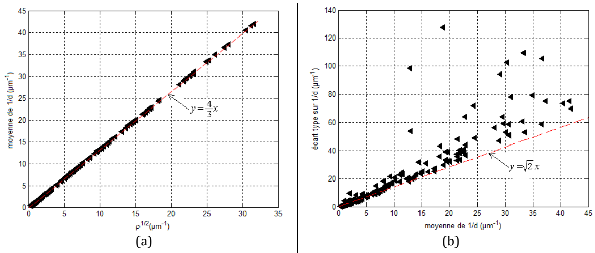
fig. 4 Lien entre : (a) \sqrt{\rho} et \overline{1/d} et (b) \overline{1/d} et \sigma_{1/d} pour des microstructures 2D de densités aléatoires.
