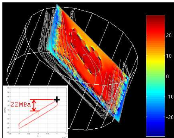
(b) champ de contrainte à longue distance produit par une microstructure fictive constituée de 4 plans de glissements dans lesquels le mouvement des dislocations reste confiné par inhibition forcée du glissement dévié. Il est quasi uniforme à l'intérieur de l'empilement.
