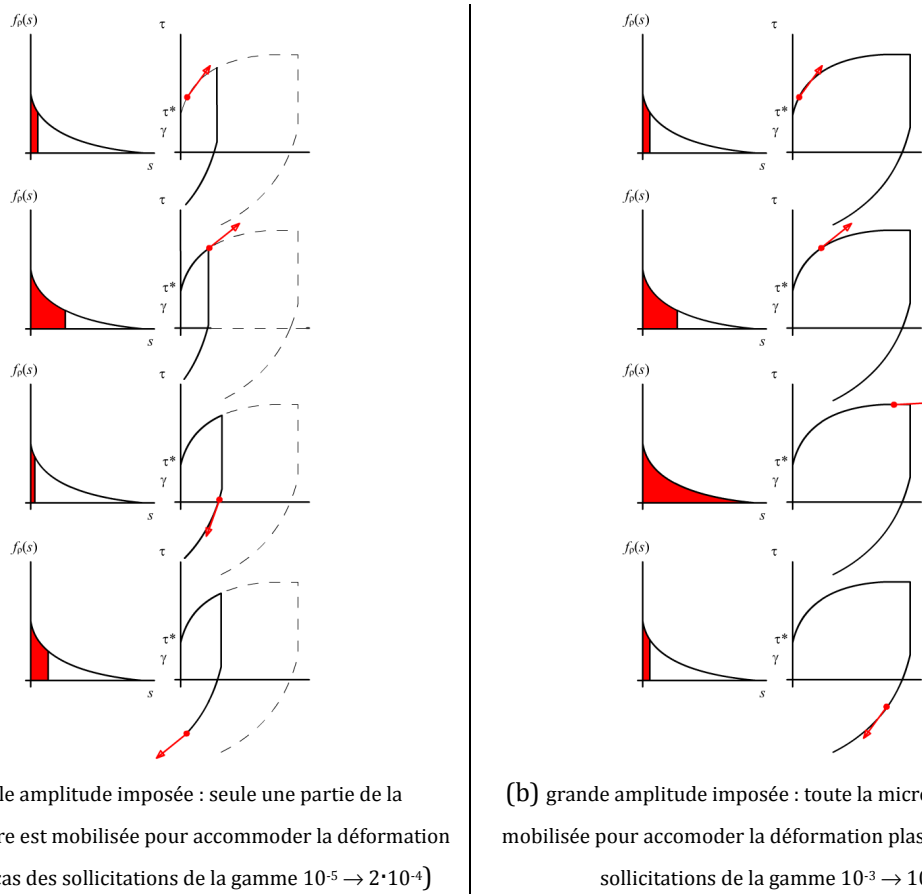
fig. 6 Lien entre la quantité de dislocations mobilisée (en rouge) et la forme du cycle.
