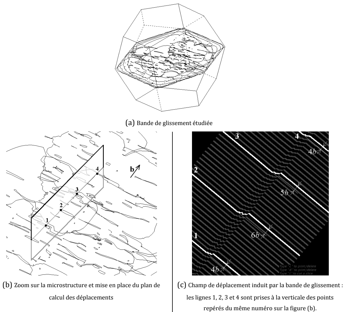
fig. 22 Mise en évidence de l'hétérogénéité de déformation induite par les dipôles dans une microstructure simple.
