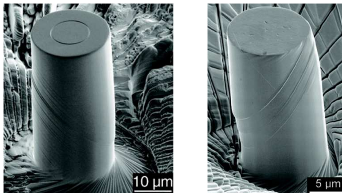
fig. 1 Marches en surface observée au MEB sur un micro-monocristal de Ni [Dimiduk et al. 05].
