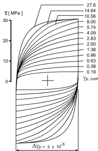
fig. 15 Boucles d'hystérésis mesurées dans le Cuivre monocristallin.
