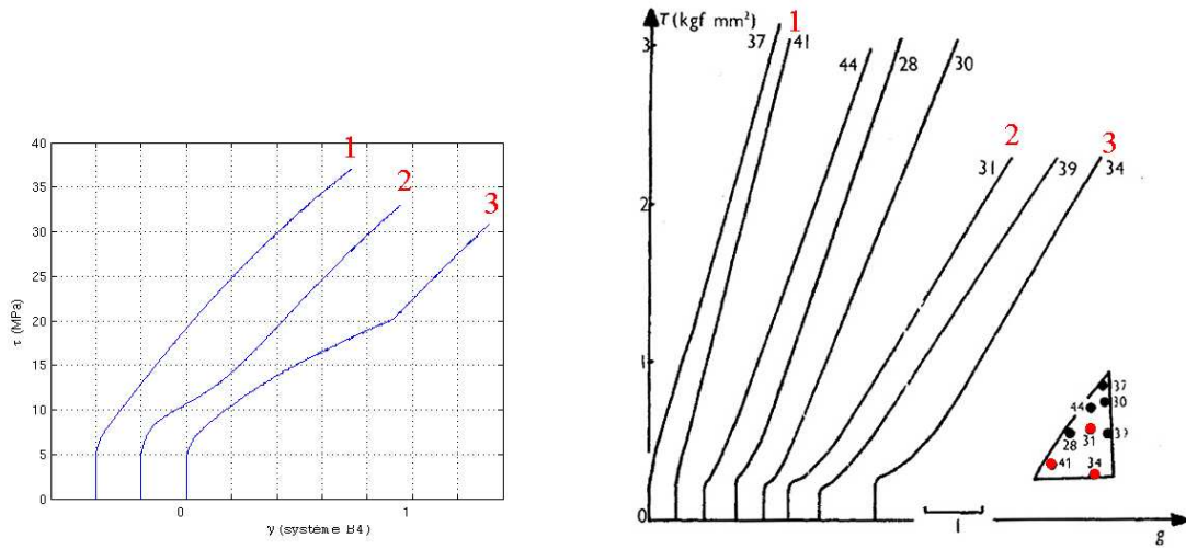
(a) Comportement mécanique du système B4 en traction monotone d'un monocristal de cuivre pour différentes orientations. Expérience tirée de [Jaoul 08].
