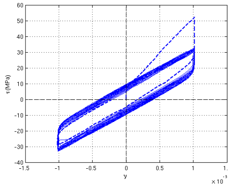
fig. 11 Boucle d'hystérésis correspondant à l'essai.
