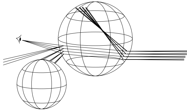
Figure 1.1 : Groupes de rayons rencontrant une sphère réfléchissante et réfractante.
