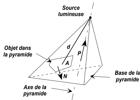
Figure 1.51 : Facteur de forme des ombres.
