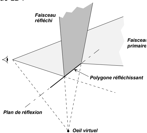
Figure 1.25 : Construction d'un faisceau de réflexion.
