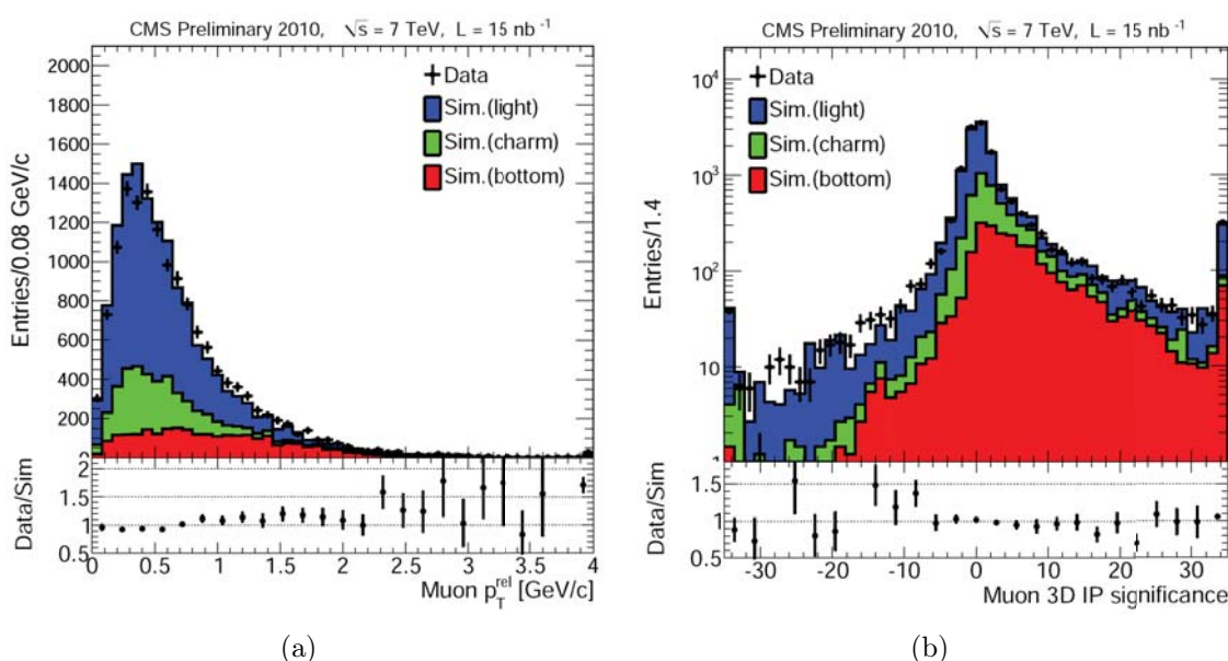
FIG. 4.16 – Distributions du p_T relatif (a) et du paramètre d'impact 3D (b) du muon utilisés au sein de l'algorithme “Soft Muon” sur les premières données [115]. Les distributions comparent les premières données avec la simulation et sont accompagnées du ratio données/simulation.
