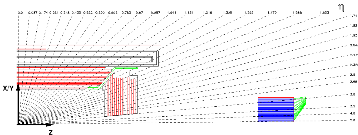
FIG. 1.16 – Quart d'une coupe transversale du calorimètre hadronique
