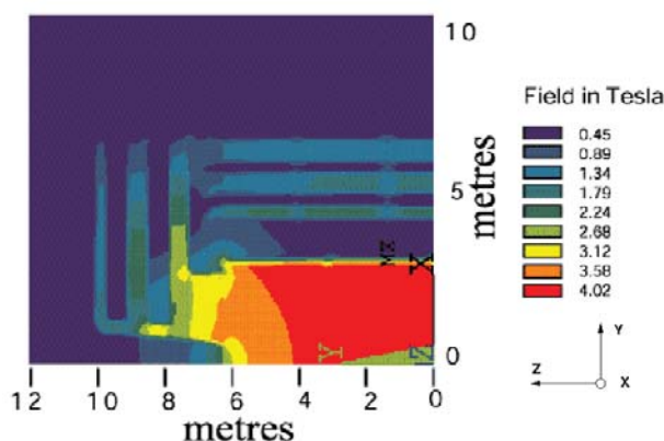
FIG. 1.11 – Valeur du champ magnétique dans le détecteur CMS
