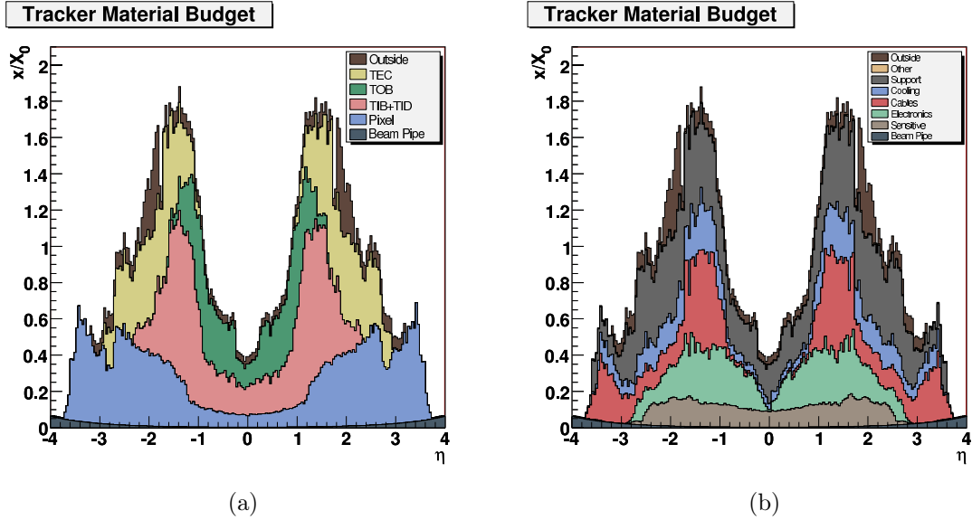
FIG. 2.6 – Quantité de matière rencontrée en unité de longueur d’interaction en fonction \eta détaillée en sous-détecteurs (a) et en fonctionnalités (b)[42].
