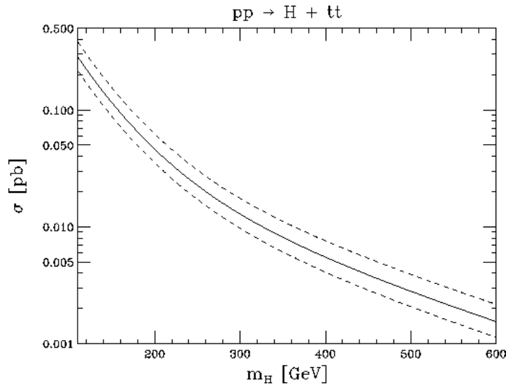
FIG. 3.13 – Section efficace de production t\bar{t} H^0 à l'ordre LO pour \sqrt{s} = 7 TeV en fonction de la masse du boson de Higgs. Les pointillés indiquent les incertitudes provenant des échelles de renormalisation et de factorisation
