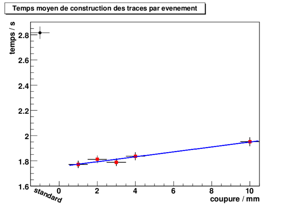
FIG. 2.22 – Temps de calcul moyen de la reconstruction des traces pour différentes valeurs de coupure de la contrainte \sigma_z autour du vertex pour les paires mixtes sur un lot de données simulées t\bar{t}
