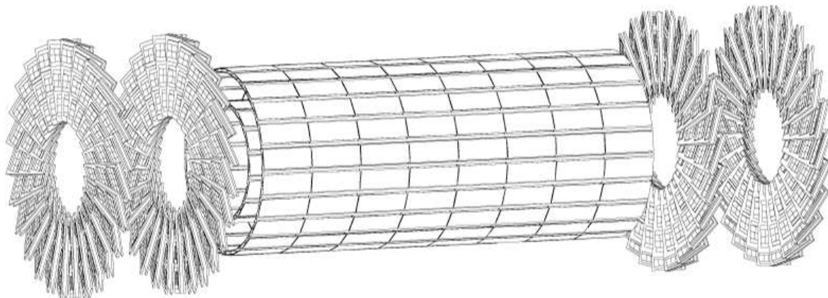
FIG. 1.13 – Vue tridimensionnelle du détecteur à pixels
