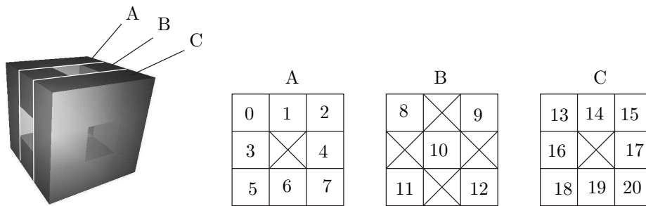
FIG. 7.7 – Les sous cubes de l'élément de base sont numérotés. La fonction getRepere donne la translation entre le repère de l'élément (centré sur celui-ci) et les 20 sous repères.
