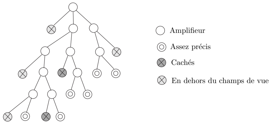
FIG. 5.6 – En fonction de l’observation, l’arbre d’évaluation va se générer jusqu’à sa complexion, c’est-à-dire quand toutes les conditions d’arrêt des feuilles sont positives. Comme les conditions d’arrêt dépendent de l’observation, l’arbre d’évaluation est différent à chaque affichage.
