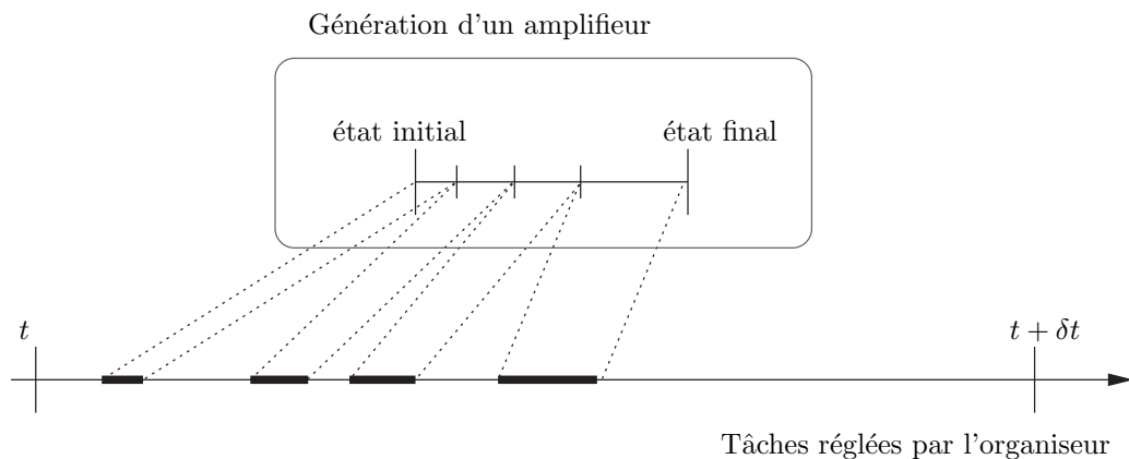
FIG. 6.3 – L'organiseur cadence le générateur pour que celui-ci évalue un amplifieur en plusieurs fois. En conséquence, l'organiseur reprend non seulement la main à la fin d'une évaluation, mais éventuellement plusieurs fois durant une même évaluation.
