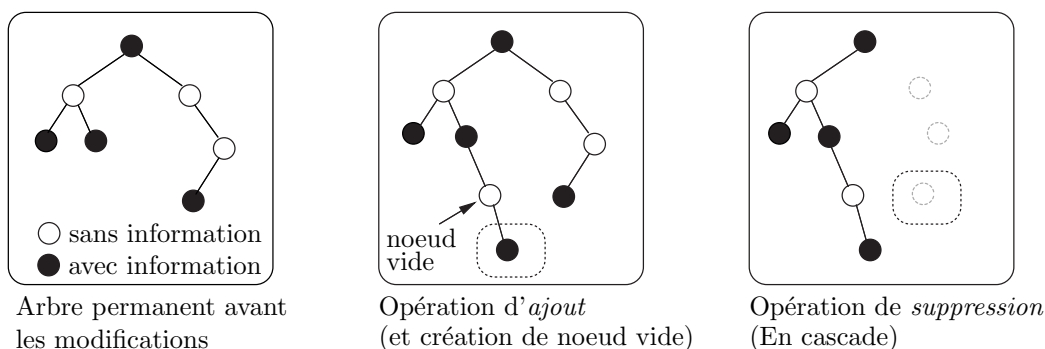
FIG. 6.10 – L'arbre permanent, lors d'ajout ou de suppression d'informations, rajoute ou supprime des noeuds vides afin de garder la taille minimum requise pour accéder à toutes les informations permanentes. Remarquons qu'une conséquence de cela est que chaque feuille de l'arbre contient toujours de l'information.
