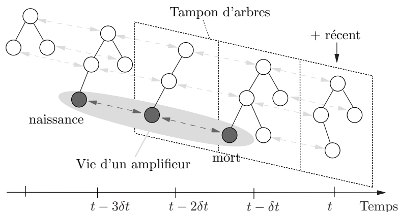
FIG. 6.6 – Chaque amplifieur de chaque arbre d'évaluation stocké dans le tampon d'arbres a connaissance de son successeur et de son ancêtre. Ceci lui permet d'avoir accès aux informations à des temps différents (généralement passés).
