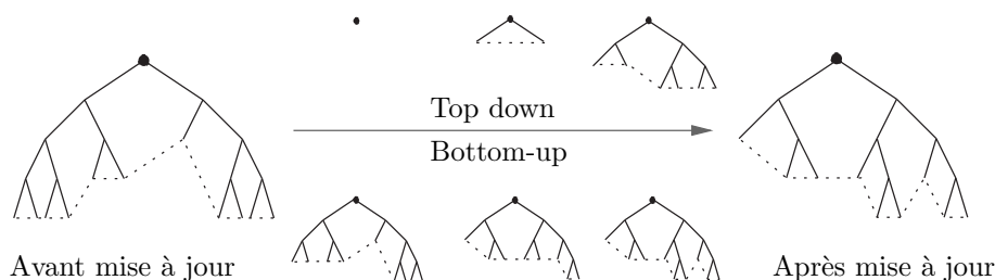
FIG. 3.7 – Lors d’une mise à jour de la figure, deux approches s’opposent. La méthode Top-down commence par la racine et descend vers les feuilles. La méthode Bottom-up commence par les feuilles et remonte vers la racine (elle redescend cependant lorsque des détails sont ajoutés).
