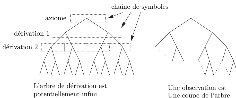
FIG. 3.6 – L'évaluation d'un L-système est ici représentée par un arbre de dérivation (éventuellement cyclique). La chaîne de caractères d'un L-système peut être dérivée à l'infini, mais une observation correspond à une coupe de cet arbre.
