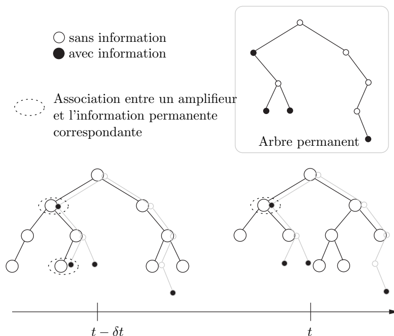
FIG. 6.9 – Cette figure montre l’arbre dynamique à deux pas de temps successif avec, en grisé, l’arbre permanent. L’arbre permanent ne change pas dans le temps. Les données permanentes sont associées à un amplifieur qui, à un instant donné, peut exister ou non. Certains noeuds de l’arbre permanent sont vides et ne servent qu’à atteindre des noeuds non vides.
