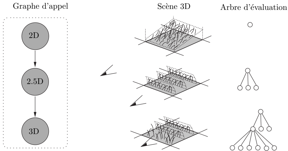
FIG. 5.5 – Lorsque l’observateur se rapproche, l’arbre d’évaluation se développe. Il s’arrête lorsque l’objet est suffisamment précis ou non-visible.
