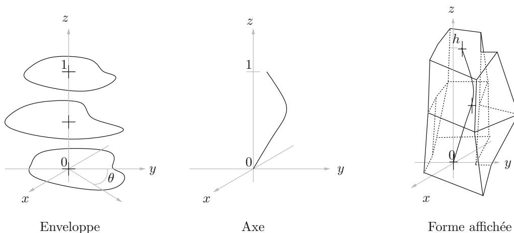
FIG. 7.14 – Deux fonctions définissent un super-cylindre. La forme s’affiche avec une mise à l’échelle à la volée et un échantillonnage en z de l’axe et en (z, \theta) de l’enveloppe.
