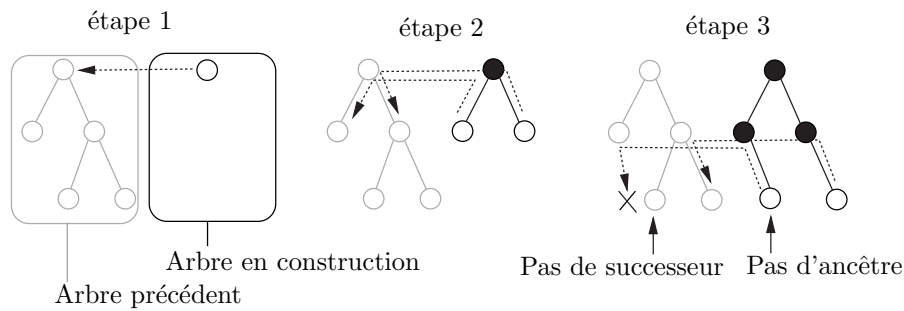
FIG. 6.8 – L’ancêtre d’un noeud est ”le fils de l’ancêtre de son père”. Cette formulation ne fait intervenir qu’une recherche d’identifiant local, c’est-à-dire la recherche d’un fils particulier parmi ses frères. Nous verrons en 7.2 que le coût de cette recherche dépend des choix que fait le créateur. Dans le meilleur des cas, elle est effectuée en coût constant.
