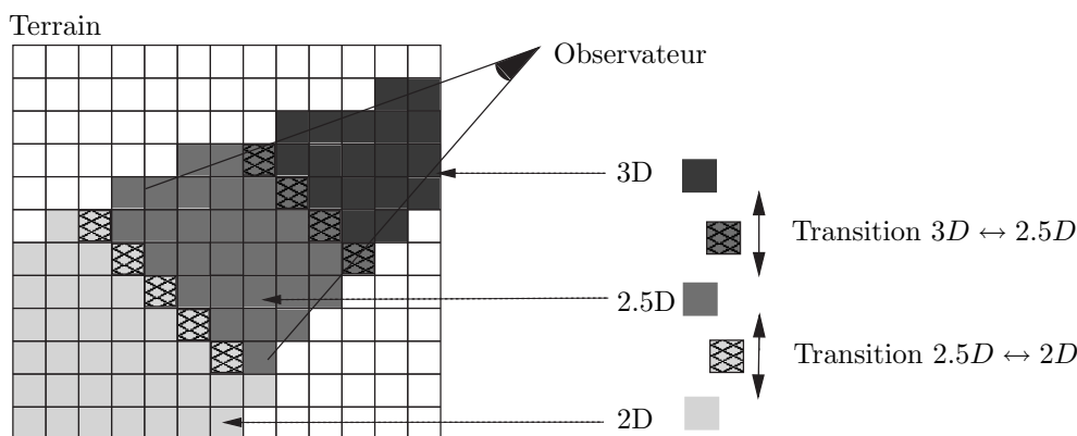
FIG. 4.3 – Les carrés d’herbe visibles du terrain peuvent être représentés par trois niveaux de détail différents. Ces niveaux de détail sont déterminés en fonction de la distance à la caméra. Entre chaque zone, des carrés d’herbe transitent d’un niveau à l’autre.
