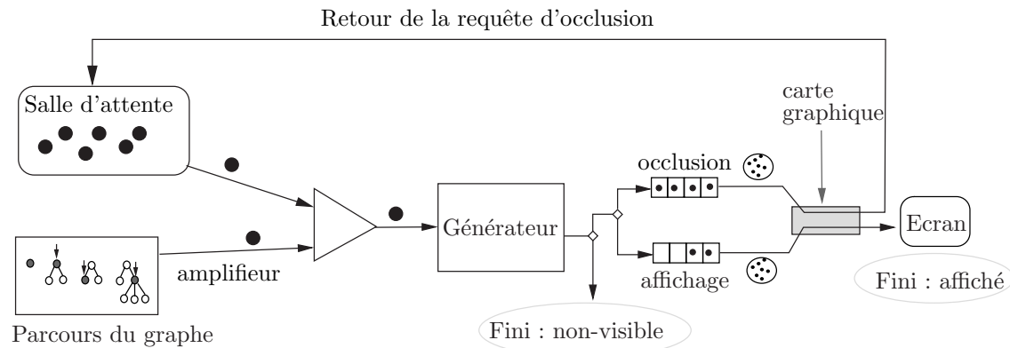
FIG. 6.24 – Afin d’assurer un parallélisme efficace entre le GPU et le CPU, la génération de l’arbre d’évaluation est jalonnée de files d’attente. Notamment, les files d’attentes de l’affichage et de l’occlusion ont pour premier objectif de grouper les commandes OpenGL. De plus, la file d’attente de l’affichage applique un tri local d’avant vers l’arrière pour compléter le tri réalisé lors du parcours du graphe.
