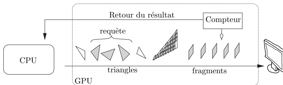
FIG. 6.20 – Le CPU envoie au GPU des primitives graphiques qui sont décomposées en fragment. Un compteur compte ces derniers et renvoie le résultat au CPU. Le problème de l’asynchronicité souhaitée vient du fait que le CPU rester bloquer pendant que la requête traverse toute le pipe-line de la carte graphique et lui revienne.
