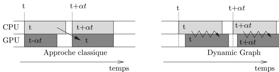
FIG. 6.25 – L'échange complexe que Dynamic Graph fait avec la carte graphique permet d'afficher un modèle en même temps qu'il est animé (évalué). Plus classiquement, les méthodes d'animation affichent usuellement le résultat d'une animation au pas de temps suivant. De ce point de vue, notre approche réduit la latence [LRC + 02] de l'affichage.
