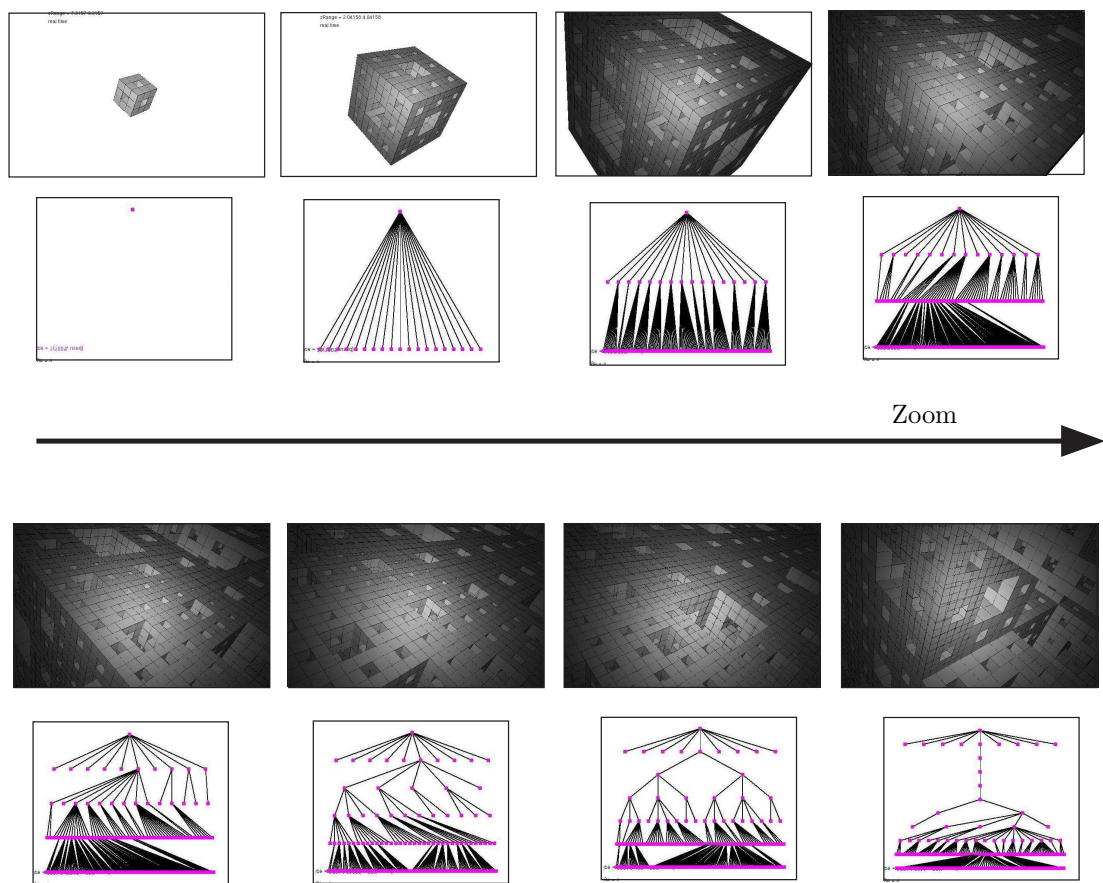
FIG. 7.4 – La visualisation de l'arbre d'évaluation donne un bon aperçu de la complexité de la scène.
