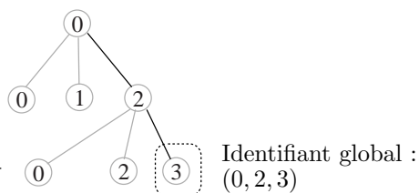
FIG. 6.7 – Un identifiant global est une liste d'identifiants locaux représentant le chemin de la racine à l'amplifieur identifié. Un identifiant local est unique parmi les identifiants des amplifieurs frères. Un identifiant global est unique parmi les identifiants des amplifieurs de l'arbre.
