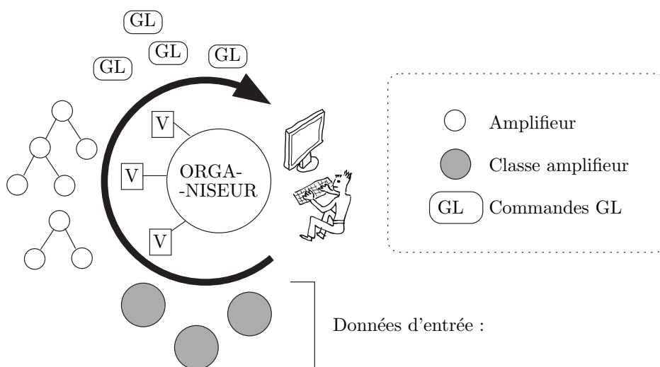
FIG. 5.7 – On reprend ici la figure 5.2 en rajoutant l’organiseur et ses visiteurs. L’organiseur s’occupe du bon ordonnancement des tâches nécessaires aux contraintes émanant de certaines fonctionnalités (tel que l’algorithme de détection d’occlusion).
