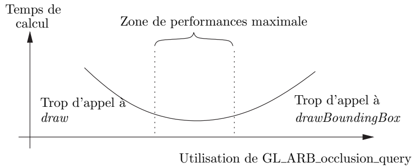
FIG. 6.23 – Comme toute méthode d’optimisation basée sur des tests, il faut s’assurer que le coût de ces derniers ne soit pas au bout du compte nuisible aux performances. En d’autres termes, il faut s’assurer que le test ne coûte pas plus cher que ce qu’il permet d’économiser.
