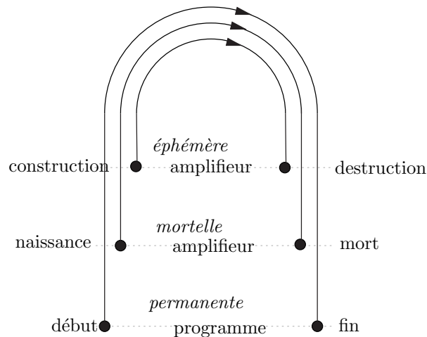
FIG. 7.12 – Plusieurs types de mémoire sont visibles depuis un amplifieur. Chacune d’elles a une durée de vie particulière. La mémoire permanente est allouée pour toute la durée de l’exécution de Dynamic Graph. La mémoire mortelle est allouée à la naissance d’un amplifieur et désallouée à sa mort. La mémoire éphémère est celle stockée dans le tampon d’arbres : elle dure 2 ou 3 pas de temps.
