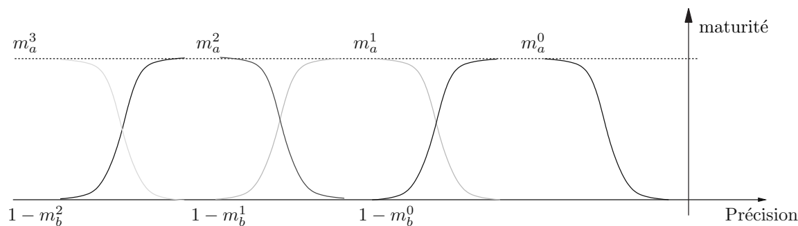
FIG. 7.19 – Les deux maturités sont déclenchées à des précisions bien particulières, assurant une bonne synchronisation entre les amplificateurs père et fils.
