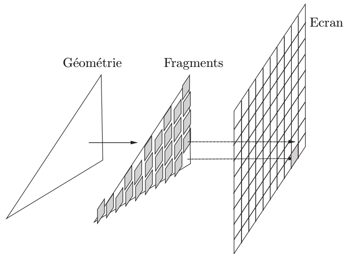
FIG. 2.2 – La géométrie est envoyée à la carte graphique. Elle est projetée et décomposée en fragments [WND99], c’est à dire rasterisée. Puis ces fragments sont envoyés sur l’écran.
