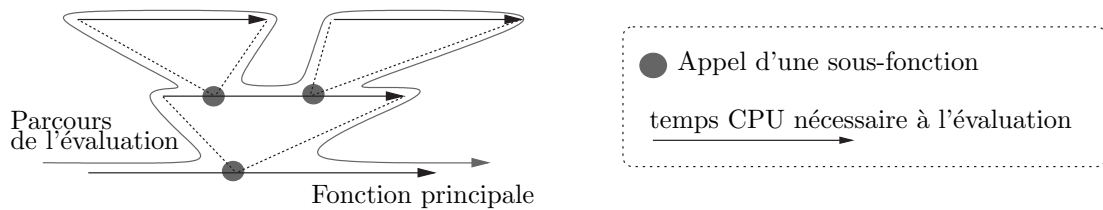
FIG. 5.8 – Dans Dynamic Graph, la construction de l'arbre d'évaluation est parfaitement contrôlée par l'organiseur. Contrairement à de simples fonctions récursives, Dynamic Graph permet de rendre la main à l'organiseur après la fin de l'évaluation de chaque amplifieur. De cette façon, l'organiseur a tous les pouvoirs pour diriger les opérations dans un ordre adéquat.
