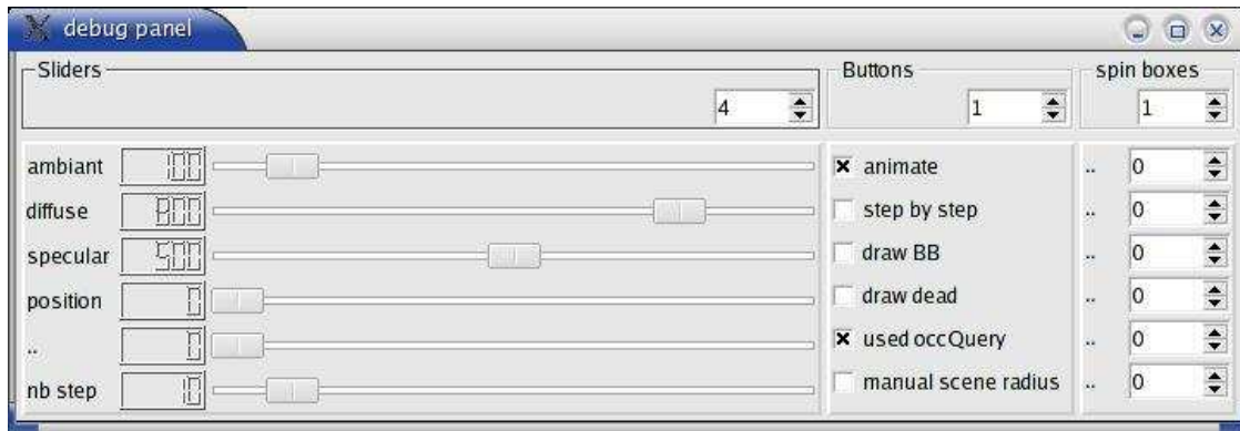
FIG. 7.2 – Le debugPanel offre la possibilité de déclarer et de modifier dynamiquement une infinité autant de valeur que le souhaite le créateur. C’est en quelque sorte la version la plus primitive qui soit d’une interface graphique procédurale. Cet outil est très utile pour contrôler les très nombreux degrés de liberté qu’offre la modélisation procédurale.
