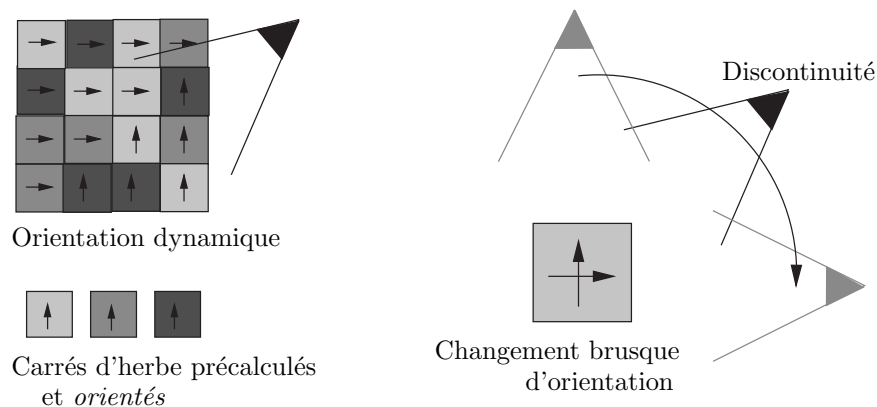
FIG. 4.17 – Les carrés d’herbe, étant constitués de tranches d’herbe orientées, sont eux-mêmes orientés. Si le marcheur tourne autour d’un carré d’herbe sans le quitter des yeux, l’orientation d’un carré d’herbe (en particulier celle des tranches texturées du niveau 2.5D) va changer brusquement, résultant en une discontinuité de l’affichage.
