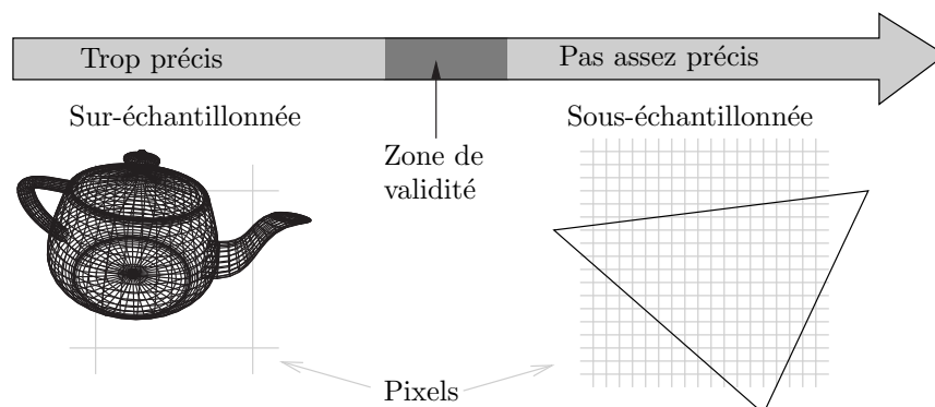
FIG. 6.14 – La précision est représentée par un réel. Une valeur positive signifie que la forme est sous-échantillonnée. Une valeur négative signifie que la forme est sur-échantillonnée. La valeur nulle représente l'échantillonnage idéal. Le but du jeu est ici de se rapprocher au maximum de la valeur nulle.
