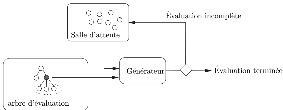
FIG. 6.4 – La salle d’attente récupère les références des amplificateurs dont l’évaluation est incomplète et attend le bon moment pour les remettre dans le circuit.
