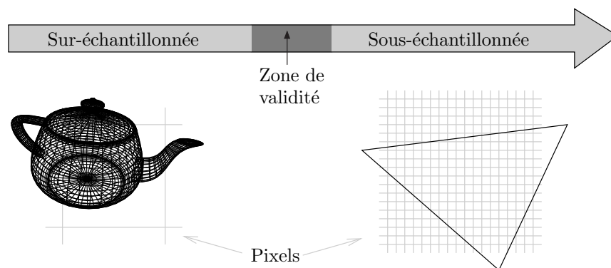
FIG. 2.6 – La projection d’un objet sur l’écran peut être sous-échantillonnée ou sur-échantillonnée . Les méthodes d’anti-aliasing permettent d’agrandir la zone de validité : même si un triangle est un peu trop petit, son affichage sera de bonne qualité. Malheureusement, cet agrandissement est très limité et permet au maximum de gagner un facteur d’échelle de l’ordre de la dizaine.
