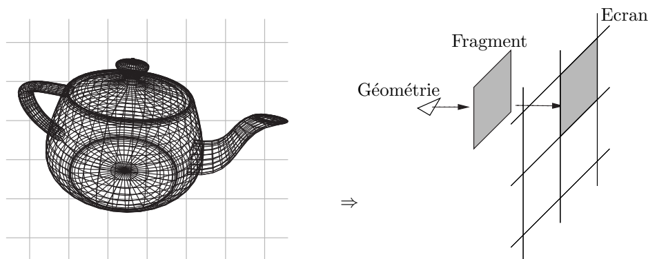
FIG. 2.5 – Exemple classique de rendu provoquant de sévères problèmes d' aliasing . La scène est sur-échantillonnée et la taille des triangles est bien inférieure à celle des pixels. Le fragment généré pour un triangle sera sur-dimensionné et ne sera pas un bon représentant du pixel.
