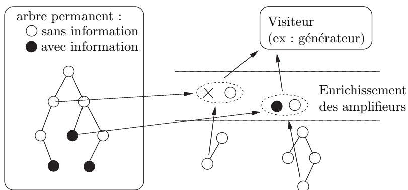
FIG. 6.11 – Avant d'être traité par le visiteur, l'amplifieur est enrichi de ses informations permanentes (si celles-ci existent).
