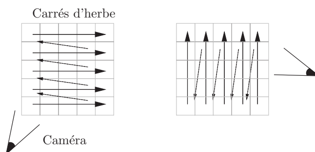
FIG. 4.5 – Dans le cas simple d’une répartition sur une grille régulière (comme c’est le cas du modèle de la prairie), un tri peut être effectué en temps linéaire.
