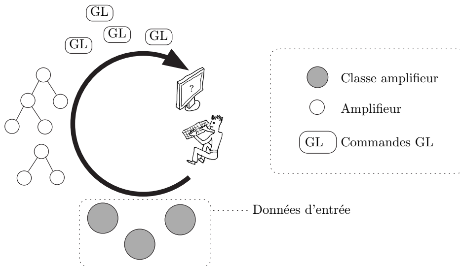
FIG. 5.2 – La nature du langage descriptif varie au fil de l'évaluation. Le langage descriptif initial est une sorte de C++ spécialisé pour la description de générateurs d'amplifieurs. Au fil de l'évaluation, ces classes génèrent des instances de classes, des commandes OpenGL et enfin des pixels sur l'écran.
