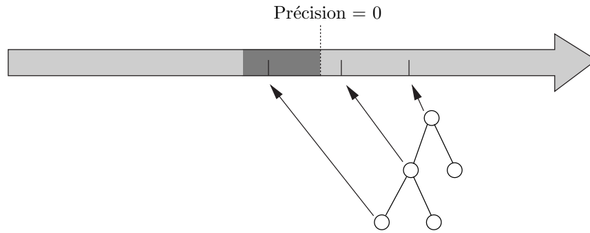
FIG. 6.16 – Les amplifieurs génèrent des fils tant qu'ils n'atteignent pas la première précision négative.
