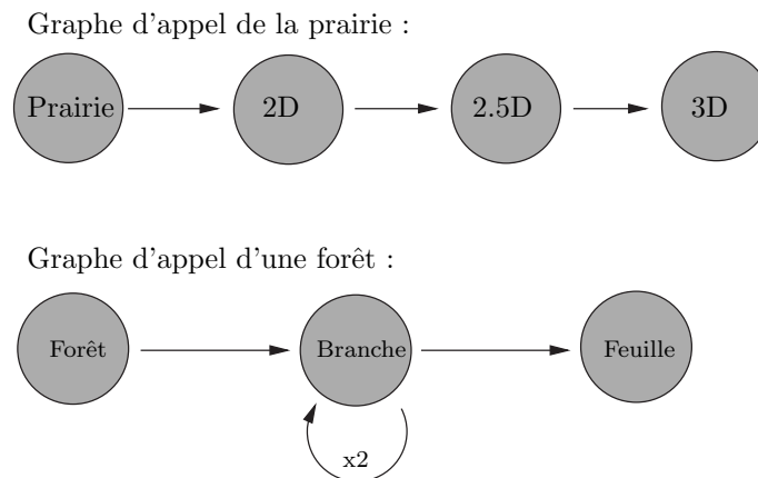
FIG. 5.4 – Les générateurs d’amplifieurs s’appellent les uns les autres. De fait, Dynamic Graph permet une représentation très concise des structures répétitives. Par exemple, le générateur de branche, en s’appellant lui-même, permet de décrire un arbre très succinctement en utilisant sa structure “pseudo-fractale”.
