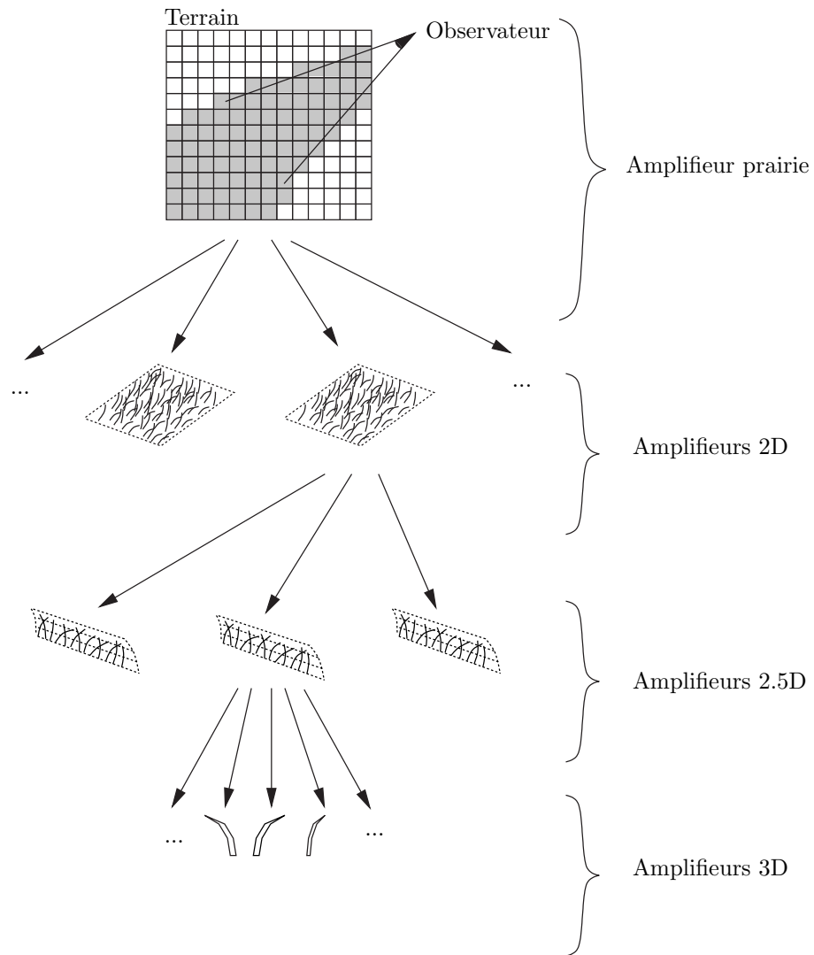
FIG. 5.1 – Un premier amplifieur “prairie” engendre les amplifieurs 2D à condition que ceux-ci soient dans le champ de vue. Ensuite, en fonction de la précision, les amplifieurs vont continuer leur ajout de précision (leur amplification) ou bien dessiner la forme qu’ils représentent.
