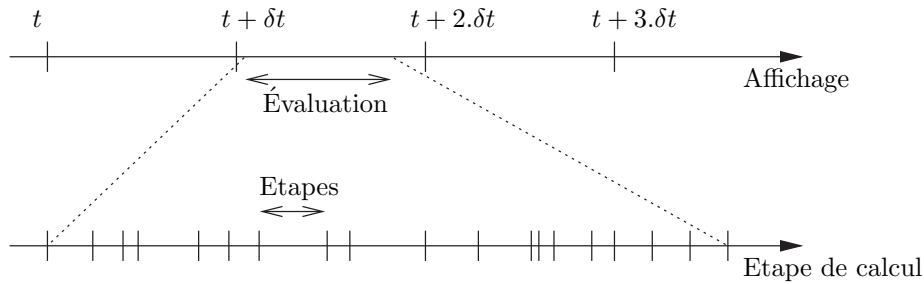
FIG. 6.1 – On appelle pas de temps les dates auxquelles une nouvelle observation est calculée. Chaque affichage est le fruit d’une évaluation, laquelle est divisée en étapes par l’organiseur.
