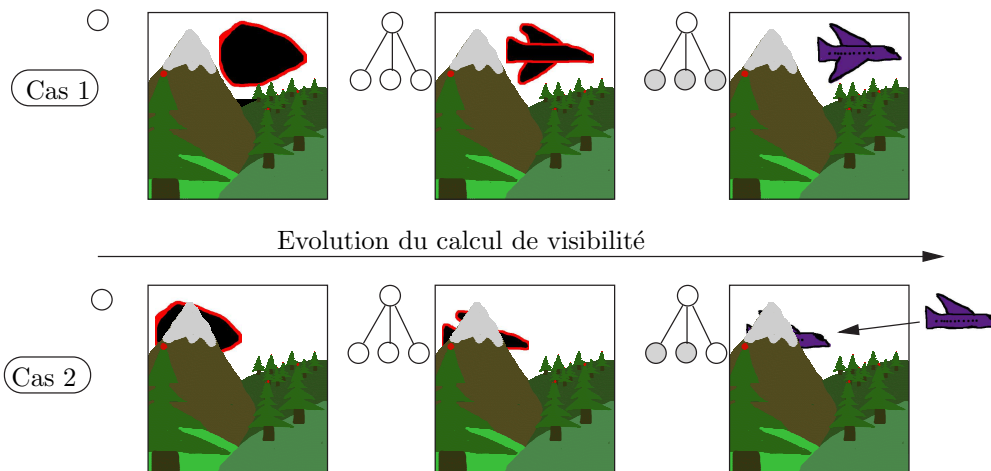
FIG. 6.22 – Les tests de visibilité s'effectuent sur une scène déjà partiellement dessinée. Avant de continuer l'amplification d'un objet, on teste la visibilité de sa boîte englobante. Si celle-ci est visible, l'amplification continue, sinon elle s'arrête. Lorsque la précision d'un amplifieur visible est suffisante, celui-ci est affiché.
