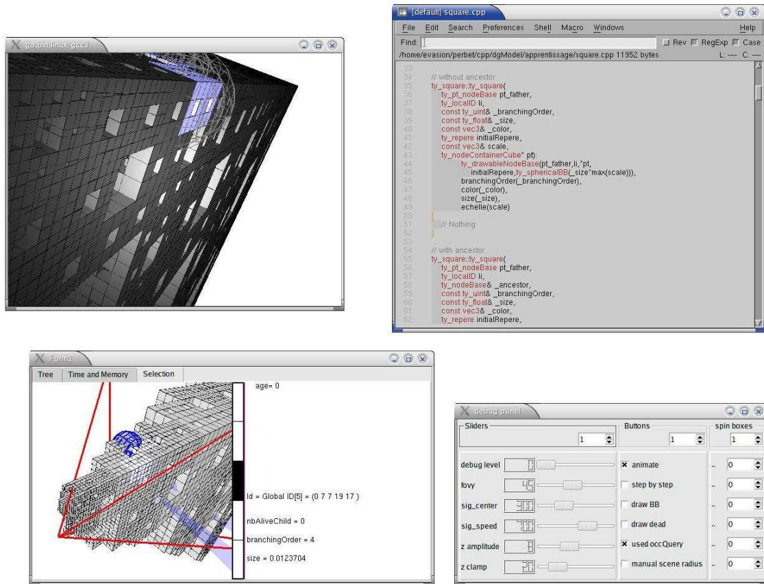
FIG. 7.5 – Exemple typique de modélisation avec Dynamic Graph. En haut à gauche, la fenêtre affiche l'objet tel qu'il est vu par l'observateur principal. En bas à gauche, une seconde observation permet de contrôler la manière dont le modèle s'adapte au point de vue; la sélection permet d'accéder aux micro-interfaces graphiques. En bas à droite, le debugPanel permet de changer dynamiquement certaines valeurs. En haut à droite, un éditeur de texte permet la modélisation des amplifieurs.
