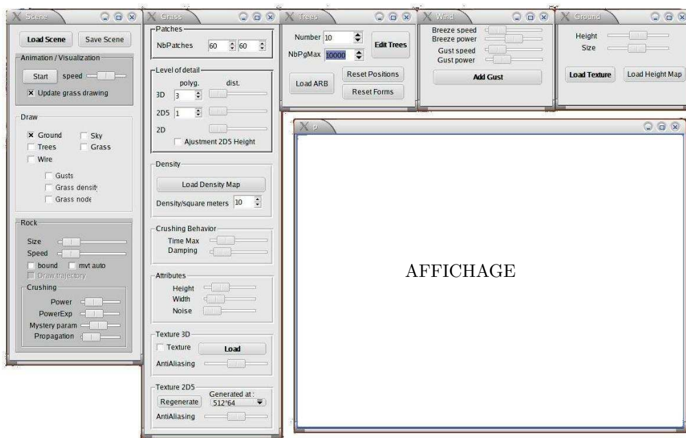
FIG. 4.25 – L'interface graphique de la seconde édition de la prairie permet de régler de très nombreux paramètres : densité de l'herbe, déclenchement des transitions, contrôle des fonctions d'animation.
