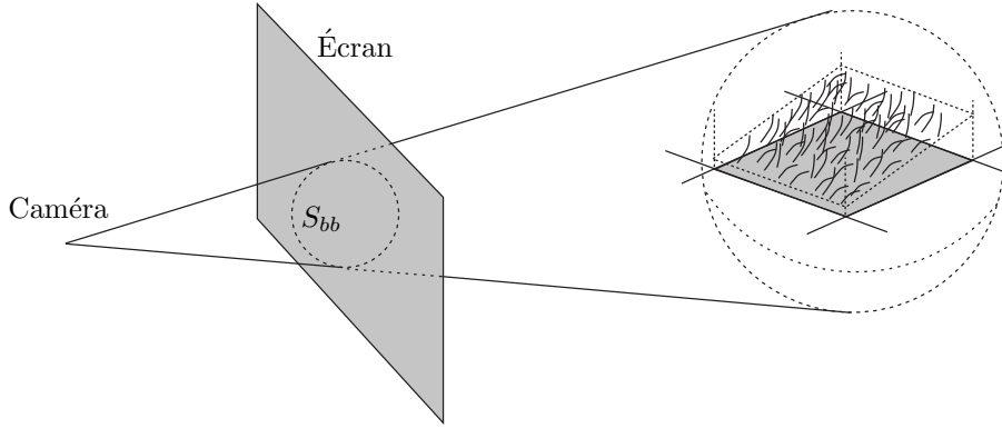
FIG. 6.15 – L’aire projetée S_{bb} de la boîte englobante d’un objet donne une idée approximative de la taille qu’il occupe sur l’écran. En diminuant le coefficient C_{créateur} , on peut prendre en compte le fait que l’objet a beaucoup de polygones (ou qu’il est texturé avec une image de grande résolution). Dans le cas de l’amplifieur 2D de la prairie, la valeur C_{créateur} est petite car le polygone est texturé (ce qui, visuellement, est équivalent à une subdivision plus fine du polygone).
