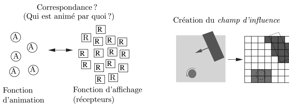
FIG. 4.13 – Chaque récepteur peut être animée ou non par des fonctions d'animation (bourrasque, tornade). Il est donc nécessaire d'établir une mise en correspondance coûteuse. Un calcul d'intersection entre chaque carré d'herbe et les masques d'influences permet de diminuer ce coût.
