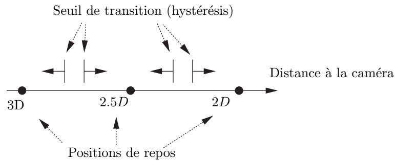
FIG. 4.10 – Les transitions se déclenchent lorsque la distance de la caméra au carré d’herbe passe par certains seuils. Pour éviter les oscillations entre deux niveaux de détails, les seuils sont différents selon le sens de la transition.
