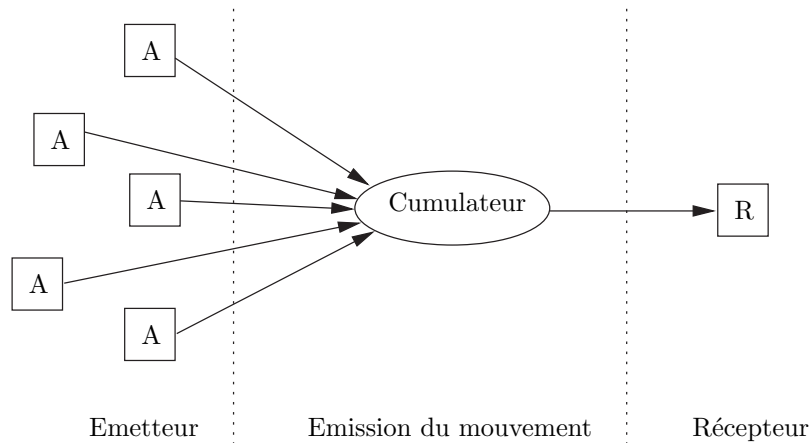
FIG. 4.23 – Le cumulateur combine les différentes influences des fonctions d'animation appliquées à un récepteur. Par défaut, il propose de pondérer les influences aux moyens de simples coefficients.
