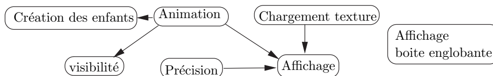
FIG. 6.5 – Au contact d’un visiteur, un amplificateur peut exécuter différentes fonctions. Celle-ci dépendent les unes des autres. Par exemple, l’affichage ne peut être effectué qu’après le calcul de l’animation.
