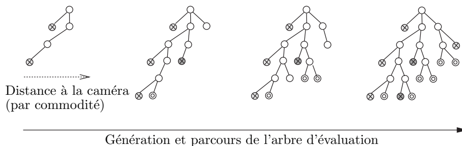
FIG. 5.9 – Un parcours trié en profondeur d'abord assure un rendu de l'avant vers l'arrière. Un noeud envoie ses commandes OpenGL dès que possible. Les feuilles visibles représentées par deux cercles imbriqués sont les amplifieurs les plus susceptibles de s'afficher. Sur ce schéma, par commodité de représentation, les amplifieurs à droite de l'arbre sont les plus distants de la caméra.
