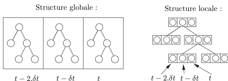
FIG. 6.12 – Pour que chaque noeud d’un graphe se souvienne de son ancêtre, deux structures sont possibles. La structure globale de Dynamic Graph stocke n arbres représentant les n dernières observations. La structure locale ne représente qu’un seul arbre, mais au sein de chaque noeud, n amplifieurs sont stockés (représentant les n dernières observations).
