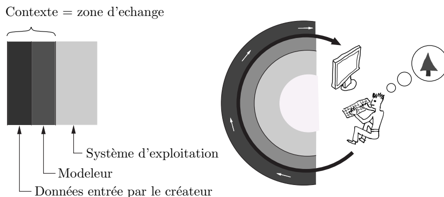
FIG. 3.2 – Durant le processus de création, un programme traite les idées du créateur ( les données d'entrée ) et les transforme en pixels. On peut considérer que tout le système d'exploitation fait partie du programme, mais cela n'a que peu d'influence : on se focalise sur, le contexte, c'est à dire la frontière entre l'outil et les données entrées par l'utilisateur.
