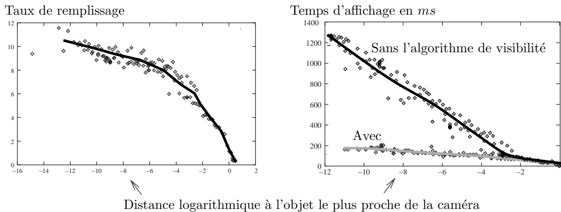
FIG. 6.27 – Les mesures sont effectuées en fonction de l'échelle d'observation (plus précisément, en fonction de la distance à l'objet le plus proche). Le modèle utilisé est le cube de Sirpienski. À gauche, la courbe représente le taux de remplissage engendrée par les boîtes englobantes uniquement . À droite, des mesure du frame-rate avec et sans l'algorithme de visibilité ont été effectuées.
