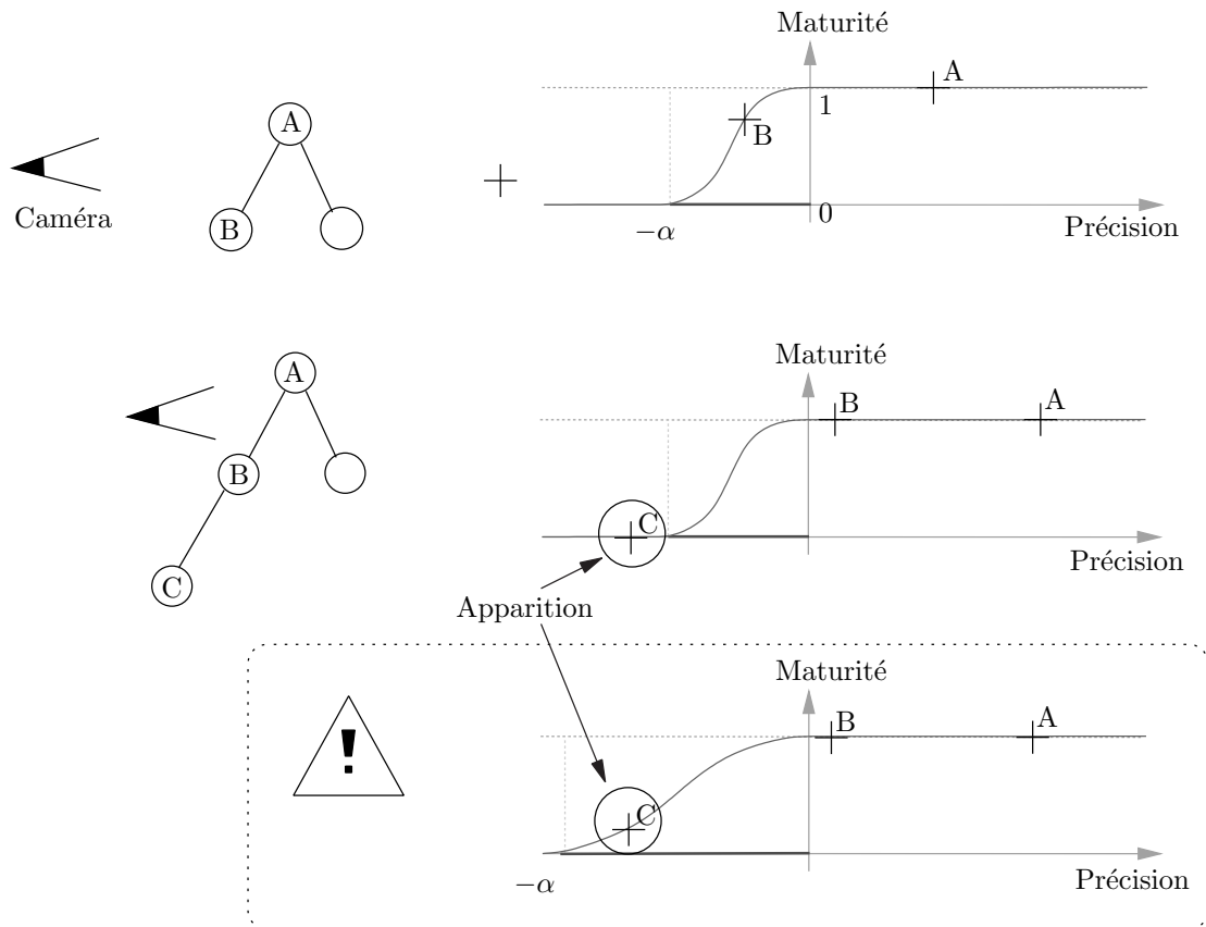
FIG. 6.18 – Lorsque la caméra se rapproche, un nouvel amplifieur naît. Si tout se passe bien, la précision de celui-ci sera suffisamment faible pour que sa maturité soit nulle. En conséquent, l’ajout de détail est initialement indiscernable. Mais si \alpha est mal réglé par le créateur, un amplifieur peut naître avec une maturité non nulle, ce qui engendrera un ajout soudain de précision.
