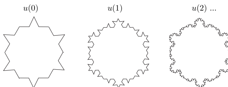
FIG. 3.5 – La construction de certaines fractales peut être vue comme un ajout successif de précision.
