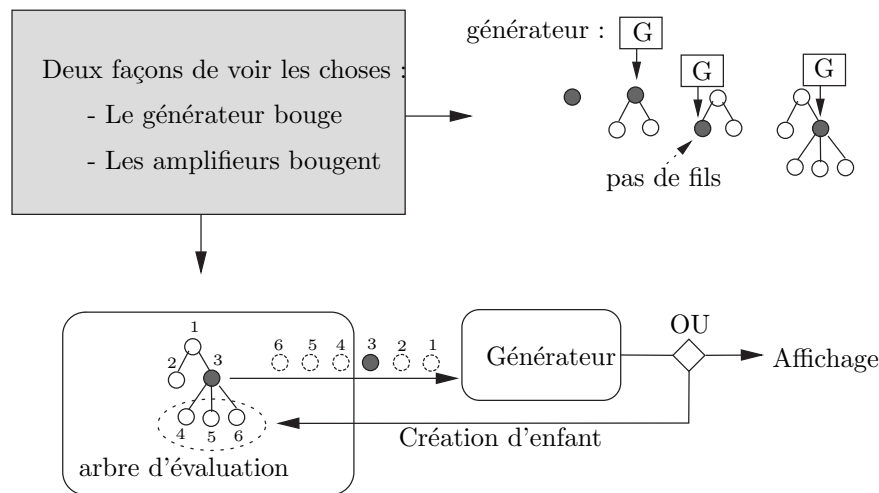
FIG. 6.2 – Il est plus facile de rendre compte de l’architecture en pipe-line lorsque ce sont les noeuds (les amplifieurs) qui bougent. Attention, ceci n’est qu’une vue de l’esprit. Concrètement, ni le visiteur ni les noeuds ne changent de place en mémoire.
