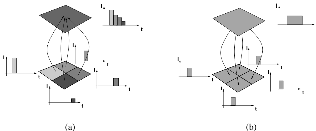
Figure 9.5 - Représentation hiérarchique de la radiosité temporelle. (a) Un écho peut être représenté à un niveau supérieur de détail par quatre échos de même temps de propagation et intensité. (b) Lorsqu'ils sont utilisés à un niveau de détail moindre, la distribution temporelle des échos est maintenue alors que leurs intensités est pondérée au prorata des rapports d'aires « fils/père ».
