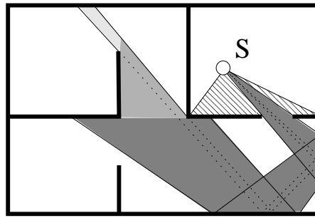
Figure 3.5 - Réflexion et fenêtrage des faisceaux générés depuis la source (S) 4 .
