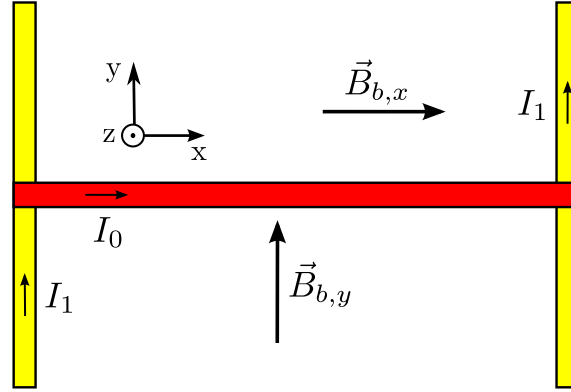
FIG. 2.4 – Piège Ioffe-Pritchard en « H ». Deux fils parallèles parcourus par des courants égaux croisent les extrémités du fil qui génère le confinement transverse. Combinés au champ B_{b,x} , ils assurent le confinement selon l'axe x .
