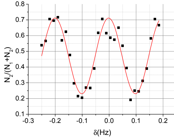
FIG. 5.13 – Spectroscopie Ramsey effectuée avec une durée d'interrogation de Ramsey de 5 s, conduisant à une largeur à mi-hauteur de 100 mHz, conduisant à un facteur de qualité \nu_0/\Delta\nu = 7 \times 10^{10} . Le contraste des franges est de 51%, réduit par la température élevée des atomes par rapport à la mesure présentée figure 5.10. La durée de cycle de 14,7s. En rouge : ajustement des données par une courbe suivant l'équation 5.5. Le rapport signal à bruit est de 8, conduisant à une stabilité à une seconde de 4 \times 10^{-12} .
