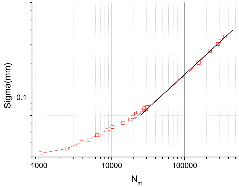
FIG. 4.8 – Taille du nuage en fonction du nombre d'atomes, en échelle log-log. \text{Log}[\text{Sigma}] est proportionnel à \text{log}[T] . Chaque point correspond à une fréquence finale différente pour l'évaporation, allant de 8 à 3,855 MHz de droite à gauche. Le courant dans le dispenser est de 3,8 A. La droite noire correspond à une régression linéaire effectuée sur les 6 premiers points.
