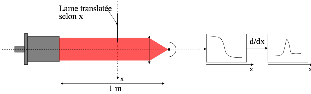
FIG. 3.12 – Mesure de la divergence du faisceau. On mesure le profil du faisceau à différentes distances, afin d'en extraire son diamètre. On en tire la divergence du faisceau, qui est ici de 0,6 \text{ mrad} \pm 0,6 \text{ mrad}
