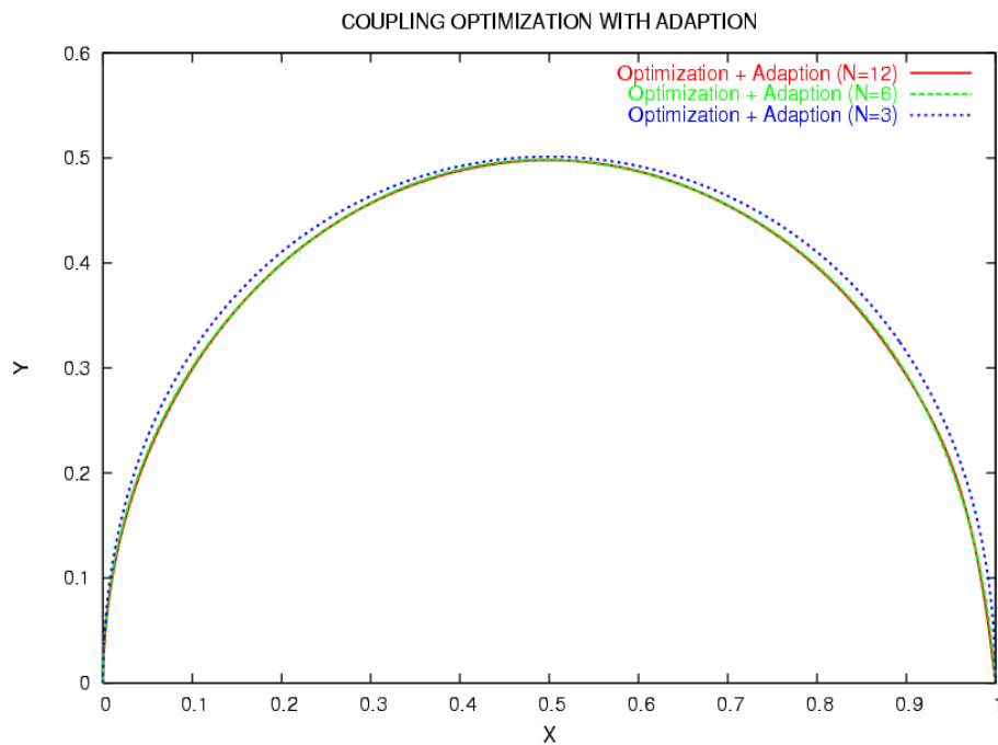
FIGURE 5.6 – Couplage optimisation-adaptation : pour N=3, 6 et 12, et avec une stratégie hiérarchique (N=3->6->12)
