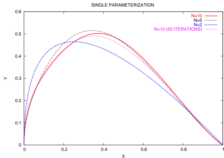
FIGURE 4.8 – Formes optimales obtenues pour n = 2, 5 et 10
