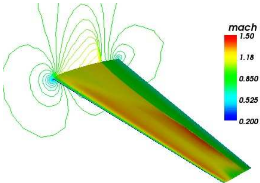
FIGURE 4.23 – Champs et isovaleurs de nombre de Mach : configuration initiale
