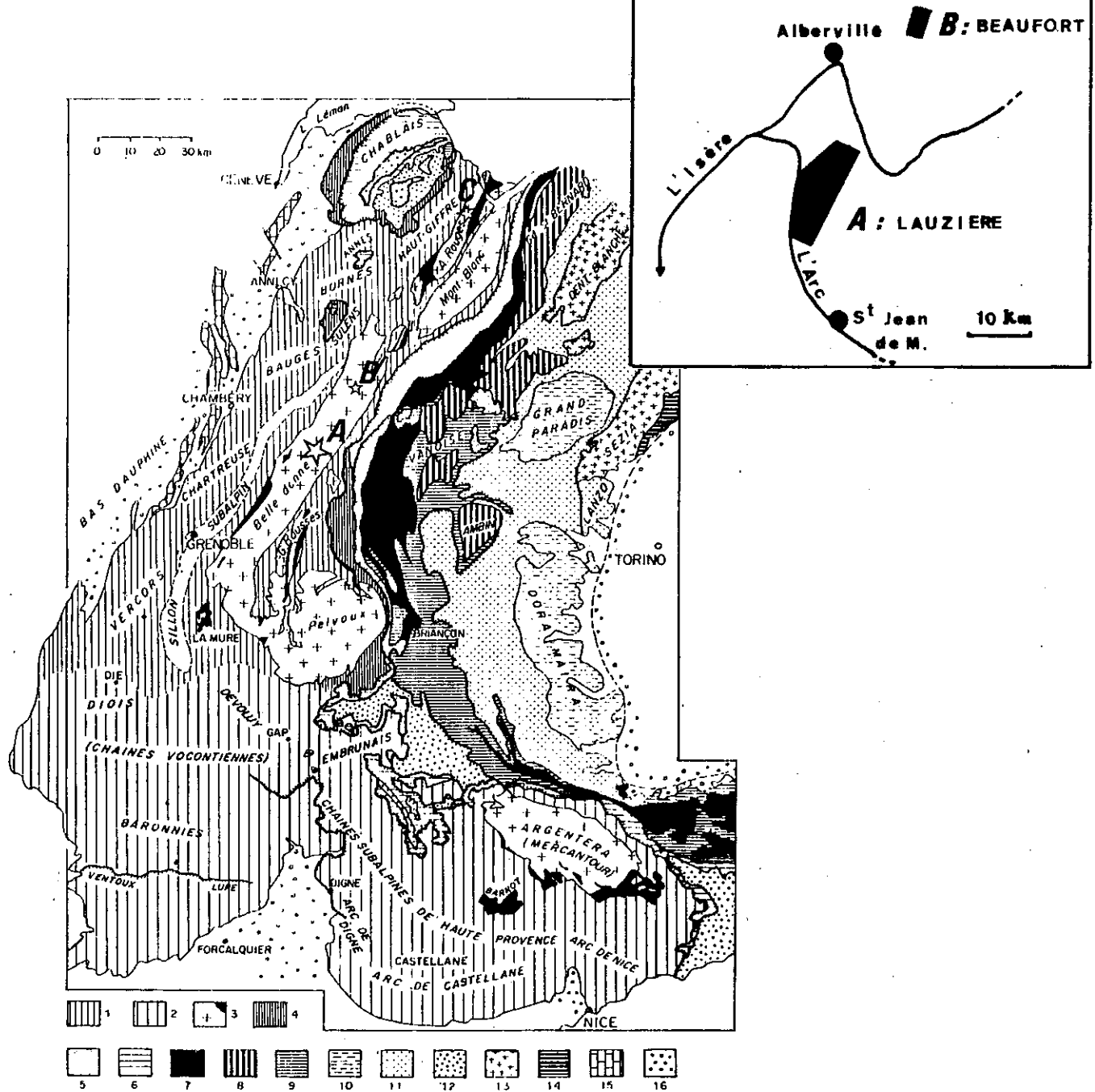
Schéma structural simplifié des Alpes franco-italiennes.
