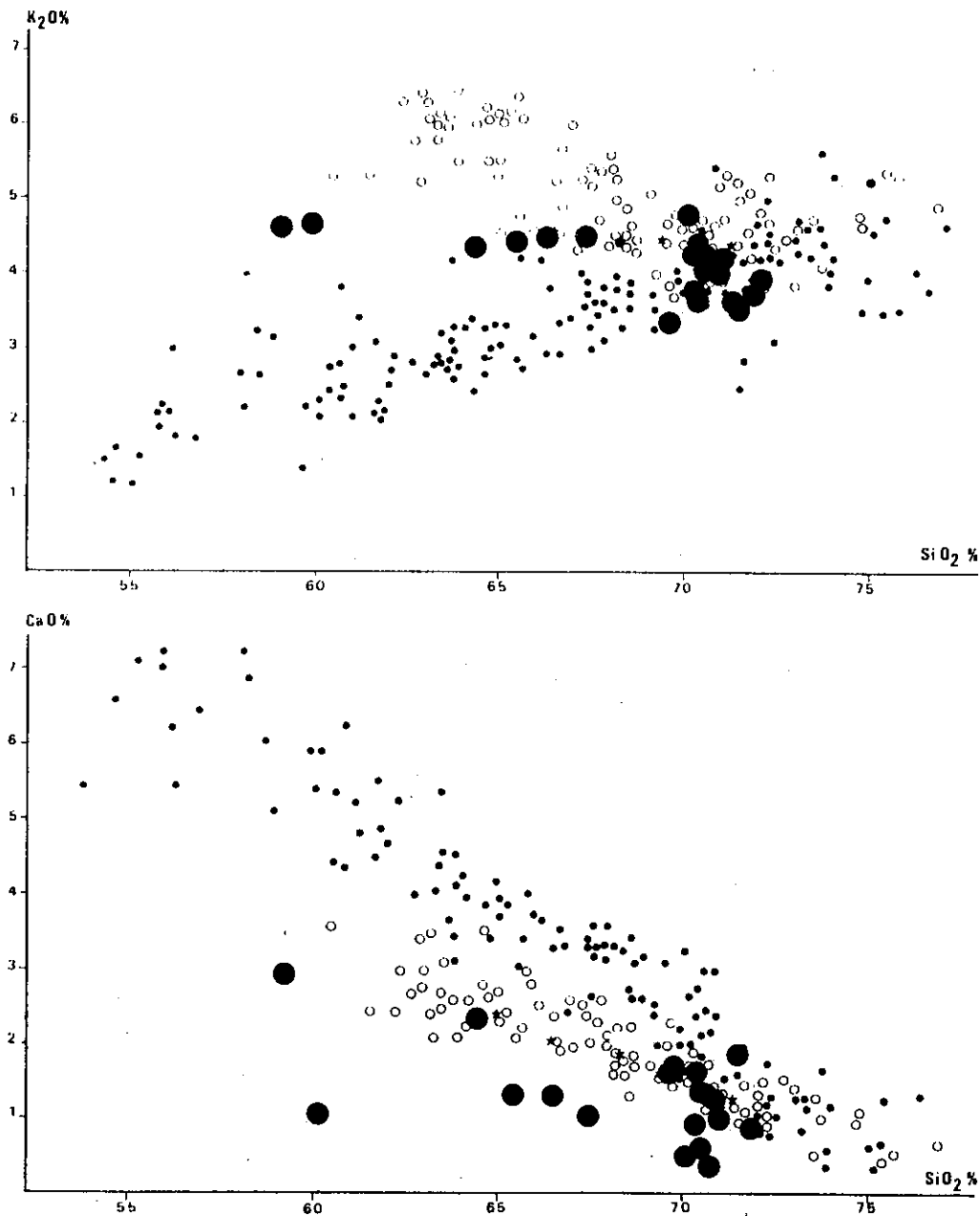
Diagrammes montrant l'évolution des teneurs en CaO et K_2O par rapport à SiO_2 dans l'association calco-alkaline (cercles noirs) et les associations sub-alkalines (cercles blancs, type Balagne; étoiles, type Margeride).
