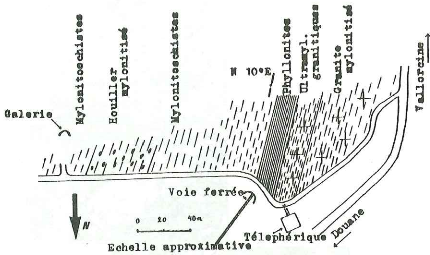
Schéma géologique de la plateforme EDF du Châtelard
