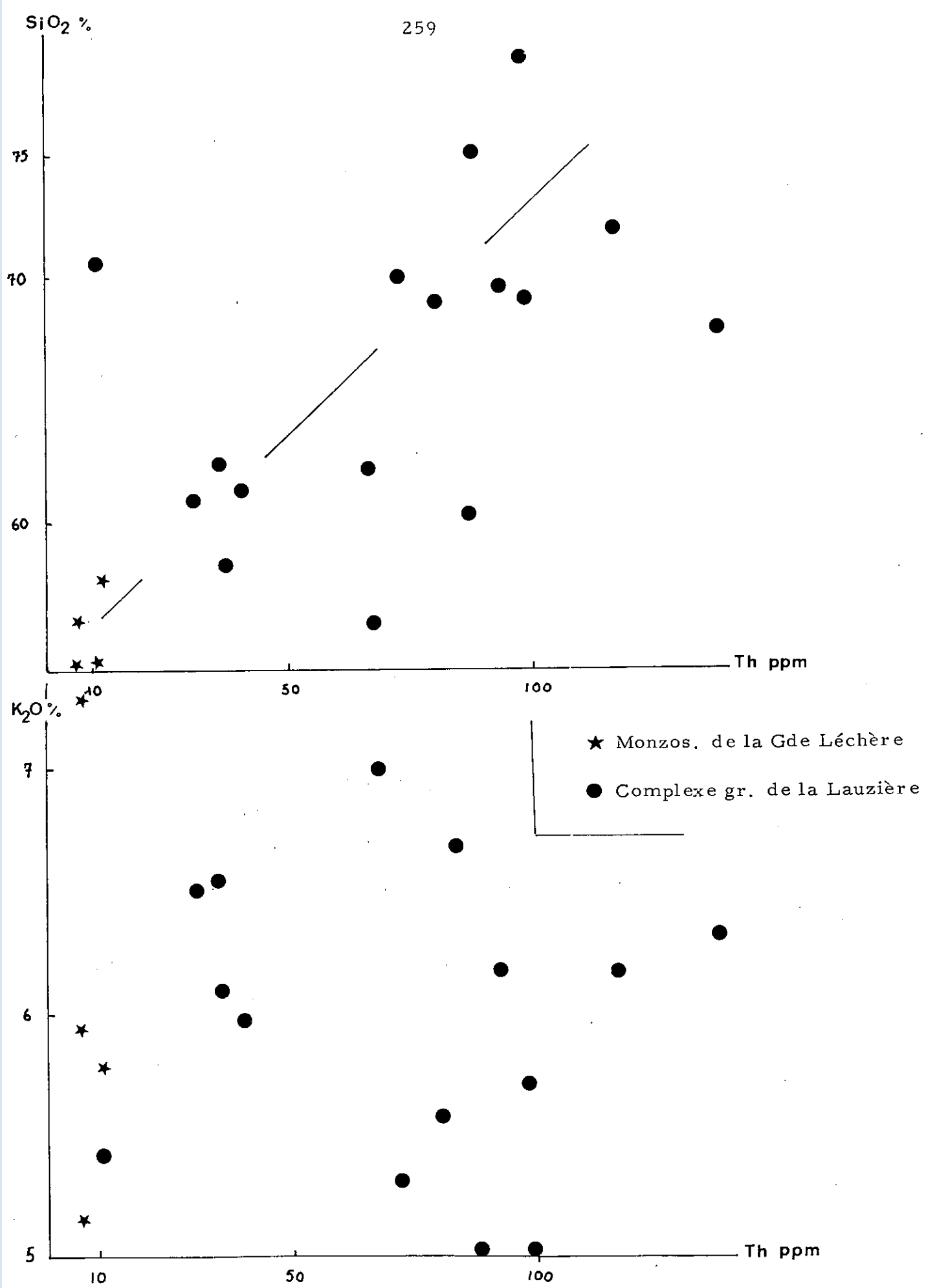
Figure 107 : corrélations Th - SiO 2 , K 2 O, Fe 2 O 3 dans le complexe granitoïde de la Lauzière et les monzos. du Lac de la Grande Léchère
