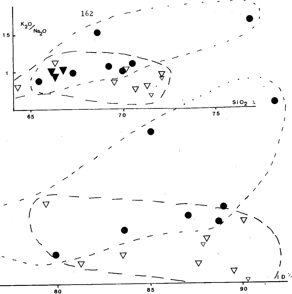
Figure 65 : granodiorites du Colombran et leptynites du complexe du Col de Montjoie; évolution du rapport K_2O/Na_2O en fonction de la différenciation (diagr. K_2O/Na_2O - SiO_2 , I. D., Fe_2O_3/MgO ) (Lég. id. fig 64)
