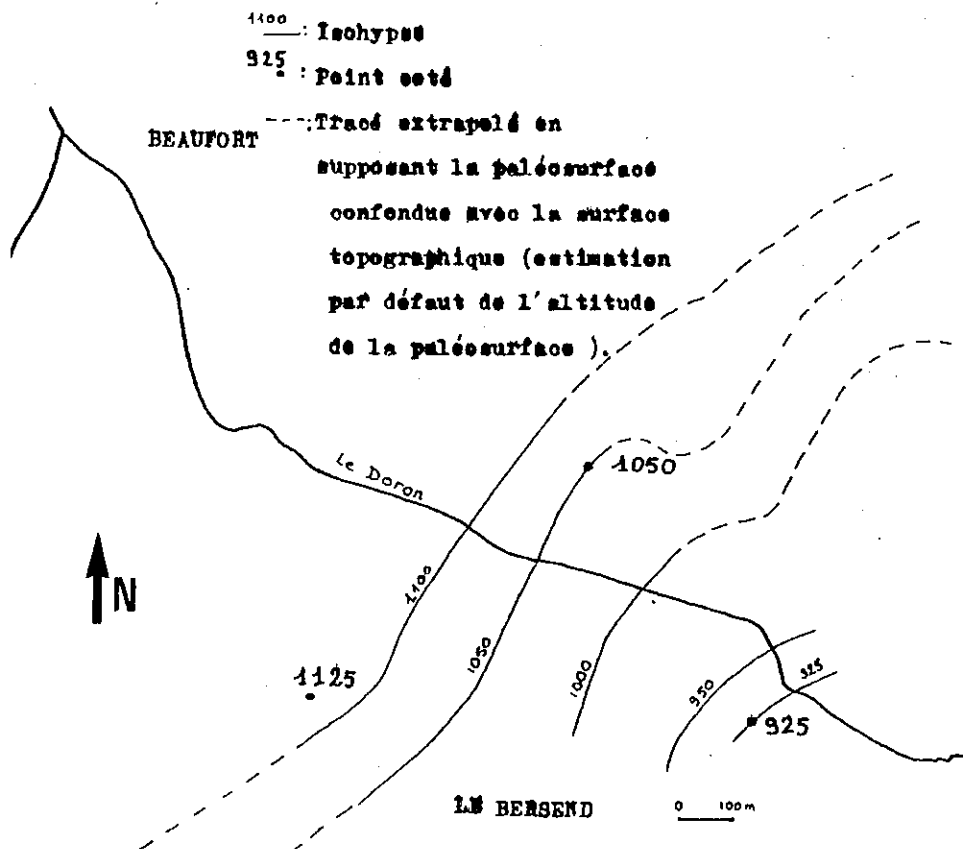
Figure 35 - Carte hypsométrique de la paléosurface du granite de Beaufort
