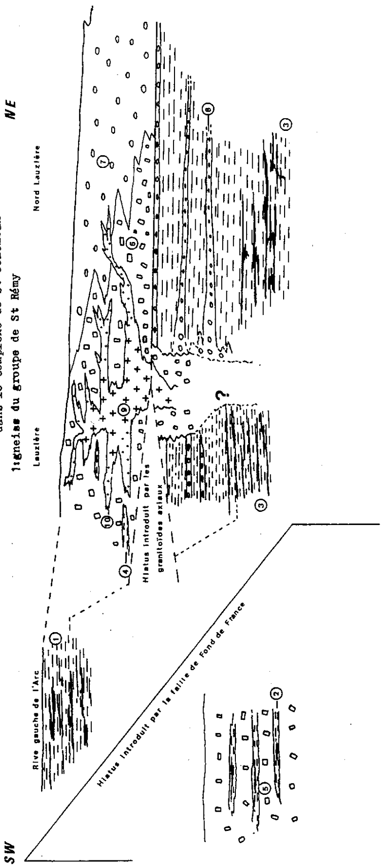
Figure 97 : coupe schématique illustrant les relations entre les séries anciennes avant l'évènement tectonométamorphique principal les ayant affectées
