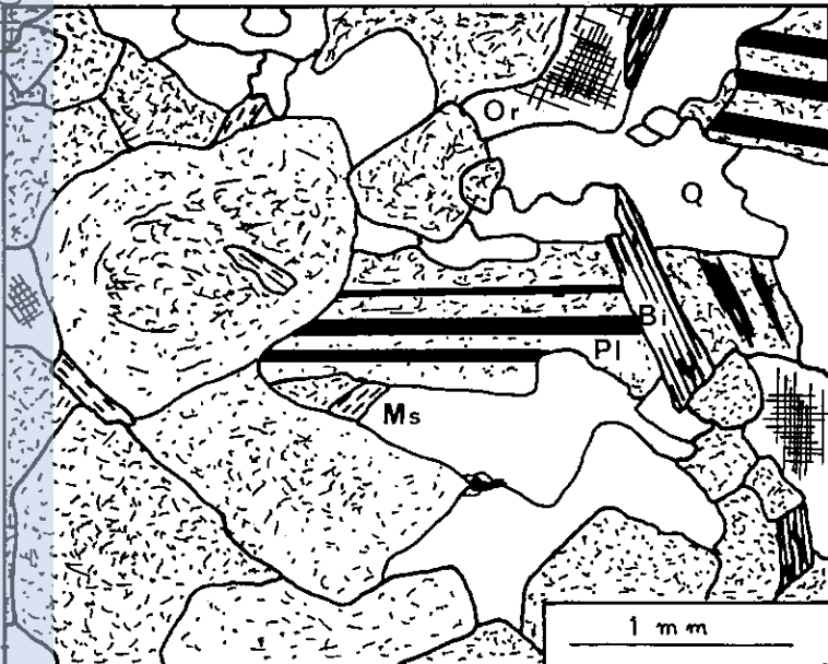
Figure 52 : granodiorites du Colomban
