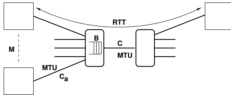
FIG. 2.5 – Network parameters
