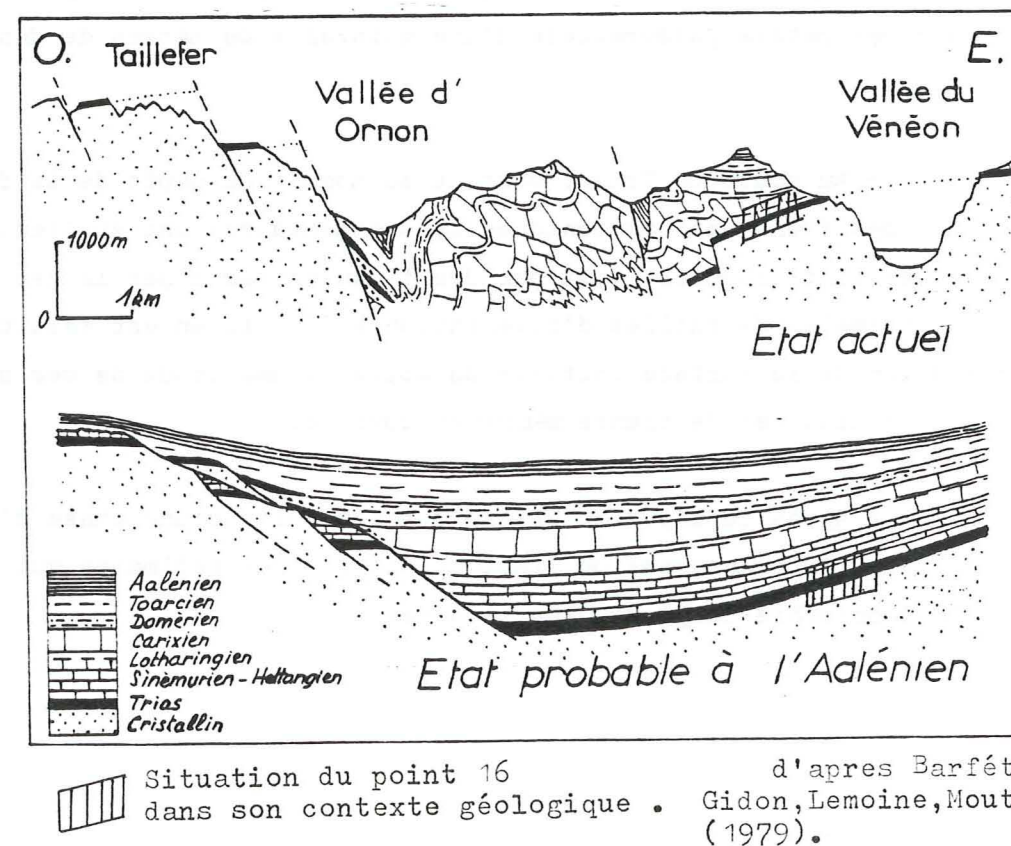
Fig. 5.14. Accident du col d'Ornon
