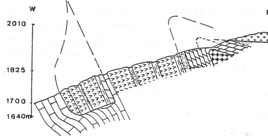
Fig. 4-10. Le redoublement de la série triasique expliqué par la présence d'un olistolithe
