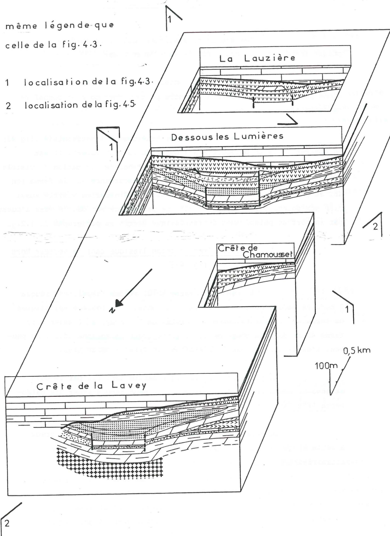
Fig.4.7. Bloc diagramme restitué du secteur de l'Esparcelet au début du Sinémurien.
