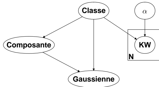
FIGURE 7.3 – Modèle de mélange GM-Mult
