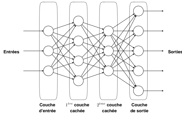
FIGURE 3.3 – Exemple d'un perceptron multicouches
