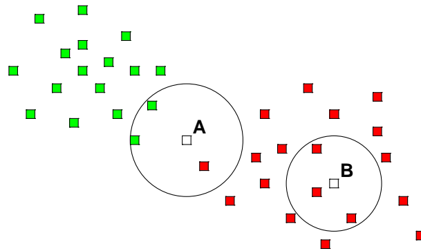
FIGURE 3.2 – Exemple de classification biclasses avec un kppv où k = 3
