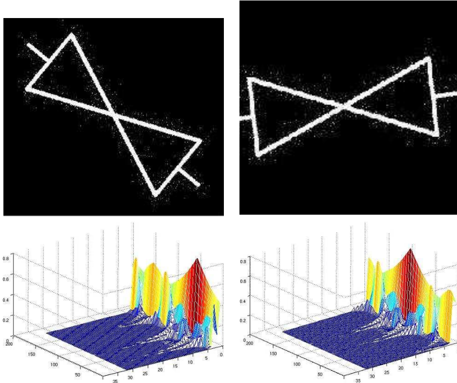
FIGURE 6.1 – Le descripteur HRT face à la rotation
