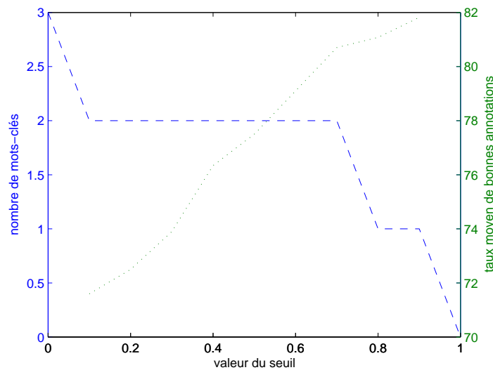
FIGURE 7.7 – Taux moyen de bonnes annotations et nombre moyen de mots-clés obtenus en fonction de la valeur du seuil
