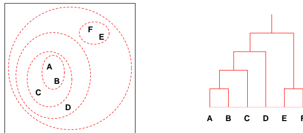
FIGURE 3.6 – Exemple de classification hiérarchique
