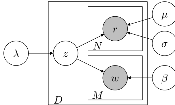
FIGURE 4.8 – Modèle GM-Mixture
