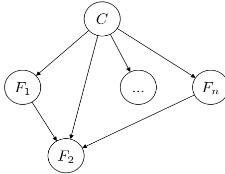
FIGURE 5.6 – Réseau Bayésien naïf augmenté
