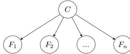
FIGURE 5.5 – Classificateur Bayésien naïf
