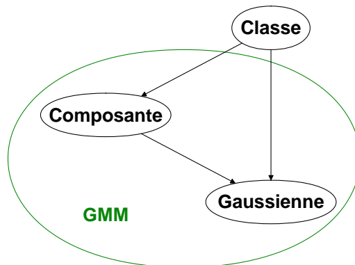
FIGURE 7.2 – GMMs représentés par un modèle graphique probabiliste
