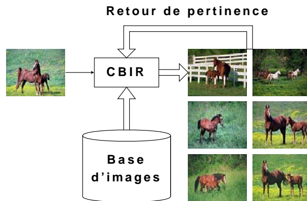
FIGURE 2.6 – Bouclage de pertinence dans un système de CBIR
