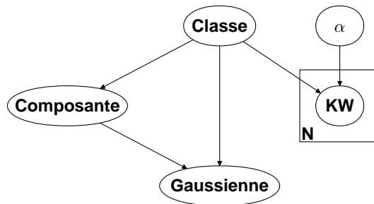
FIGURE 7.4 – Modèle de mélange de lois de Bernoulli et de mélanges de Gaussiennes, pour la combinaison de caractéristiques visuelles et sémantiques
