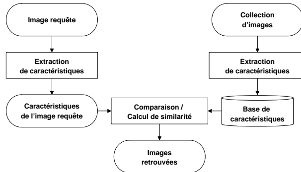
FIGURE 2.5 – Système de recherche d'images par le contenu
