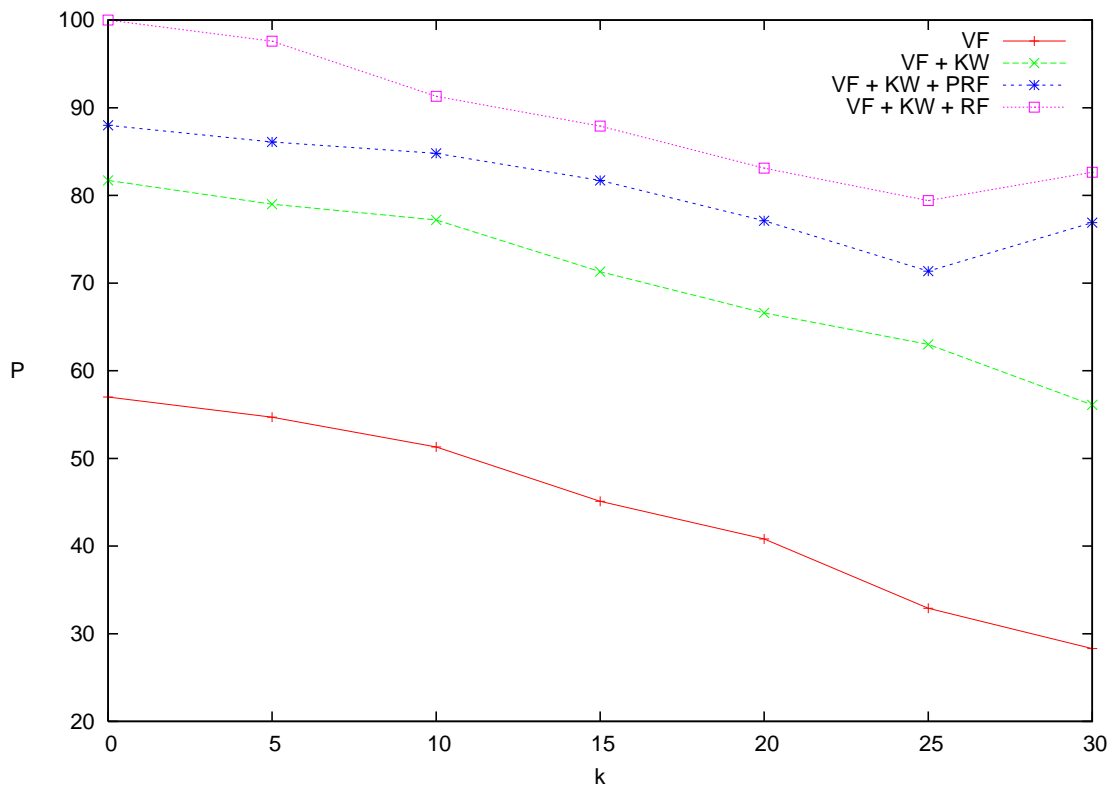
FIGURE 8.3 – Précision P en fonction du rang k
