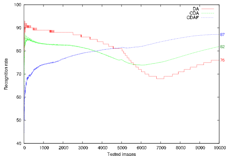
FIGURE 3.5 – Évolution du taux de reconnaissance de la CDA, avec ou sans retour de pertinence, comparée à la DA
