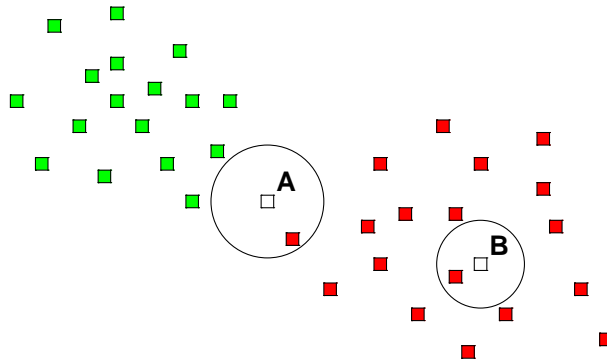
FIGURE 3.1 – Exemple de classification biclasses avec un kppv où k = 1
