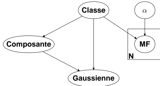
FIGURE 6.7 – Modèle de mélange de lois de Bernoulli et de mélanges de Gaussiennes, pour la combinaison de descripteurs
