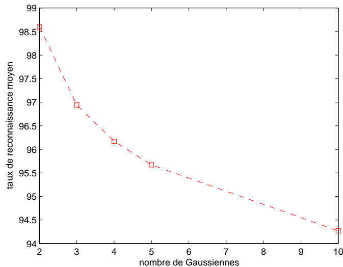
FIGURE 6.10 – Taux de reconnaissance moyen en fonction du nombre de Gaussiennes
