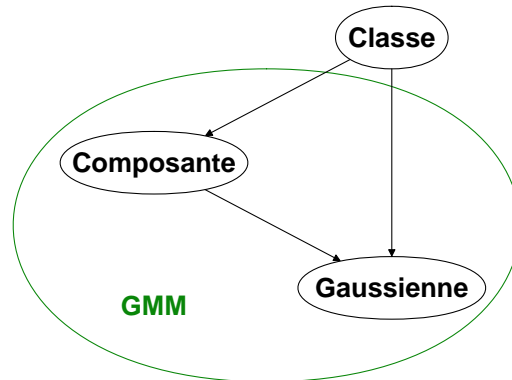
FIGURE 8.1 – GMMs représentés par un modèle graphique probabiliste
