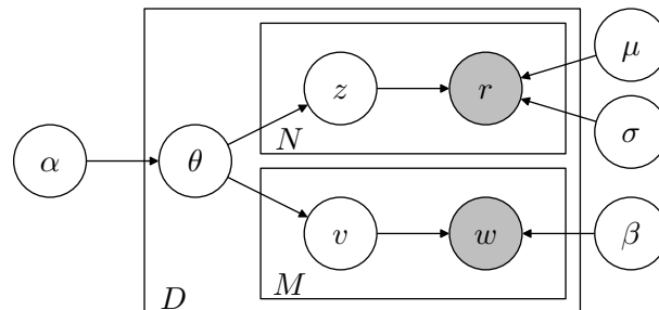
FIGURE 4.9 – Modèle GM-LDA
