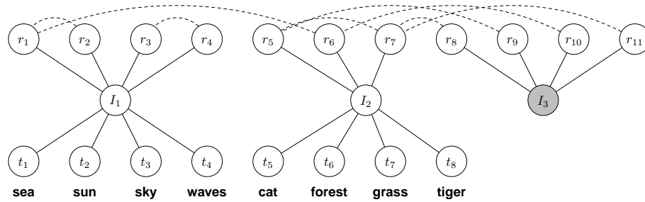
FIGURE 4.7 – Graphe « MMG »
