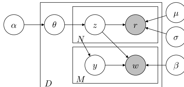
FIGURE 4.10 – Modèle Corr-LDA
