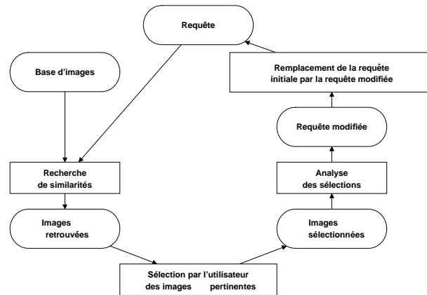
FIGURE 2.3 – Processus de base du retour de pertinence en recherche d'images
