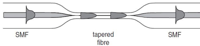
Figure I.46 : Schéma d'une fibre effilée.
