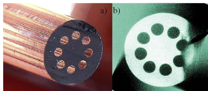
Figure I.34 : a) Photo d'une préforme de fluorure obtenue par extrusion puis perçage. b) Vue de coupe d'une fibre obtenue par cette méthode. [52]
