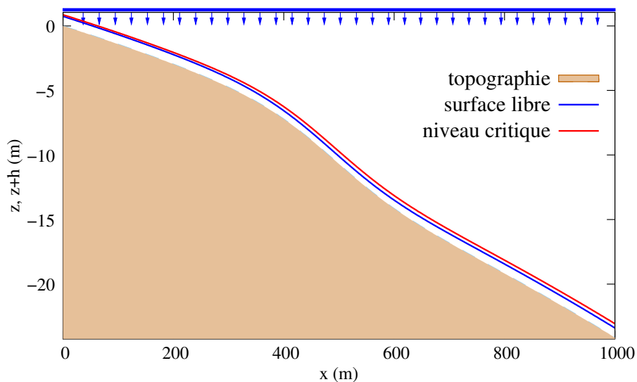
FIG. 5.7: Écoulement torrentiel-torrentiel avec de la pluie pour la loi de Darcy-Weisbach.
