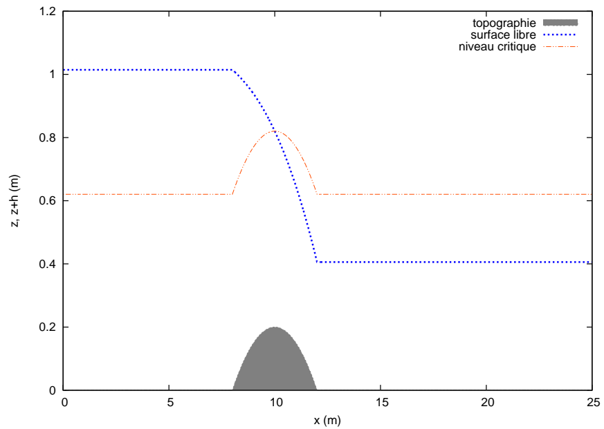
FIG. 2.5: Ecoulement transcritique à l'équilibre.
