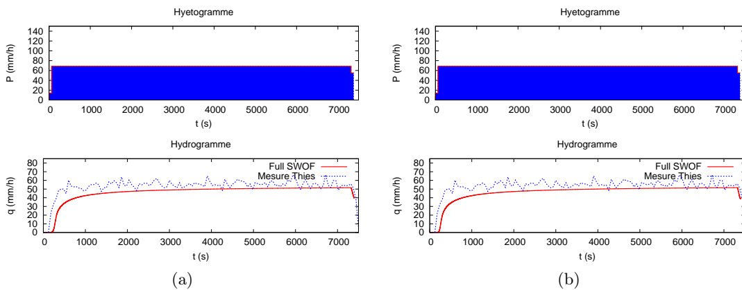
FIG. 6.20: Parcelle de Thies : hyétogramme et comparaison des hydrogrammes simulées et mesurées (a) pour f = 0.26 et (b) pour les coefficients de frottement hétérogènes.
