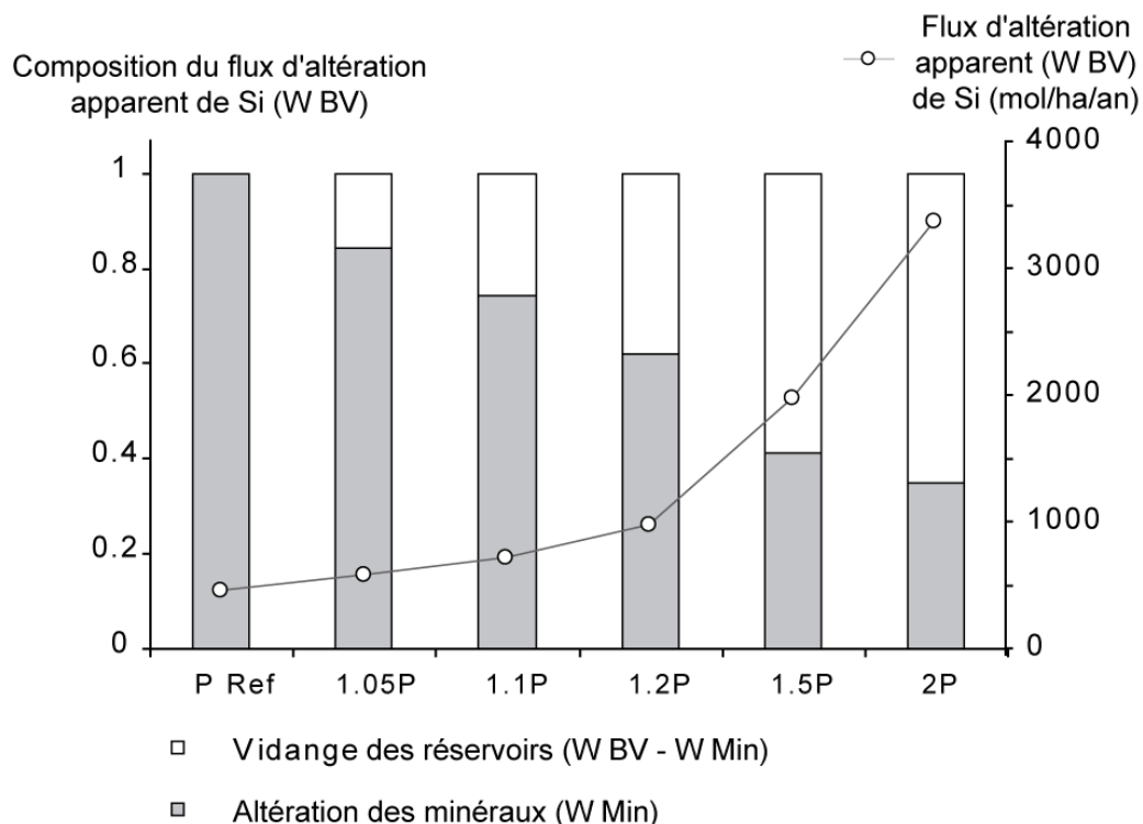
Figure II7.5 : Flux d'altération apparent à l'échelle du bassin versant de la silice pour les simulations « impact » et part correspondante de l'altération des minéraux et de la « vidange » des réservoirs. Les forçages climatiques des simulations « impacts » sont indiqués sur la figure. P Ref : simulation de référence à l'équilibre (Chapitre II-3). W BV : Bilan d'altération apparent à l'échelle du bassin versant (exports par le ruisseau et la nappe moins les intrants atmosphériques). W Min : Bilan d'altération des minéraux.
