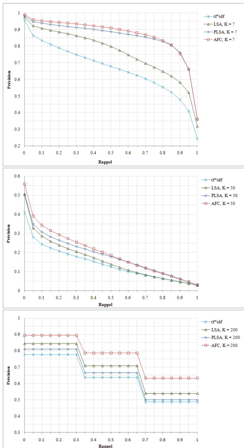
FIGURE 3.8 – Courbes de précision-rappel des différentes méthodes avec la similarité de cosinus pour les bases Caltech-4 (en haut), Caltech-101 (au milieu) et Nistér-Stewenius (en bas).
