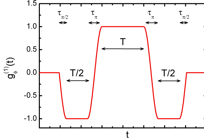
FIG. 2.6 – Fonction de sensibilité à la phase dans le domaine temporel pour un interféromètre à 4 impulsions de temps d'interaction total 2T=800 ms.
