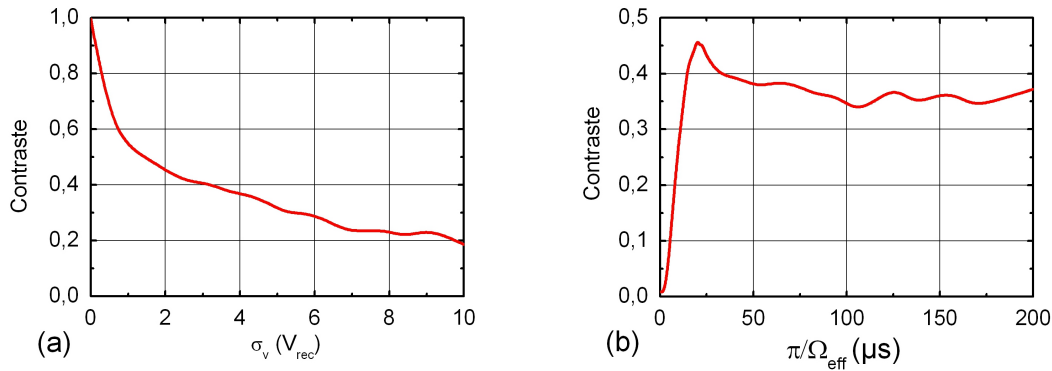
FIG. 4.15 – (a) Con contraste maximal de l'interféromètre, pour \Omega_{eff} = 5 \times 10^4 \text{ rad.s}^{-1} au centre du faisceau Raman, en fonction de la largeur de la distribution en vitesse initiale des atomes. (b) Con contraste de l'interféromètre en double-diffraction en fonction de \pi/\Omega_{eff} pour une distribution en vitesse initiale correspondant à celle de l'expérience.
