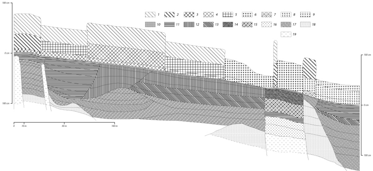
Figure 5.3 : Représentation du milieu naturel le long de la première toposéquence de Kamech (seuls les matériaux dominants dans chaque hoplexol sont représentés sur la coupe).
