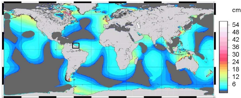
Figure C.5.2. Elévation du niveau moyen des pleines mers sous l'action du cycle nodal de marée à 18.6 ans d'ici 2015. Les zones grisées correspondent à des zones d'élévation limitées (ou de diminution). La zone encadrée (48W-62W-2N-12N) délimite le système sédimentaire du plateau des Guyanes. D'après Gratiot et al., 2008, adapté de Simon, 2007.
