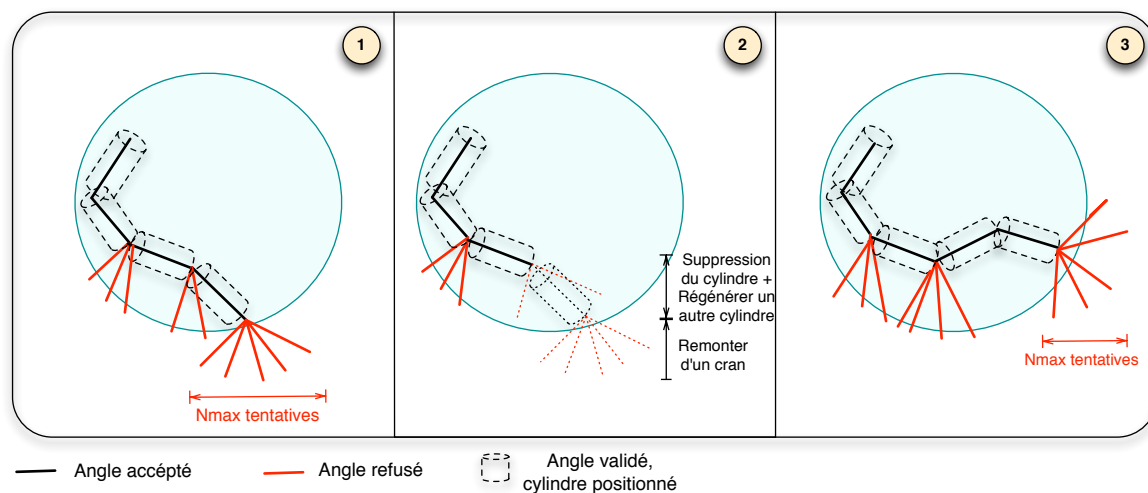
FIG. 3.14 – Etapes de la recherche d'une conformation spatiale de la molécule par l'algorithme de backtraking
