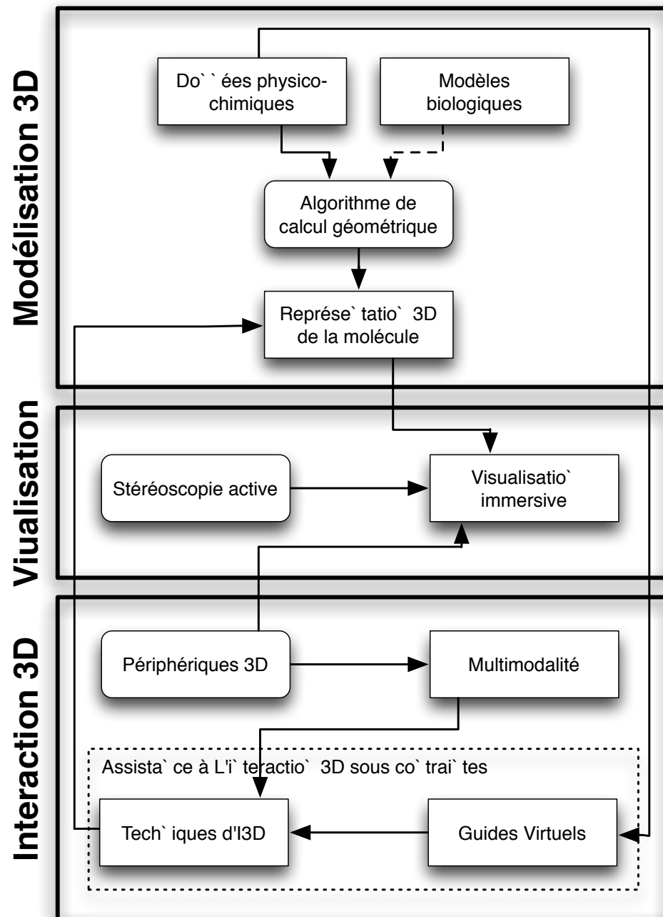
FIG. 5.6 – Schéma architectural du système d'analyse in virtuo : modélisation 3D, visualisation et interaction 3D du chromosome
