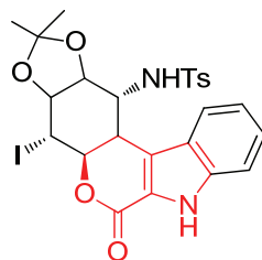
IV.1 (indolactone)
