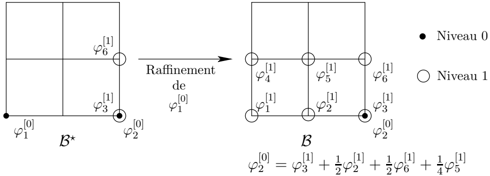
FIG. II.1 – Le raffinement ne préserve pas l'indépendance linéaire des ensembles multiniveaux ne satisfaisant pas (\mathcal{P}_{LI}) .
