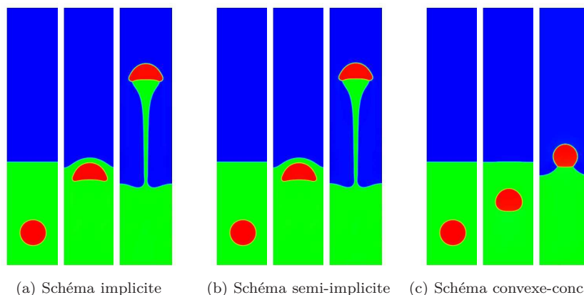
FIG. 8 – Comparaison des différents schémas sur une simulation de montée de bulle aux mêmes instants physiques.
