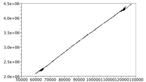
(b) en fonction du nombre total d'inconnues
