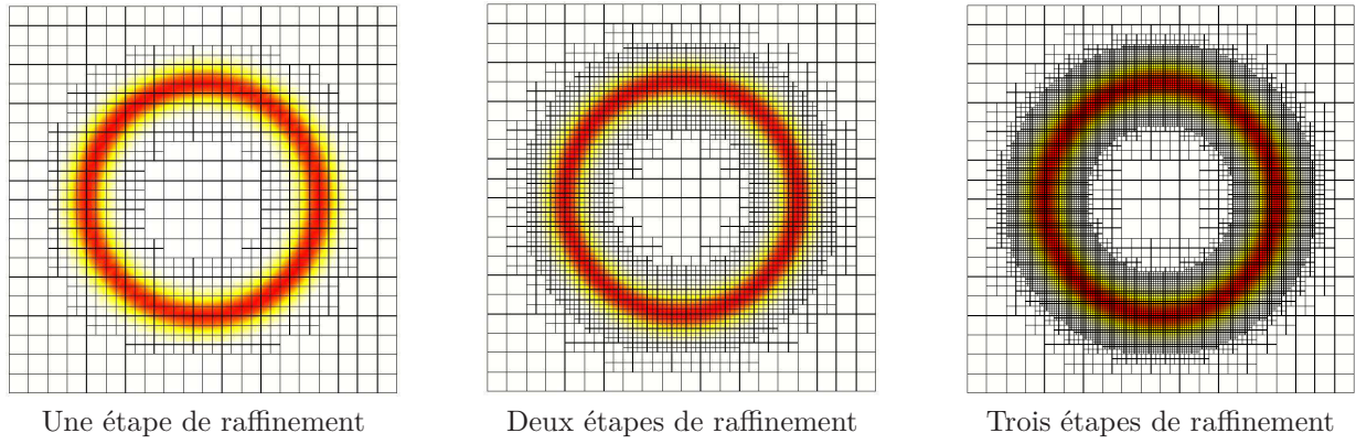
FIG. II.14 – Carrés- Q_1 . Maillages raffinés.
