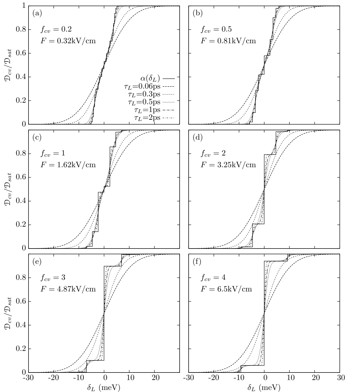
FIG. 2.10 – Absorption optique du super-réseau S2 ( \Delta_{cv} = 9.28 \text{ meV} , d = 14.3 \text{ nm} ) à différentes valeurs de \tau_L et champ effectifs f_{cv} . Sur les mêmes figures l'absorption due à une excitation continue \alpha(\delta_L) est présentée (traits pleins).
