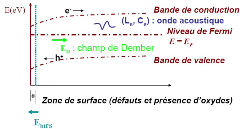
FIGURE 4.1 – Situation générale et existence du phénomène de pinning ; cas d'un semi-conducteur de type p ; description des champs électrique E_D et E_{bif/P}
