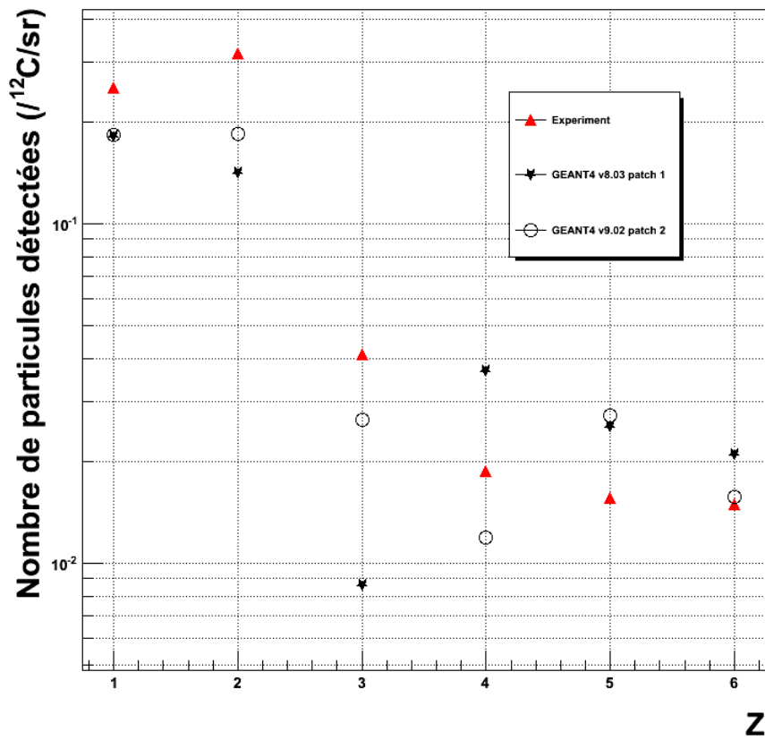
Figure 63 : comparaison des distributions en charge pour 1,5 cm de PMMA à 10°. Les résultats issus de la version 8.3 patch 1 sont représentés par une étoile, les résultats de la version 9.2 patch 2 avec un cercle creux et les résultats expérimentaux avec un triangle.
