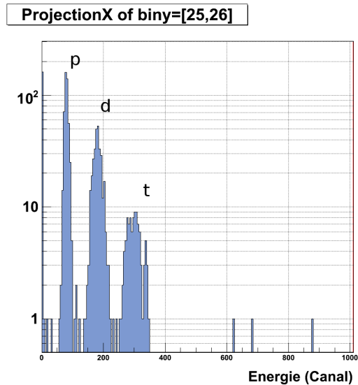
Figure 26 : spectre construit à partir de la projection suivant l'axe E (voir fig 25). Les trois pics représentent les isotopes de l'hydrogène.
