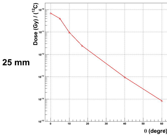
Figure 39 : évolution de la dose déposée dans le silicium en fonction de l'angle de détection pour les cibles de PMMA de 5, 10, 15, 20, 25 et 40 mm. Les valeurs de dose sont représentées par des triangles. Les traits guident l'œil.
