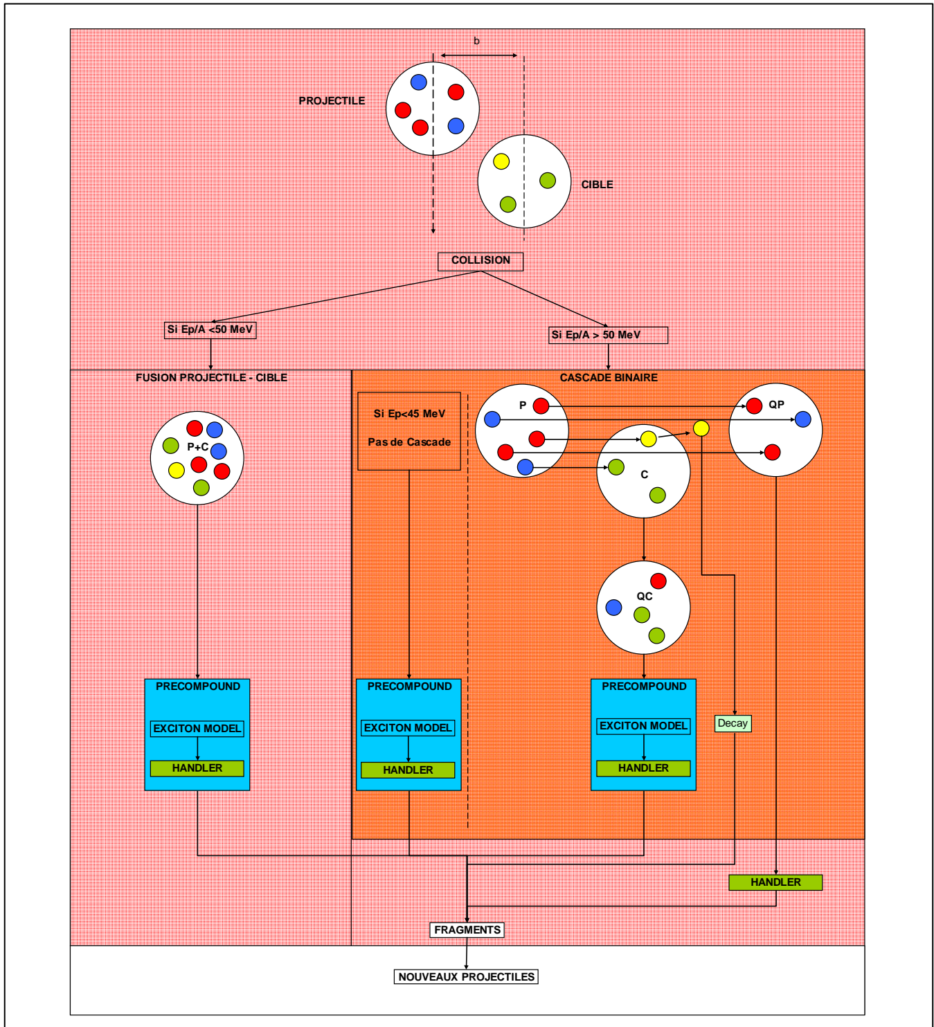
Figure 64 : schéma descriptif du traitement des collisions noyau-noyau par la classe G4BinaryLightIonReaction.
