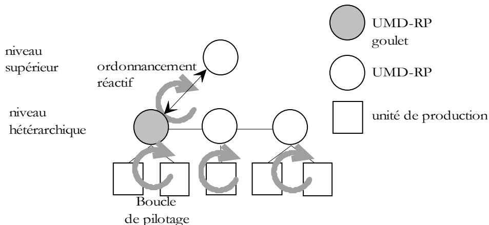
Figure 5. Agencement hétérarchique-supervisé (classe II) et pilotage de l'UMD-RP goulet.
