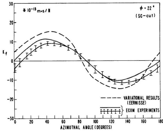
FIG. 4.21: Coefficient force-fréquence K_f(\psi) pour le résonateur standard [72].
