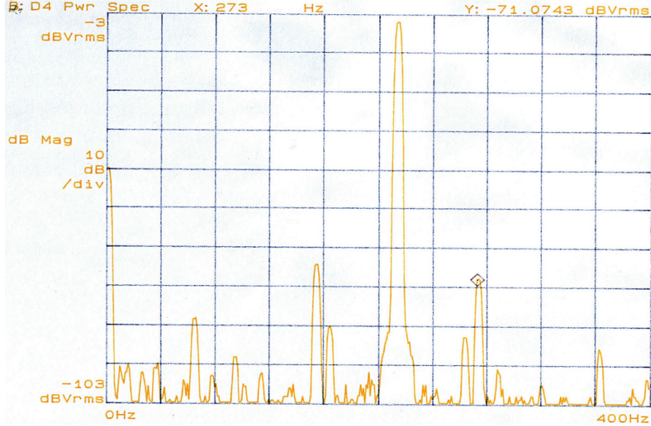
FIG. 2.5: Spectre d'un résonateur soumis à une vibration sinusoïdale.
