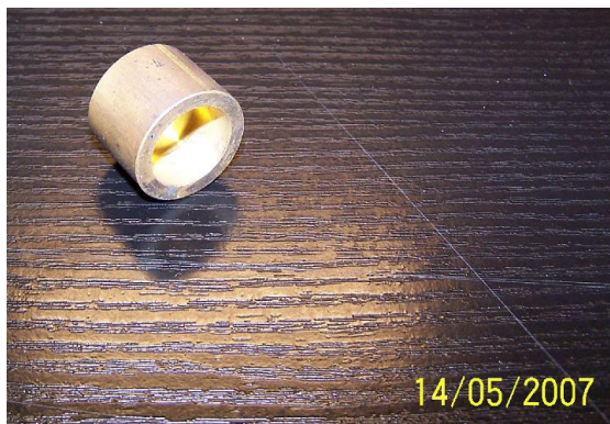
FIG. C.9: Le four placé sur le résonateur dans l'oscillateur OP22-M.
