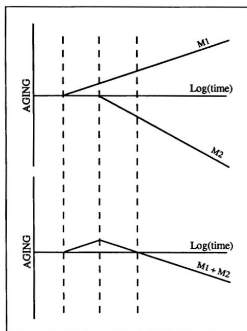
FIG. 3.14: Dépendance à deux mécanismes logarithmiques du vieillissement changeant de direction. [21].
