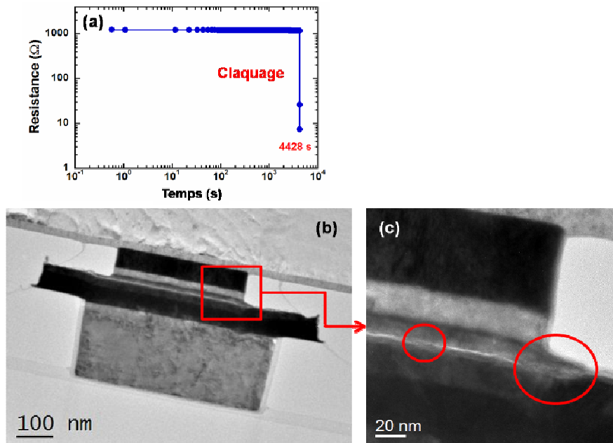
Figure A-2-28 : (a) Caractéristique I(V) mesurée sur une jonction magnétique présentant un claquage diélectrique après 4 428 s sous une sollicitation statique de 0,8 V. (b) et (c) Sections transverses MET de cette jonction après claquage (observations à deux grossissements différents).
