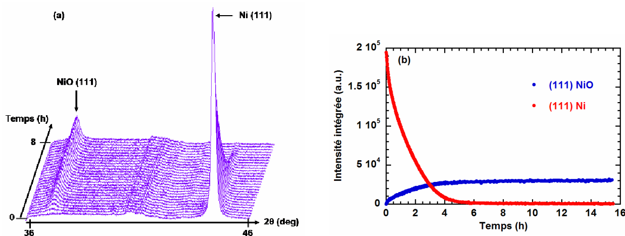
Figure B-2-14 : (a) Variations concomitantes des réflexions (111) de Ni et NiO en fonction du temps d'oxydation à 400^\circ\text{C} . L'évolution de l'intensité intégrée est présentée sur la figure (b).
