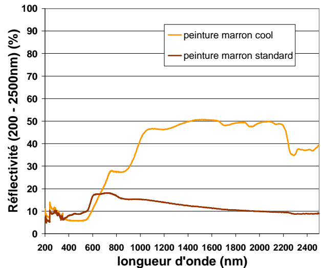
Figure 30 : comparaison de la réflectivité spectrale à une source de 1000W/m 2 d'une peinture standard et d'une teinte équivalente préparée COOL pour des teintes verte et marron
