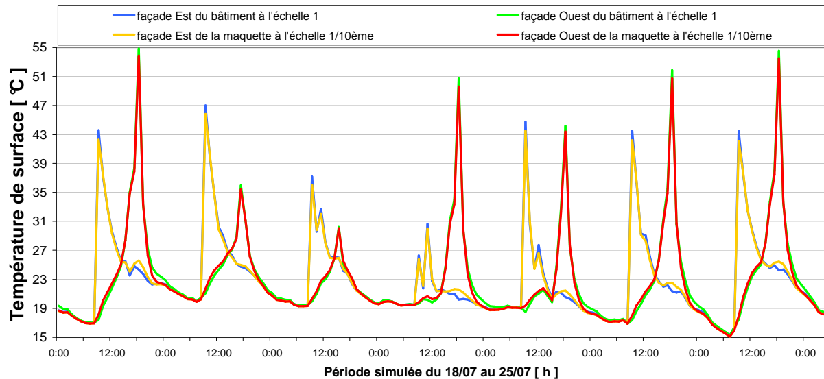
Figure 60 : Températures de façades pour un bâtiment réel et la maquette à l'échelle 1/10 ème simulées avec TRNSYS
