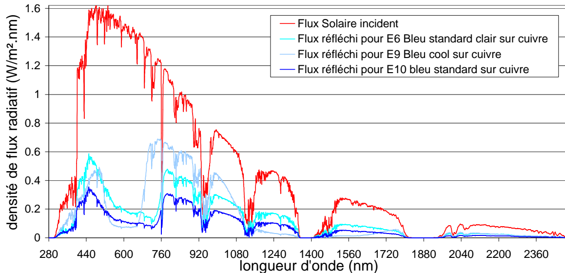
Figure 29: comparaison de la réflectivité des peintures Bleues standard, standard éclairci avec du blanc et COOL
