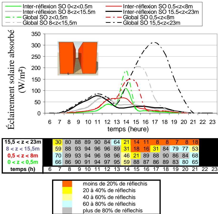
Figure 121 : Répartition modélisée de l'éclairement solaire absorbée lors de la première incidence et après inter-réflexions pour la rue orange standard au 16 juillet par ciel clair
