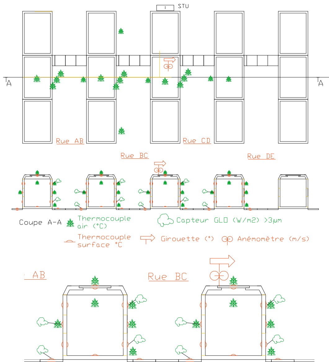
Figure 76 : Schéma des emplacements des thermocouples, capteurs de flux GLO et de l'anémomètre sonore
