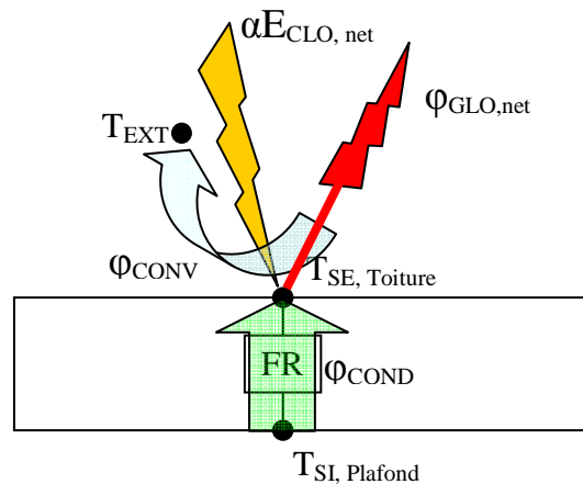
Figure 108: Bilan thermique à la surface d'une toiture
