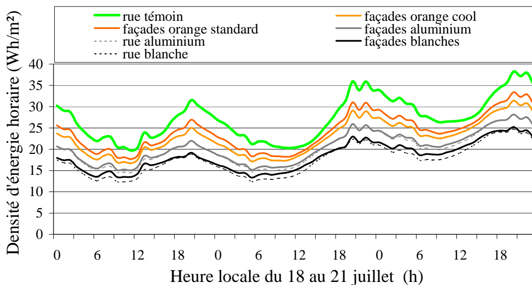
Figure 126 : Comparaison de la demande énergétique d'été pour l'ensemble des locaux situés sur la façade SO du 18/07/2001 au 20/07/2001 en fonction des stratégies
