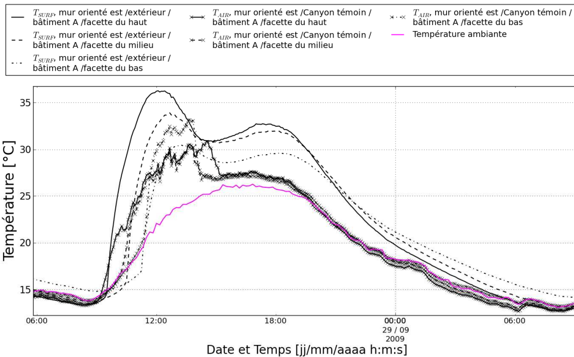
Figure 99 : Comparaison de l'évolution des températures d'air dans le canyon témoin par rapport à leur température de surface adjacente
