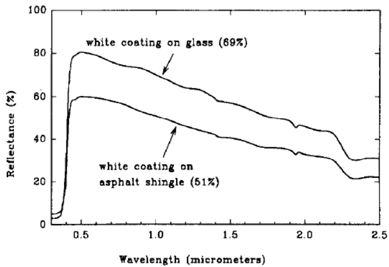
Figure 22 : Réflectivité spectrale de la même peinture appliquée sur un substrat de verre lisse et sur un bardeau d'asphalte rugueux (granules d'environ 1 mm de diamètre).
