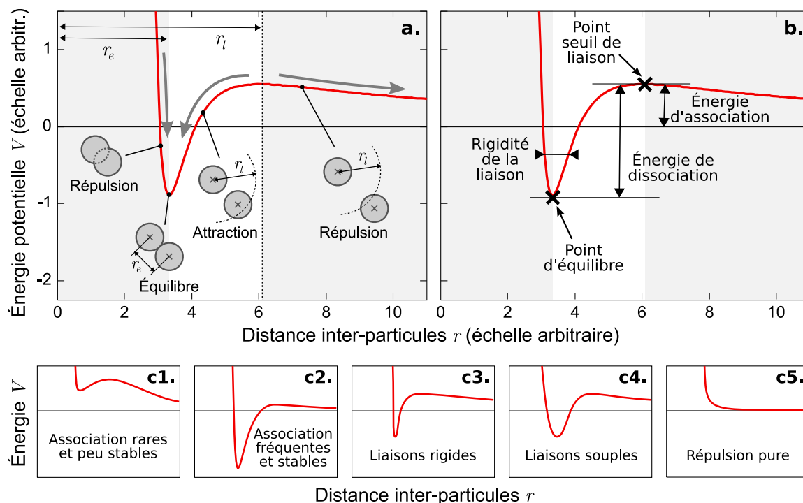
Fig. 11.3: Interprétation et pouvoir d'expression d'un potentiel d'interaction de paire. Le profil de l'énergie potentielle V représentant l'interaction entre deux particules en fonction de leur distance r permet de rendre compte de nombreux aspects physiques de leur association/dissociation. Le principe illustré ici s'applique aussi bien à l'interaction entre atomes (comme dans la figure 11.2), qu'à l'interaction entre grains ou entre macromolécules entières (cf section 1.3), le potentiel ayant par ailleurs souvent un profil qualitativement similaire dans ces différents cas. (a) La force qu'exercent les deux particules l'une sur l'autre est déterminée par la dérivée de l'énergie potentielle V par rapport à r . Le potentiel fortement décroissant pour r < r_e décrit donc ici une répulsion importante des deux particules (correspondant à la force de contact), la partie croissante pour r_e \leq r < r_l décrit une force d'attraction et la partie décroissante pour r_l \leq r , à nouveau une répulsion. Ainsi, dès lors que la distance inter-particules r est inférieure à r_l , les deux particules tendent spontanément vers l'équilibre de la liaison r = r_e où le potentiel admet une tangente horizontale convexe. (b) Non seulement le point d'équilibre et le point seuil de liaison définissent les distances r_e et r_l , mais ils déterminent également l'affinité des deux particules. La hauteur de la barrière de potentiel décrit l'énergie à fournir pour leur association (depuis une distance théoriquement infinie où le potentiel est nul) et la profondeur du puits correspond à l'énergie à fournir pour leur dissociation, permettant alors de représenter simplement différentes affinités (c1,c2). De plus, la largeur du puits de potentiel détermine à quel point deux particules associées peuvent facilement s'écarter de leur distance d'équilibre r_e , permettant alors de décrire des liaisons plus ou moins souples (c3,c4). Enfin, certaines particules peuvent n'interagir que par une simple exclusion stérique, auquel cas le potentiel reste décroissant et ne représente qu'une force de contact (c5).
