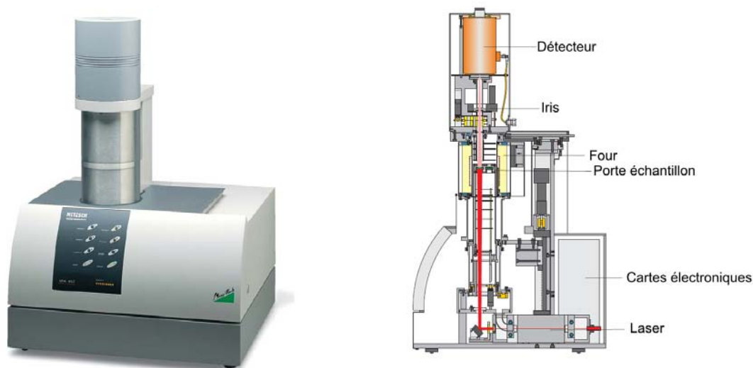
FIGURE 16 – Photographie (à gauche) et schéma (à droite) du diffusivimètre « LFA 457 ».
