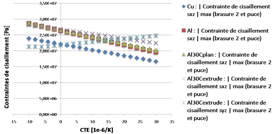
FIGURE 1.24 – Valeurs absolues des maxima de contrainte de cisaillement sxy et sxz , dans la brasure 2 et le drain, en fonction du coefficient d’expansion thermique des différents matériaux utilisés pour le drain thermique.
