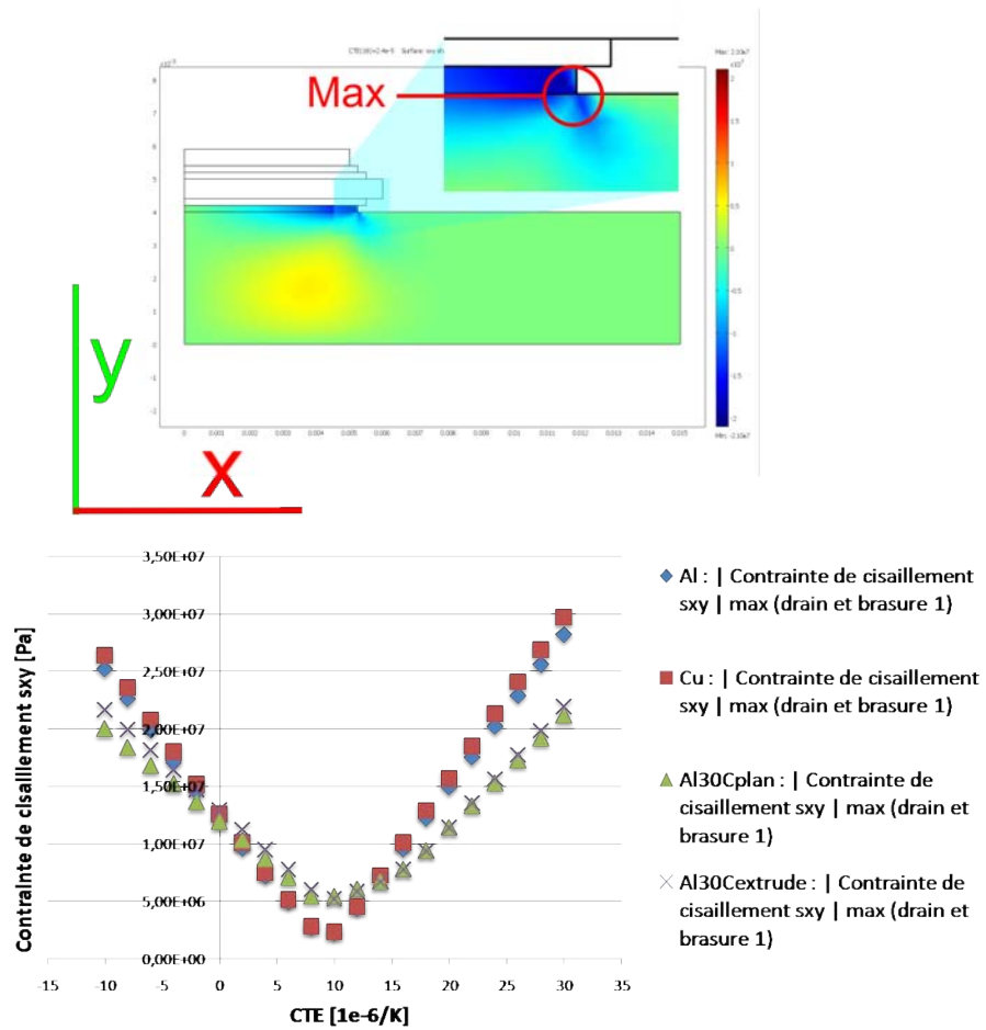
FIGURE 1.8 – Haut : illustration de la position du maximum de contraintes de cisaillement \sigma_{xy} dans la semelle et la brasure 1. Bas : valeurs absolues des maxima de contrainte de cisaillement \sigma_{xy} , dans la semelle et la brasure 1, en fonction du coefficient d’expansion thermique des différents matériaux utilisés pour la semelle.
