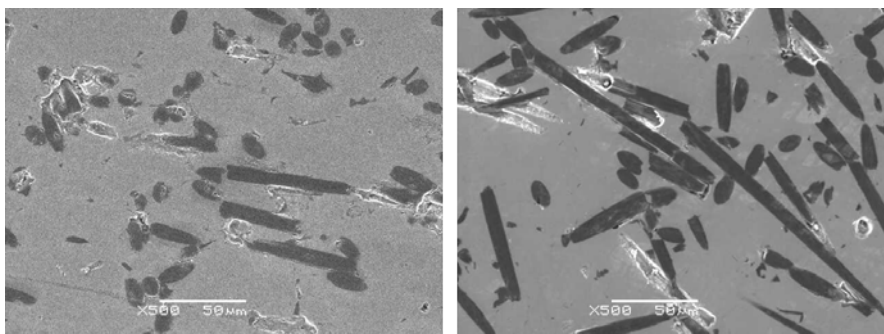
FIGURE 2.21 – Micrographies électroniques d'échantillons Al F3731-30% vol CN80C frittés à 600 °C, 20 minutes par induction (gauche) et par SPS (droite).
