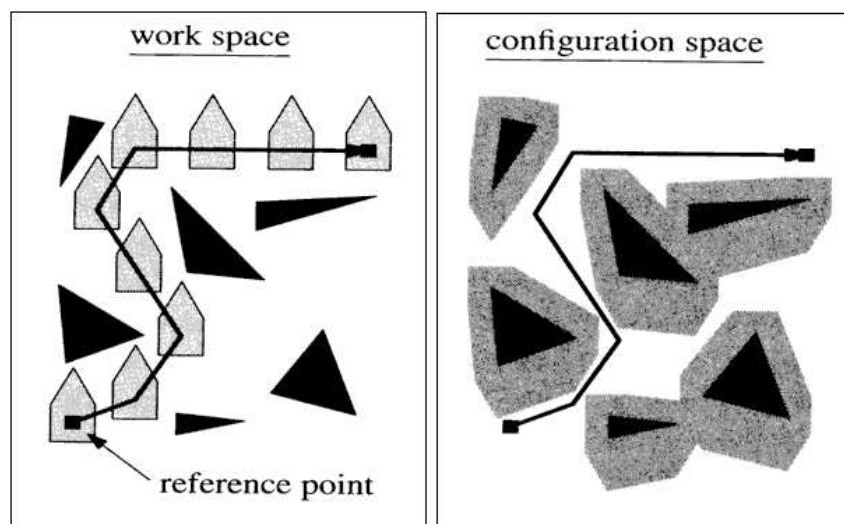
FIG. 2.3 – De [Esteves Jaramillo 2007]. Passage d'un espace de travail usuel (à gauche), vers l'espace des configurations correspondant (à droite).
