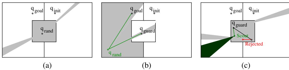
FIG. 2.11 – Illustration de la création des trois différents types de nœuds : (a) Un nœud gardien ( q_{rand} , au milieu), (b) Un nœud connecteur ( q_{rand} , en vert à gauche) et (c) Un nœud éclaircur (en vert au centre). Le nœud rouge est plus proche de la racine que son nœud parent, il est donc rejeté.
