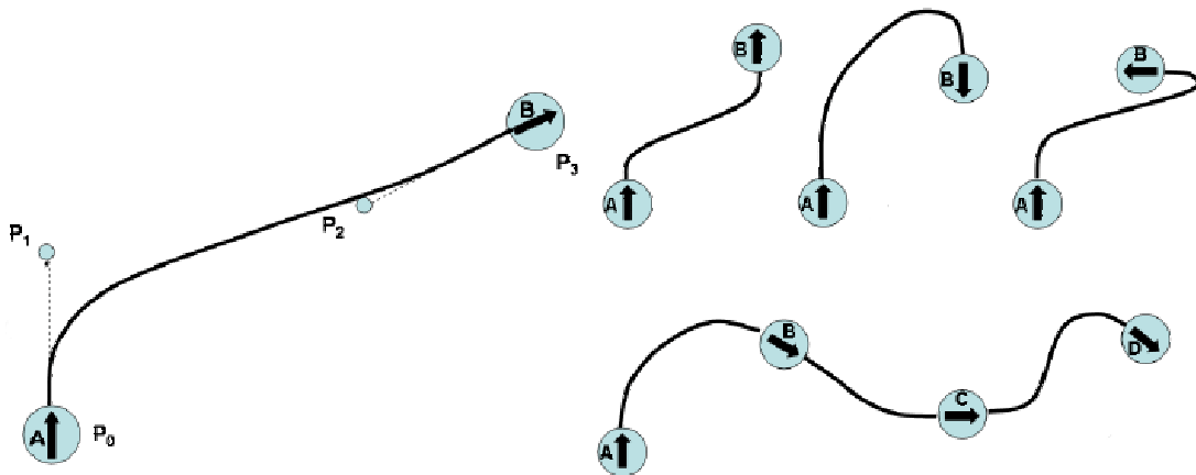
FIG. 4.2 – De [Pettré 2003]. Quelques exemples de chemins locaux construits avec des courbes de Bézier. En bas à droite, un exemple de chemin global composé de plusieurs chemins locaux de Bézier.
