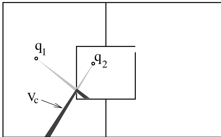
FIG. 2.9 – Un exemple de la difficulté de créer un nœud de connexion avec la méthode Visibility PRM. Un nœud de connexion ne peut être créé que si un échantillon est tiré dans la région V_C , région de visibilité commune de q_1 et q_2 . La probabilité d'avoir une configuration échantillonnée dans la région V_C (en gris foncé) est faible.
