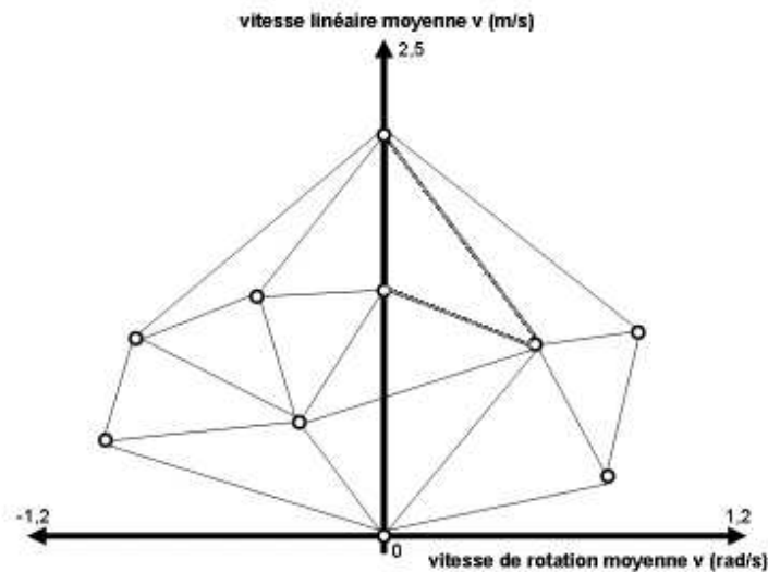
FIG. 4.3 – De [Pettré 2003]. Représentation de l'espace (v, \omega) . Chaque point blanc représente une capture de mouvement, caractérisée par sa vitesse linéaire et sa vitesse angulaire. L'ensemble de mouvements qui peuvent être générés à partir de ces captures se situe à l'intérieur du polygone convexe formé par ces points.
