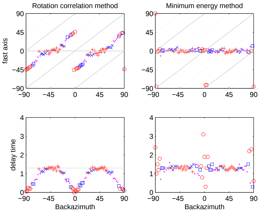
Figure A: Test synthétique à \text{SNR}_R = 15 pour la technique de Rotation-Corrélation (RC, gauche) et la technique minimum d'énergie (SC, droite). Les panneaux supérieurs montrent les haches rapides résultantes à différents backazimuths, expositions inférieures de panneaux que résulter retardent des évaluations de temps. Les valeurs d'entrée ( \Phi_{\text{in}} = 0^\circ et dt_{\text{in}} = 1.3\text{sec} ) sont indiquées par les traits horizontaux. La technique de SC rapporte des évaluations stables pour un éventail de backazimuths. Pour \text{SNR}_R inférieur et/ou plus petit retarder les périodes (voir le supplément électronique) que la RC-technique diffère encore plus des valeurs d'entrée. Bon Nulls détecté automatiquement sont marqué comme cercles, proche Nulls comme carres. De bons résultats sont marqués comme plus des signes, et des résultats proches comme croix. Des résultats pauvres sont indiqués comme points.
